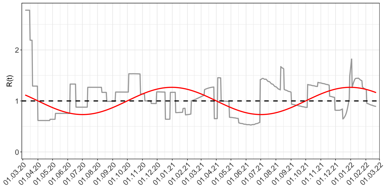
Abbildung 5: Saisonalitätseffekt auf die Infektiosität von SARS-CoV-2 im Laufe des Jahres (rote Linie) und die von dem Modell abgeschätzten R(t) Werte (graue Linie)
