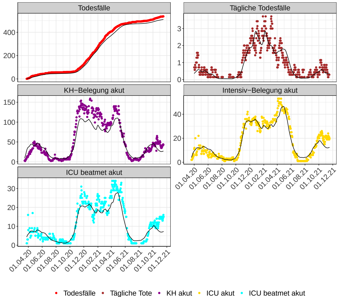
Abbildung 58: Modellbeschreibung der Belegung von KH Betten und Intensivstationen, und Todesfällen in Bremen. Punkte: gemeldete Daten; Linie: Modellbeschreibung. Tägliche Tote und Tägliche KH sind als 7-Tage gleitender Durchschnitt dargestellt
