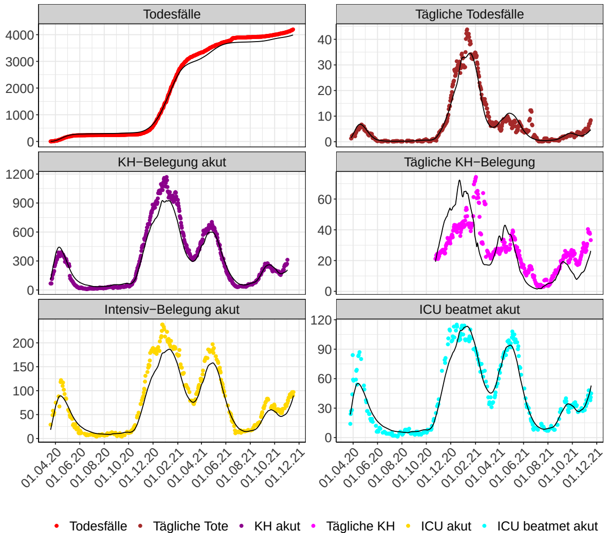
Abbildung 106: Modellbeschreibung der Belegung von KH Betten und Intensivstationen, und Todesfällen in Rheinland-Pfalz. Punkte: gemeldete Daten; Linie: Modellbeschreibung. Tägliche Tote und Tägliche KH sind als 7-Tage gleitender Durchschnitt dargestellt
