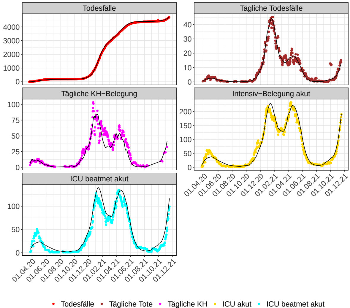
Abbildung 143: Modellbeschreibung der Belegung von KH Betten und Intensivstationen, und Todesfällen in Thüringen. Punkte: gemeldete Daten; Linie: Modellbeschreibung. Tägliche Tote und Tägliche KH sind als 7-Tage gleitender Durchschnitt dargestellt
