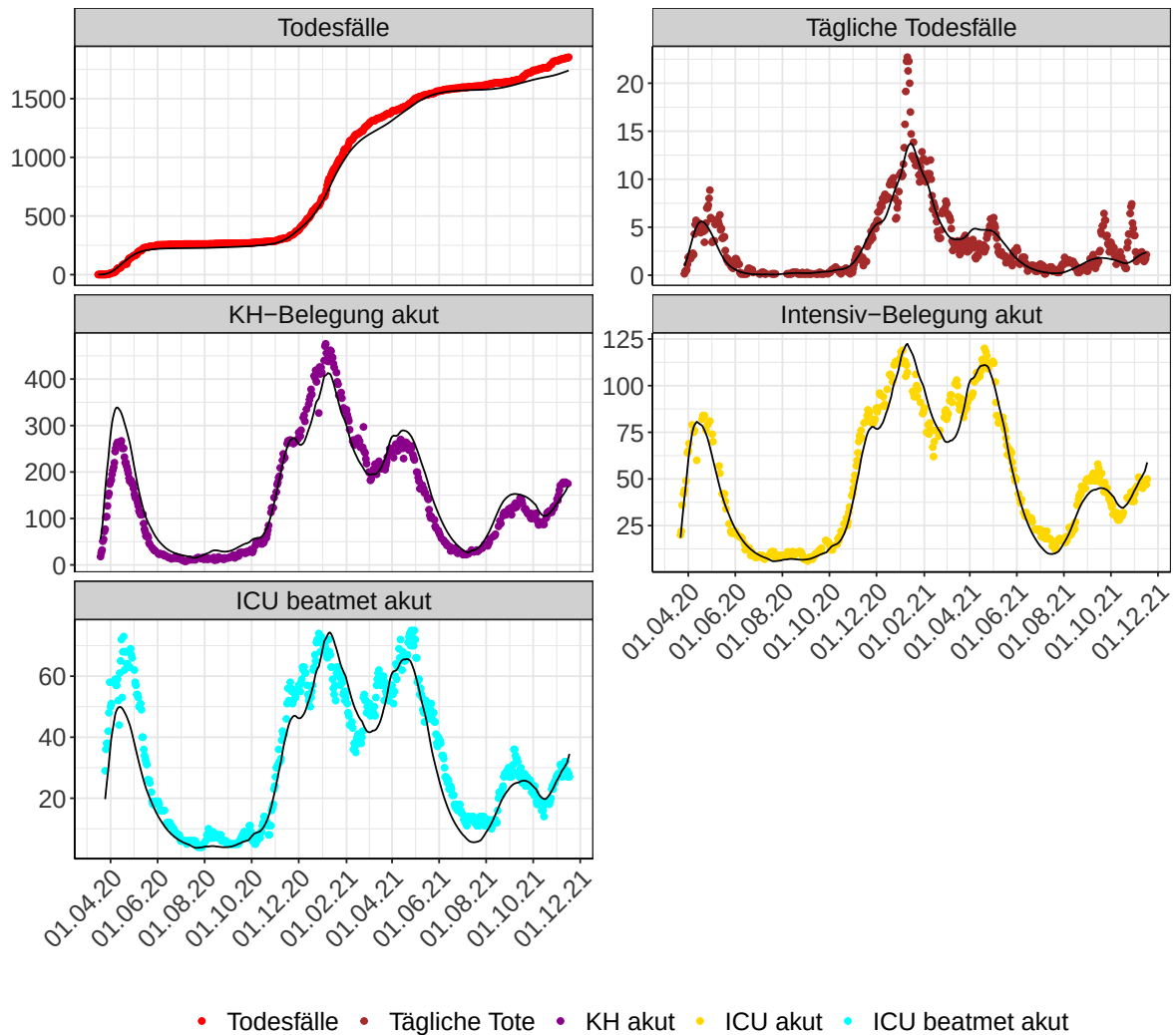
Abbildung 65: Modellbeschreibung der Belegung von KH Betten und Intensivstationen, und Todesfällen in Hamburg. Punkte: gemeldete Daten; Linie: Modellbeschreibung. Tägliche Tote und Tägliche KH sind als 7-Tage gleitender Durchschnitt dargestellt
