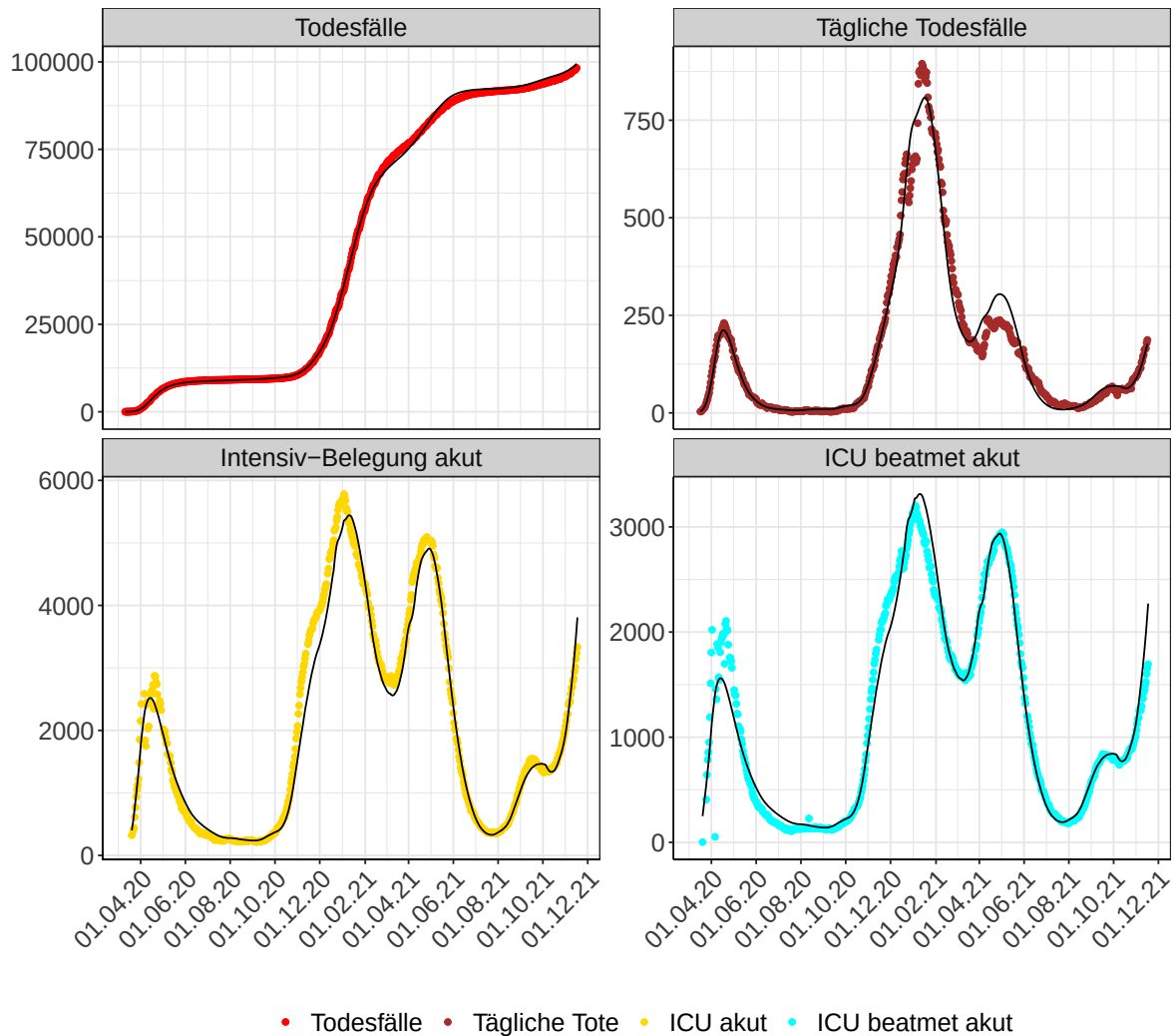
Abbildung 151: Modellbeschreibung der Belegung von KH Betten und Intensivstationen, und Todesfällen in Deutschland. Punkte: gemeldete Daten; Linie: Modellbeschreibung. Tägliche Tote und Tägliche KH sind als 7-Tage gleitender Durchschnitt dargestellt
