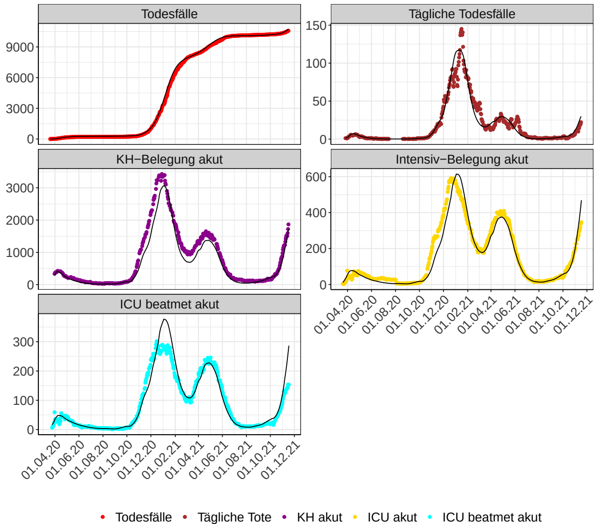
Abbildung 122: Modellbeschreibung der Belegung von KH Betten und Intensivstationen, und Todesfällen in Sachsen. Punkte: gemeldete Daten; Linie: Modellbeschreibung. Tägliche Tote und Tägliche KH sind als 7-Tage gleitender Durchschnitt dargestellt
