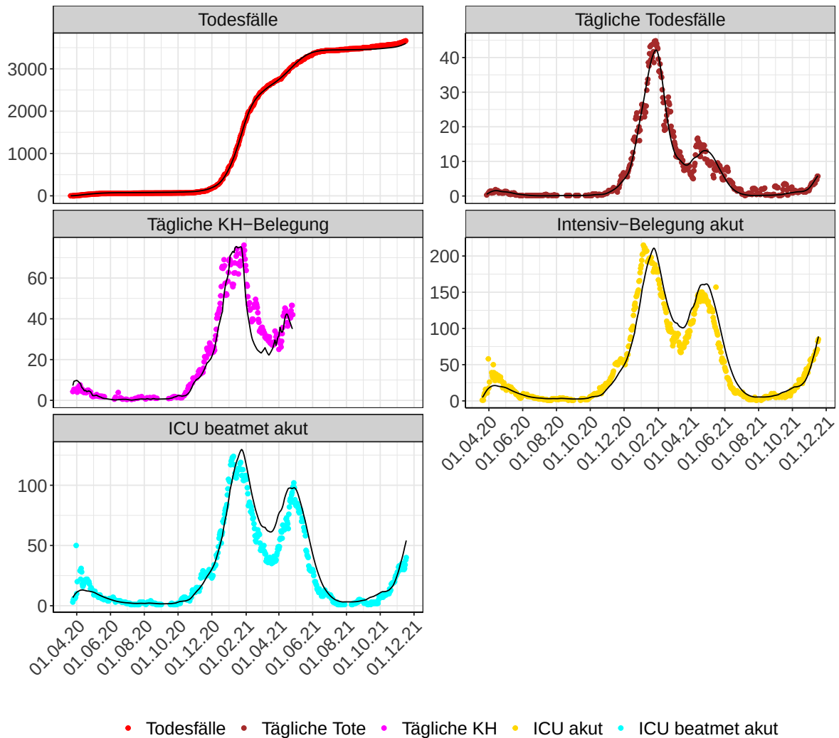
Abbildung 129: Modellbeschreibung der Belegung von KH Betten und Intensivstationen, und Todesfällen in Sachsen-Anhalt. Punkte: gemeldete Daten; Linie: Modellbeschreibung. Tägliche Tote und Tägliche KH sind als 7-Tage gleitender Durchschnitt dargestellt
