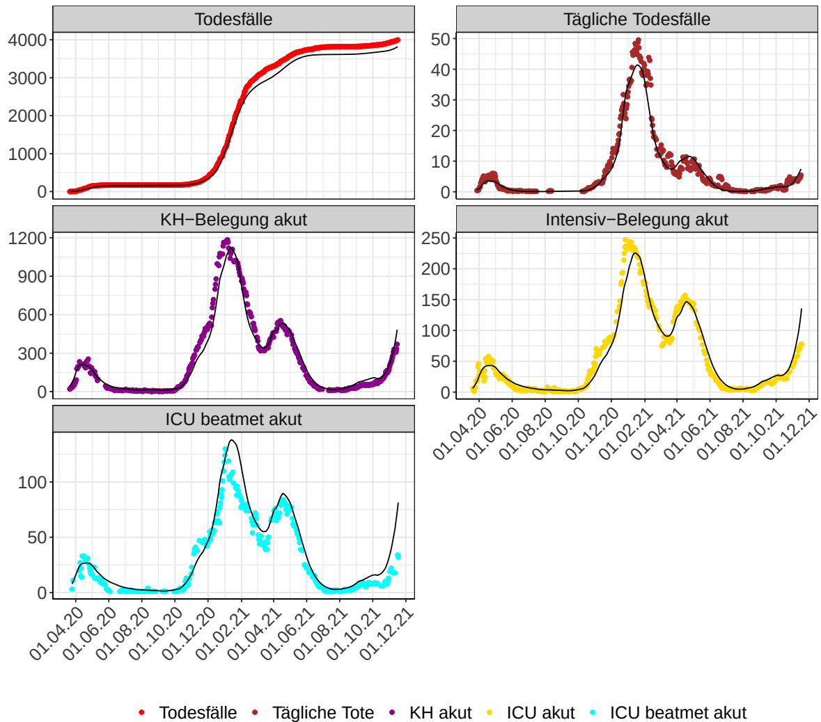
Abbildung 50: Modellbeschreibung der Belegung von KH Betten und Intensivstationen, und Todesfällen in Brandenburg. Punkte: gemeldete Daten; Linie: Modellbeschreibung. Tägliche Tote und Tägliche KH sind als 7-Tage gleitender Durchschnitt dargestellt
