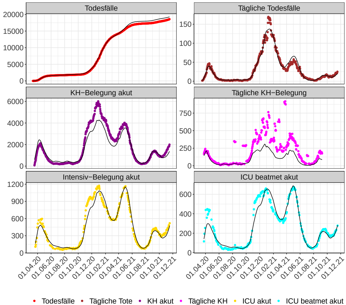
Abbildung 96: Modellbeschreibung der Belegung von KH Betten und Intensivstationen, und Todesfällen in Nordrhein-Westfalen. Punkte: gemeldete Daten; Linie: Modellbeschreibung. Tägliche Tote und Tägliche KH sind als 7-Tage gleitender Durchschnitt dargestellt
