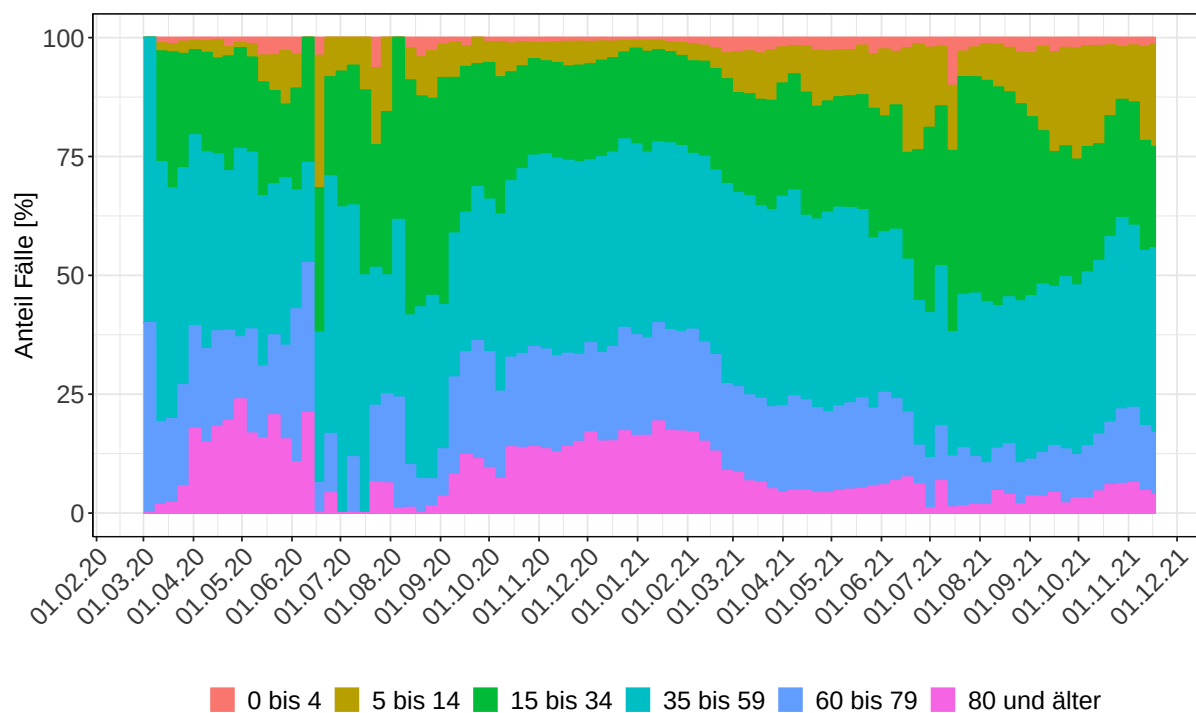
Abbildung 119: Alterverteilung der COVID-19 Fälle über die Zeit in Sachsen. Anteil der Fälle je Altersgruppe zusammengefasst je Woche
