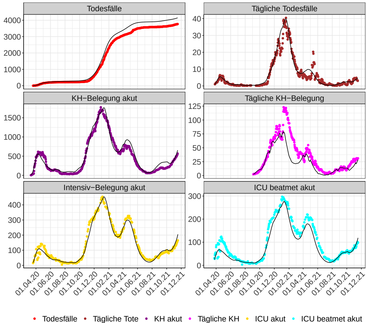
Abbildung 43: Modellbeschreibung der Belegung von KH Betten und Intensivstationen, und Todesfällen in Berlin. Punkte: gemeldete Daten; Linie: Modellbeschreibung. Tägliche Tote und Tägliche KH sind als 7-Tage gleitender Durchschnitt dargestellt
