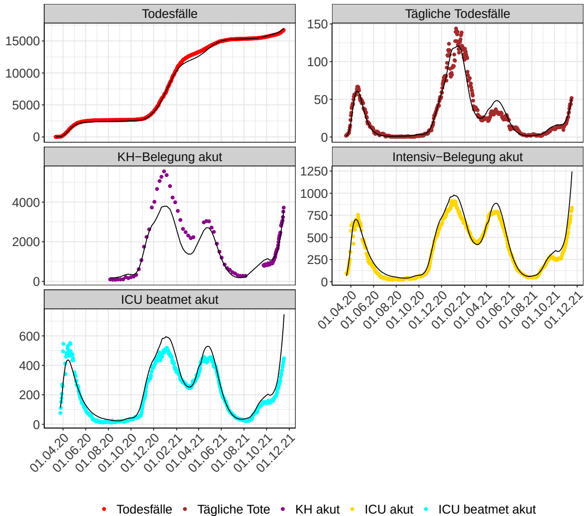
Abbildung 30: Modellbeschreibung der Belegung von KH Betten und Intensivstationen, und Todesfällen in Bayern. Punkte: gemeldete Daten; Linie: Modellbeschreibung. Tägliche Tote und Tägliche KH sind als 7-Tage gleitender Durchschnitt dargestellt
