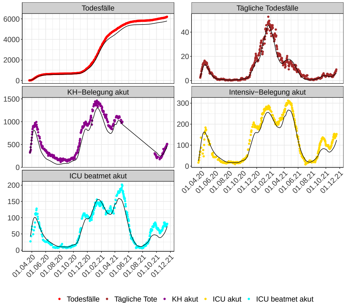
Abbildung 87: Modellbeschreibung der Belegung von KH Betten und Intensivstationen, und Todesfällen in Niedersachsen. Punkte: gemeldete Daten; Linie: Modellbeschreibung. Tägliche Tote und Tägliche KH sind als 7-Tage gleitender Durchschnitt dargestellt
