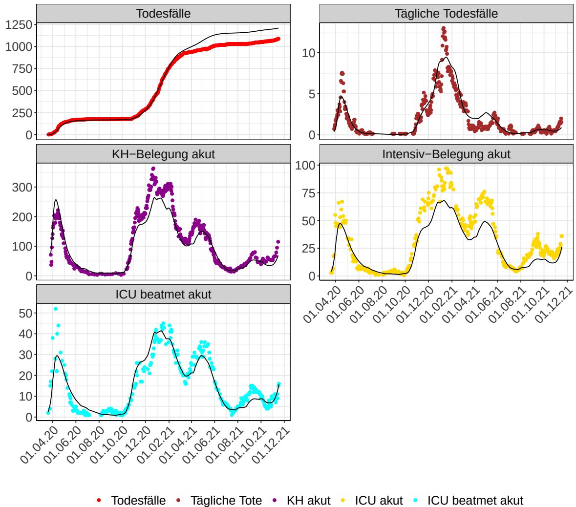
Abbildung 115: Modellbeschreibung der Belegung von KH Betten und Intensivstationen, und Todesfällen in Saarland. Punkte: gemeldete Daten; Linie: Modellbeschreibung. Tägliche Tote und Tägliche KH sind als 7-Tage gleitender Durchschnitt dargestellt
