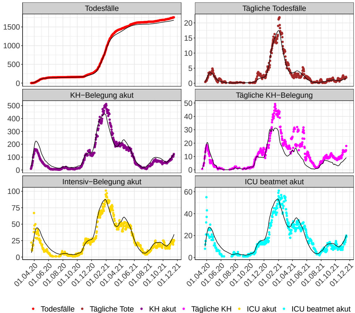
Abbildung 136: Modellbeschreibung der Belegung von KH Betten und Intensivstationen, und Todesfällen in Schleswig-Holstein. Punkte: gemeldete Daten; Linie: Modellbeschreibung. Tägliche Tote und Tägliche KH sind als 7-Tage gleitender Durchschnitt dargestellt
