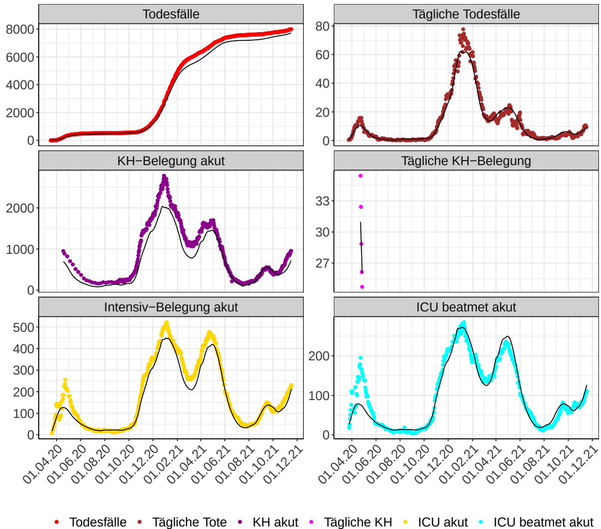
Abbildung 72: Modellbeschreibung der Belegung von KH Betten und Intensivstationen, und Todesfällen in Hessen. Punkte: gemeldete Daten; Linie: Modellbeschreibung. Tägliche Tote und Tägliche KH sind als 7-Tage gleitender Durchschnitt dargestellt
