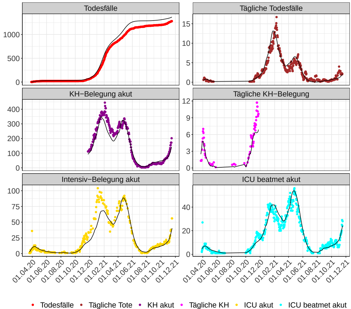
Abbildung 80: Modellbeschreibung der Belegung von KH Betten und Intensivstationen, und Todesfällen in Mecklenburg-Vorpommern. Punkte: gemeldete Daten; Linie: Modellbeschreibung. Tägliche Tote und Tägliche KH sind als 7-Tage gleitender Durchschnitt dargestellt
