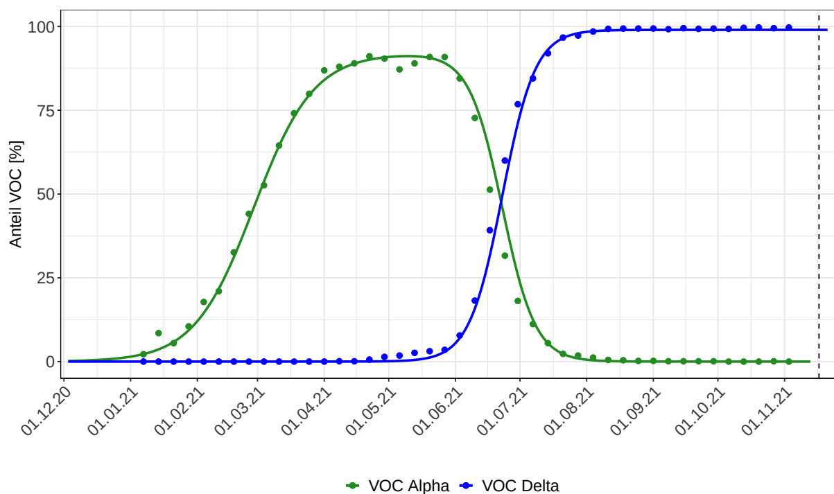
Abbildung 2: Anteile Variants of Concern B.1.1.7 (Alpha) und B.1.617.2 (Delta) in Deutschland. Punkte stellen die Daten aus der Gesamtgenomsequenzierung dar. Die gestrichelte Linie markiert den heutigen Tag.
