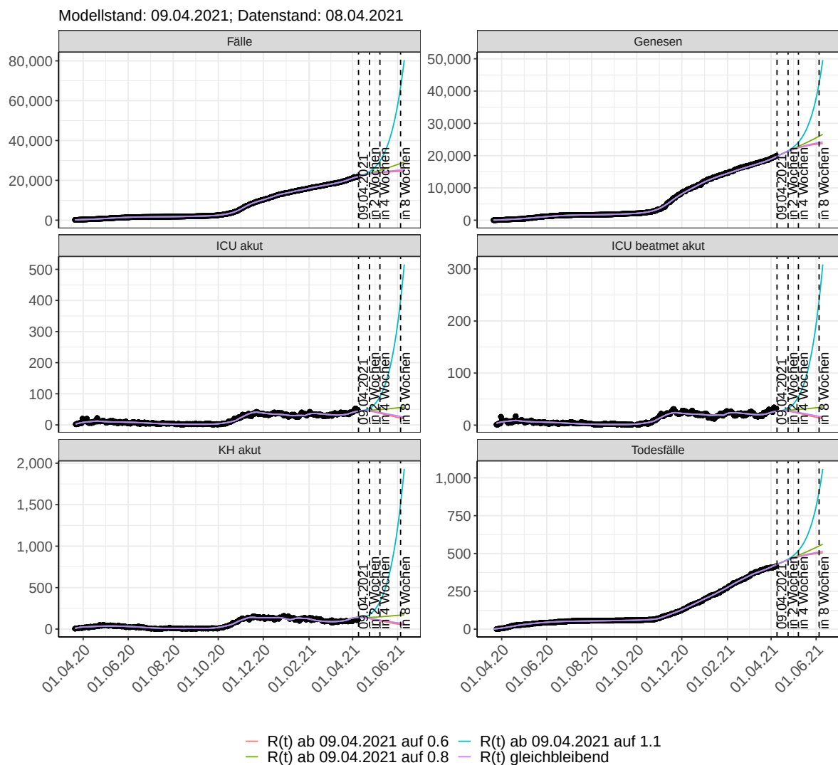
Abbildung 80: Lineare Darstellung der Modellvorhersage (Fallzahlen, Genesen, ICU Beatmet, ICU Betten, KH Betten, Todesfälle) für Bremen unter Annahme verschiedener Szenarien ab dem 09.04.2021. Punkte: gemeldete Fallzahlen; Linien: Modellvorhersage.
