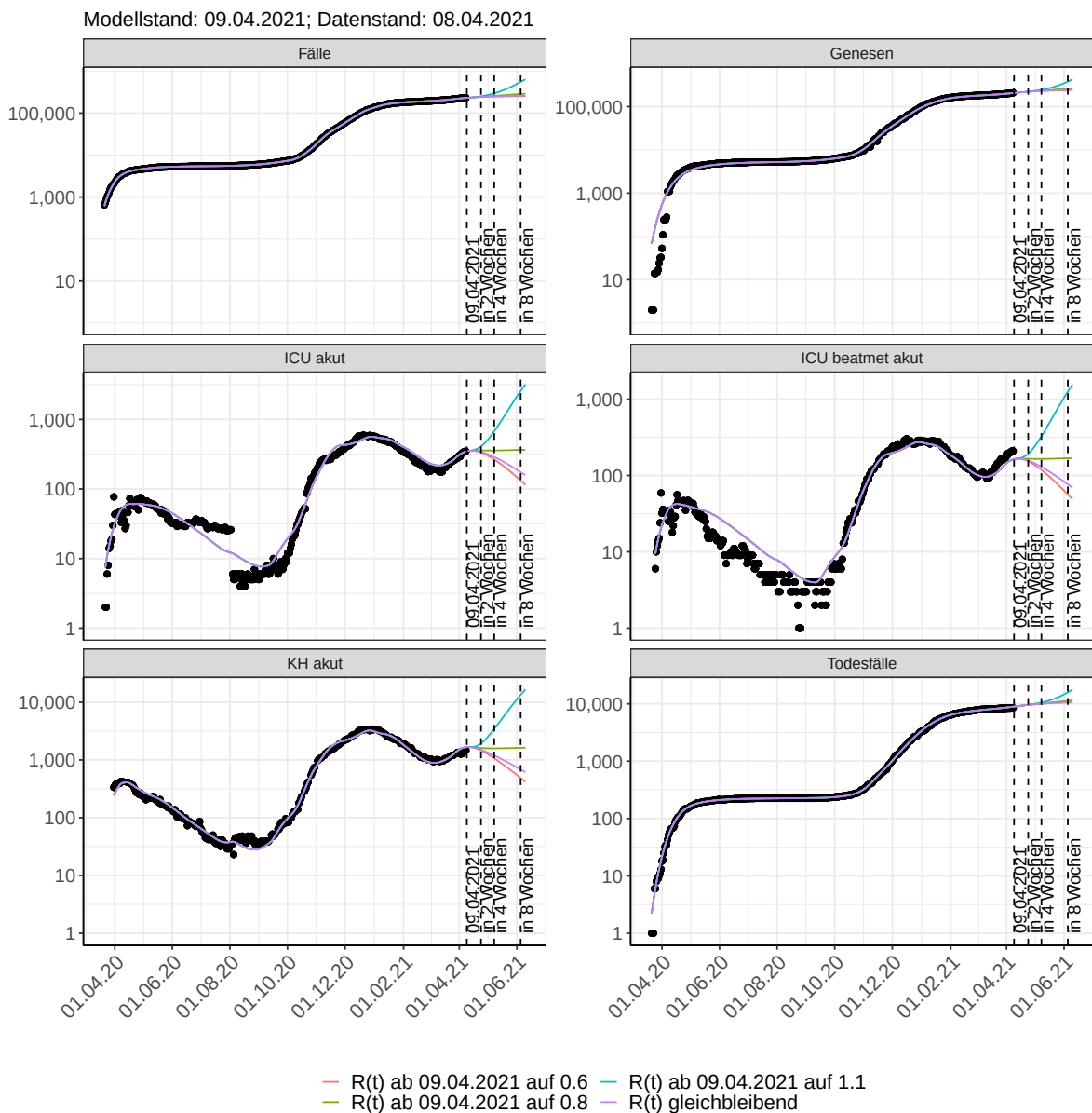
Abbildung 181: Halblogarithmische Darstellung der Modellvorhersage (Fallzahlen, Genesen, ICU Beatmet, ICU Betten, KH Betten, Todesfälle) für Sachsen unter Annahme verschiedener Szenarien nach dem 09.04.2021. Punkte: gemeldete Fallzahlen; Linien: Modellvorhersage.
