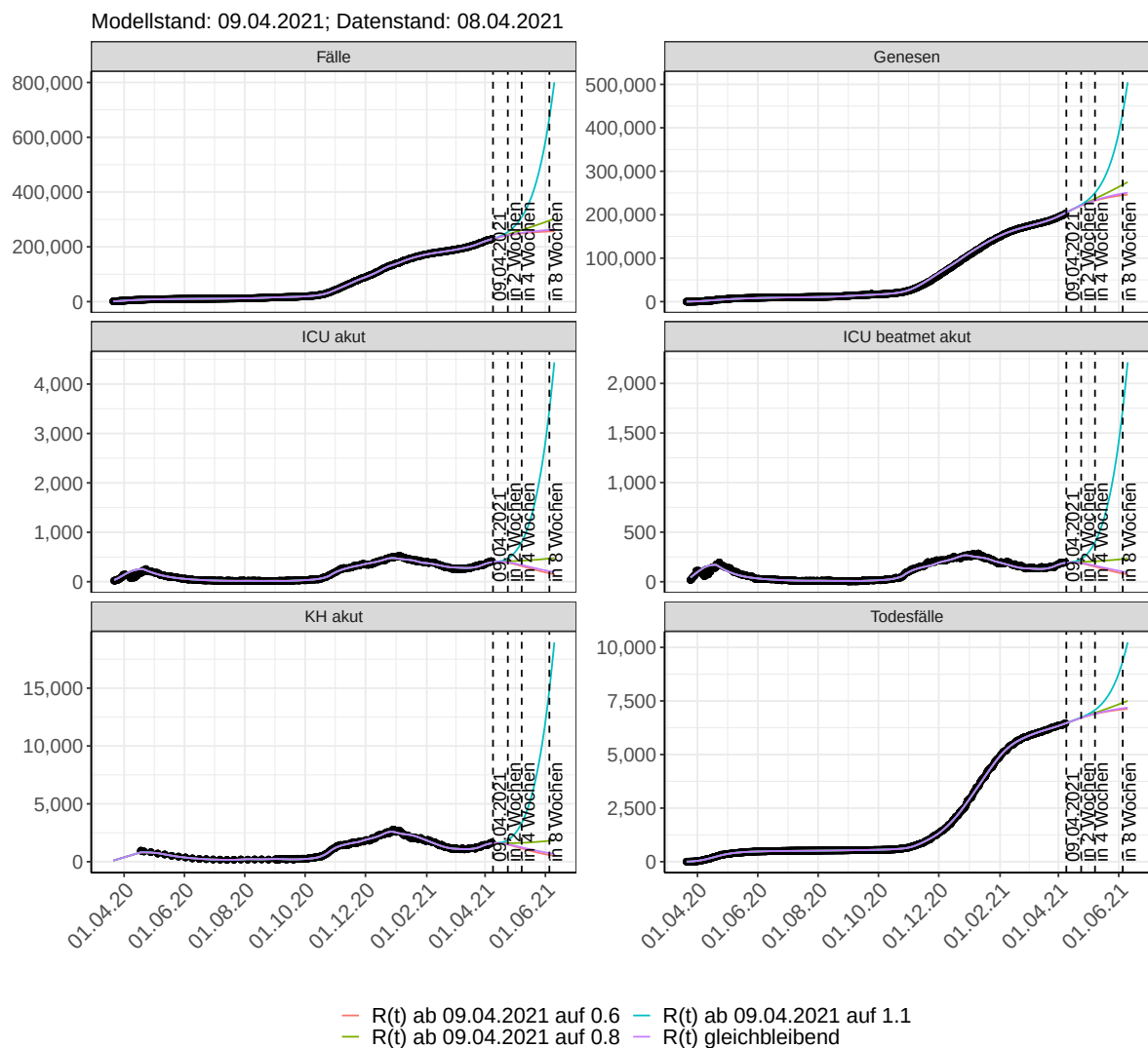
Abbildung 102: Lineare Darstellung der Modellvorhersage (Fallzahlen, Genesen, ICU Beatmet, ICU Betten, KH Betten, Todesfälle) für Hessen unter Annahme verschiedener Szenarien ab dem 09.04.2021. Punkte: gemeldete Fallzahlen; Linien: Modellvorhersage.
