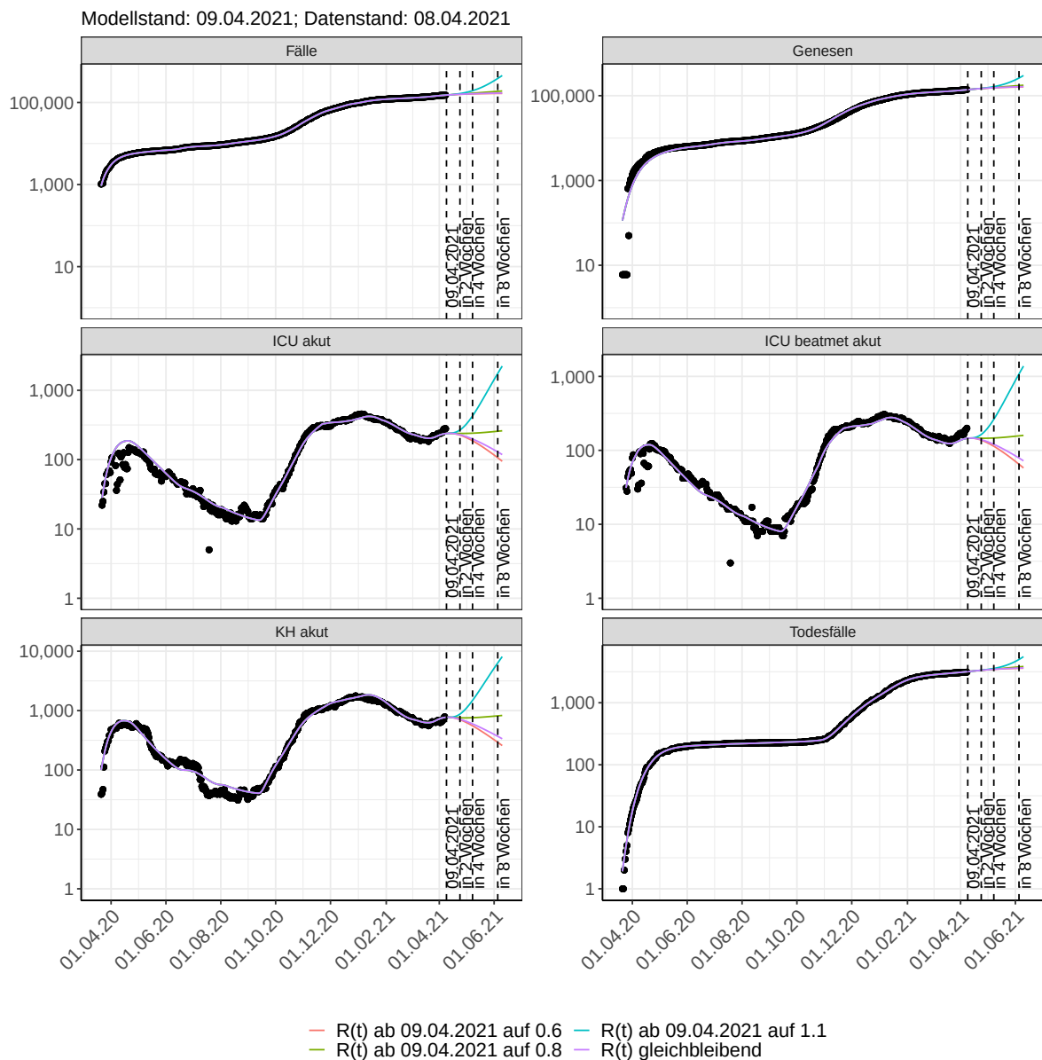
Abbildung 59: Halblogarithmische Darstellung der Modellvorhersage (Fallzahlen, Genesen, ICU Beatmet, ICU Betten, KH Betten, Todesfälle) für Berlin unter Annahme verschiedener Szenarien nach dem 09.04.2021. Punkte: gemeldete Fallzahlen; Linien: Modellvorhersage.
