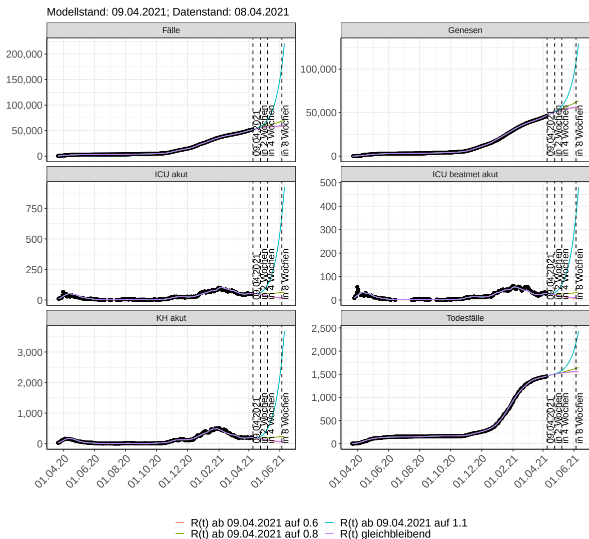
Abbildung 202: Lineare Darstellung der Modellvorhersage (Fallzahlen, Genesen, ICU Beatmet, ICU Betten, KH Betten, Todesfälle) für Schleswig-Holstein unter Annahme verschiedener Szenarien ab dem 09.04.2021. Punkte: gemeldete Fallzahlen; Linien: Modellvorhersage.
