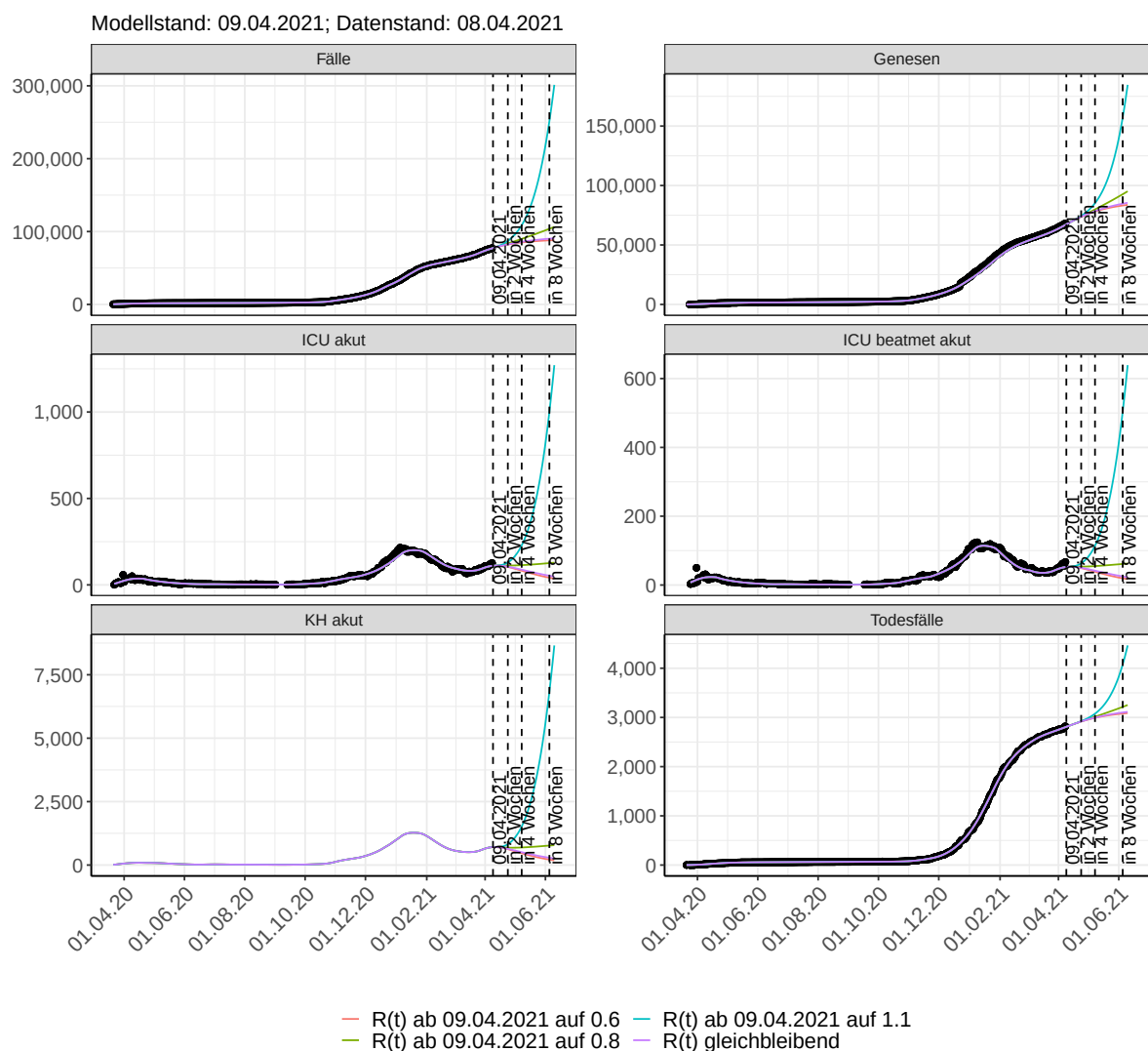
Abbildung 191: Lineare Darstellung der Modellvorhersage (Fallzahlen, Genesen, ICU Beatmet, ICU Betten, KH Betten, Todesfälle) für Sachsen-Anhalt unter Annahme verschiedener Szenarien ab dem 09.04.2021. Punkte: gemeldete Fallzahlen; Linien: Modellvorhersage.
