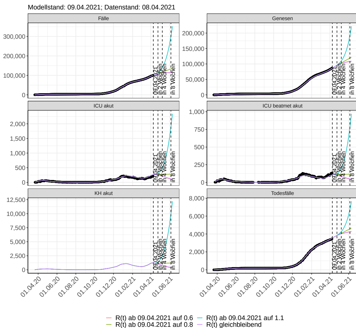
Abbildung 213: Lineare Darstellung der Modellvorhersage (Fallzahlen, Genesen, ICU Beatmet, ICU Betten, KH Betten, Todesfälle) für Thüringen unter Annahme verschiedener Szenarien ab dem 09.04.2021. Punkte: gemeldete Fallzahlen; Linien: Modellvorhersage.
