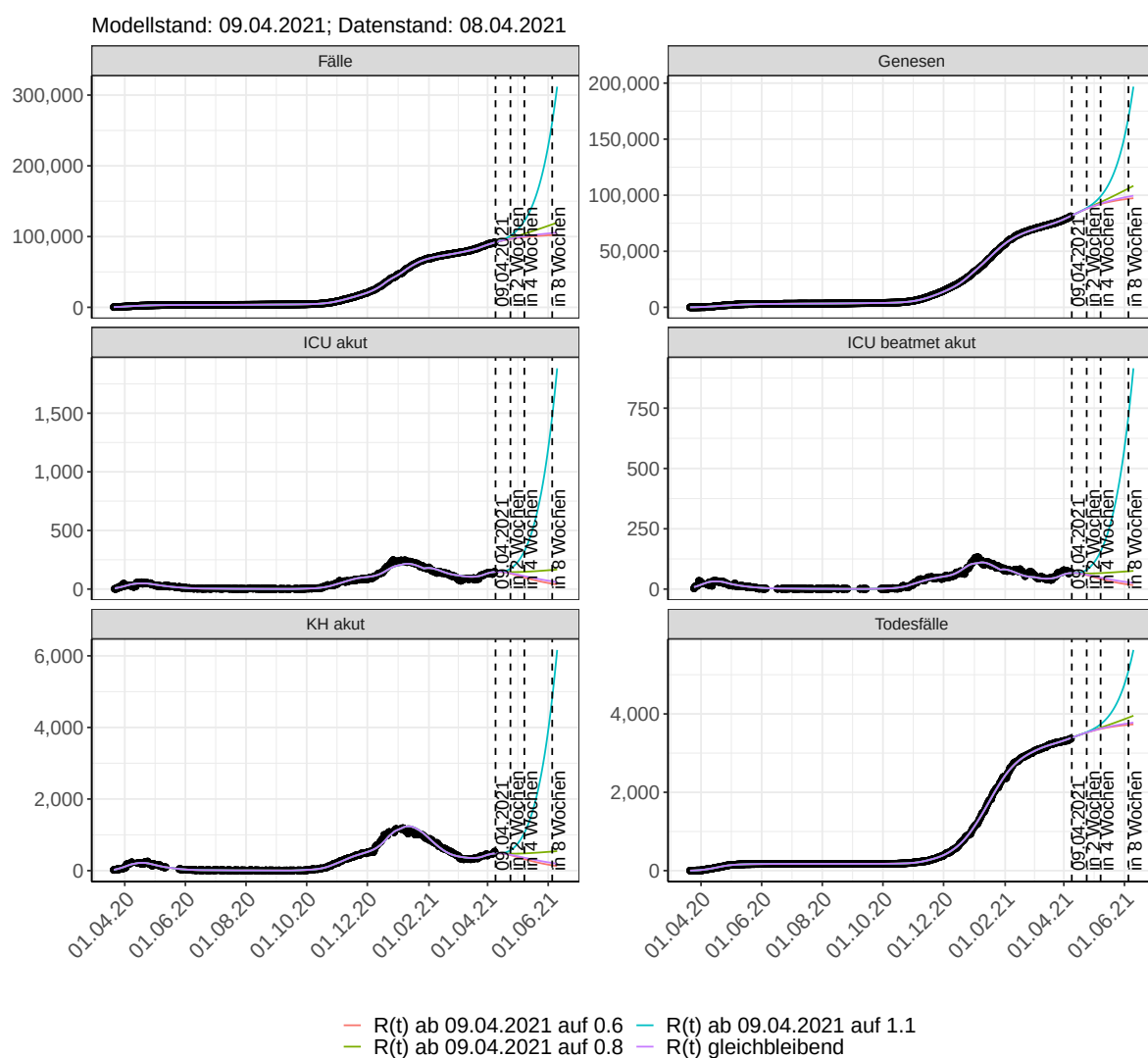
Abbildung 69: Lineare Darstellung der Modellvorhersage (Fallzahlen, Genesen, ICU Beatmet, ICU Betten, KH Betten, Todesfälle) für Brandenburg unter Annahme verschiedener Szenarien ab dem 09.04.2021. Punkte: gemeldete Fallzahlen; Linien: Modellvorhersage.
