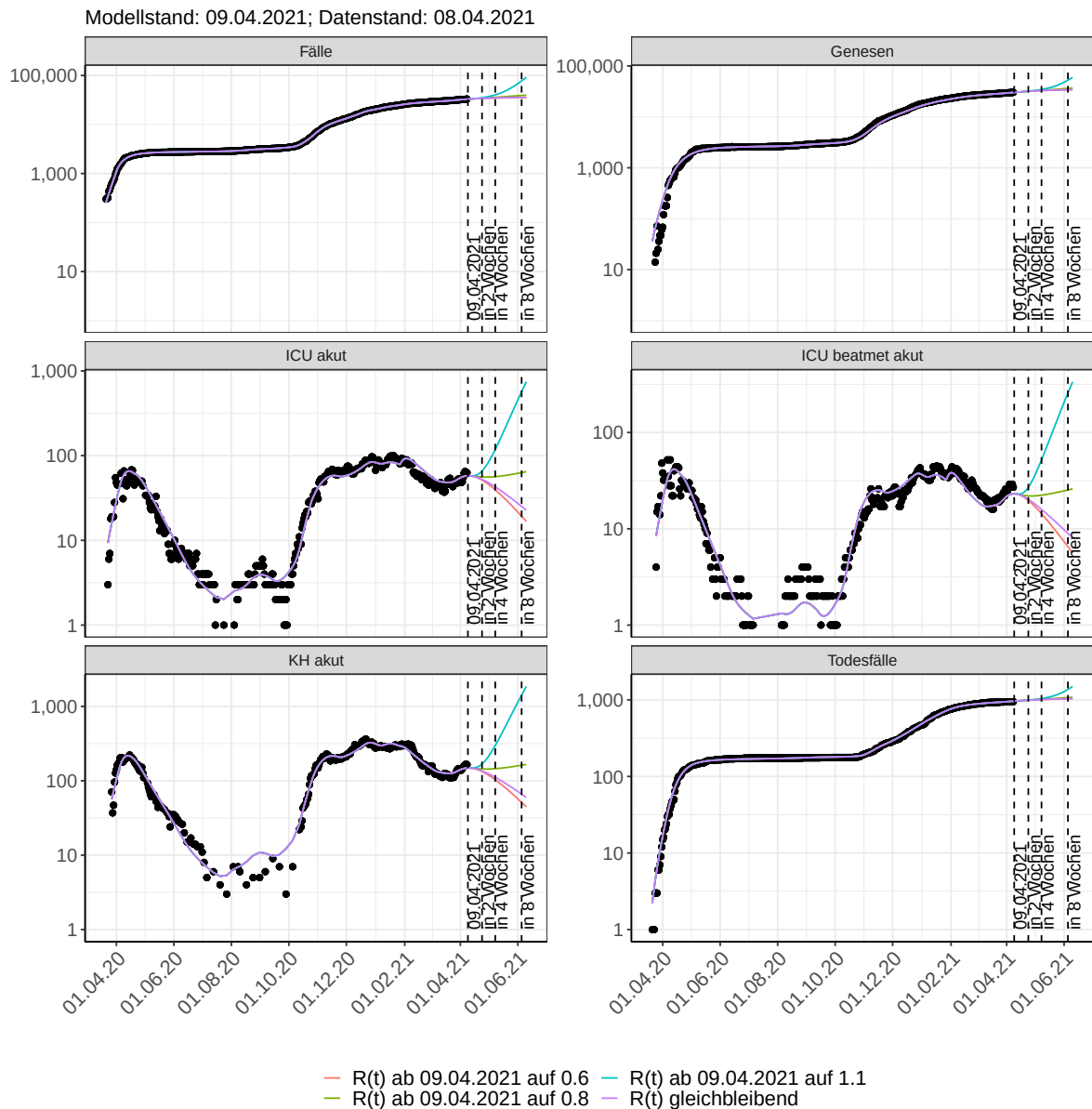
Abbildung 170: Halblogarithmische Darstellung der Modellvorhersage (Fallzahlen, Genesen, ICU Beatmet, ICU Betten, KH Betten, Todesfälle) für Saarland unter Annahme verschiedener Szenarien nach dem 09.04.2021. Punkte: gemeldete Fallzahlen; Linien: Modellvorhersage.
