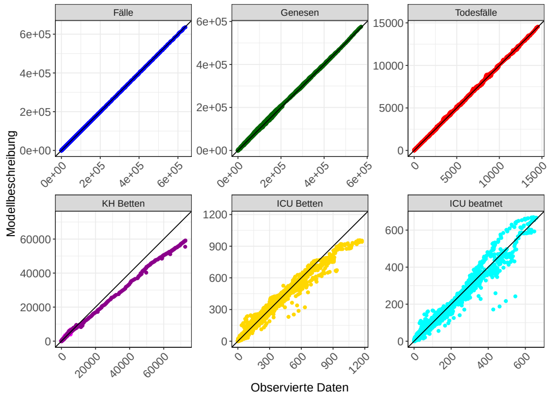
Abbildung 8: Deutschland - Güte der Modellanpassung Goodness-of-fit: gemeldete Daten vs. Modellbeschreibung
