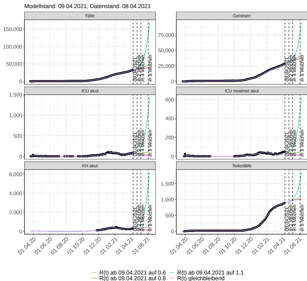
Abbildung 115: Lineare Darstellung der Modellvorhersage (Fallzahlen, Genesen, ICU Beatmet, ICU Betten, KH Betten, Todesfälle) für Mecklenburg-Vorpommern unter Annahme verschiedener Szenarien ab dem 09.04.2021. Punkte: gemeldete Fallzahlen; Linien: Modellvorhersage.
