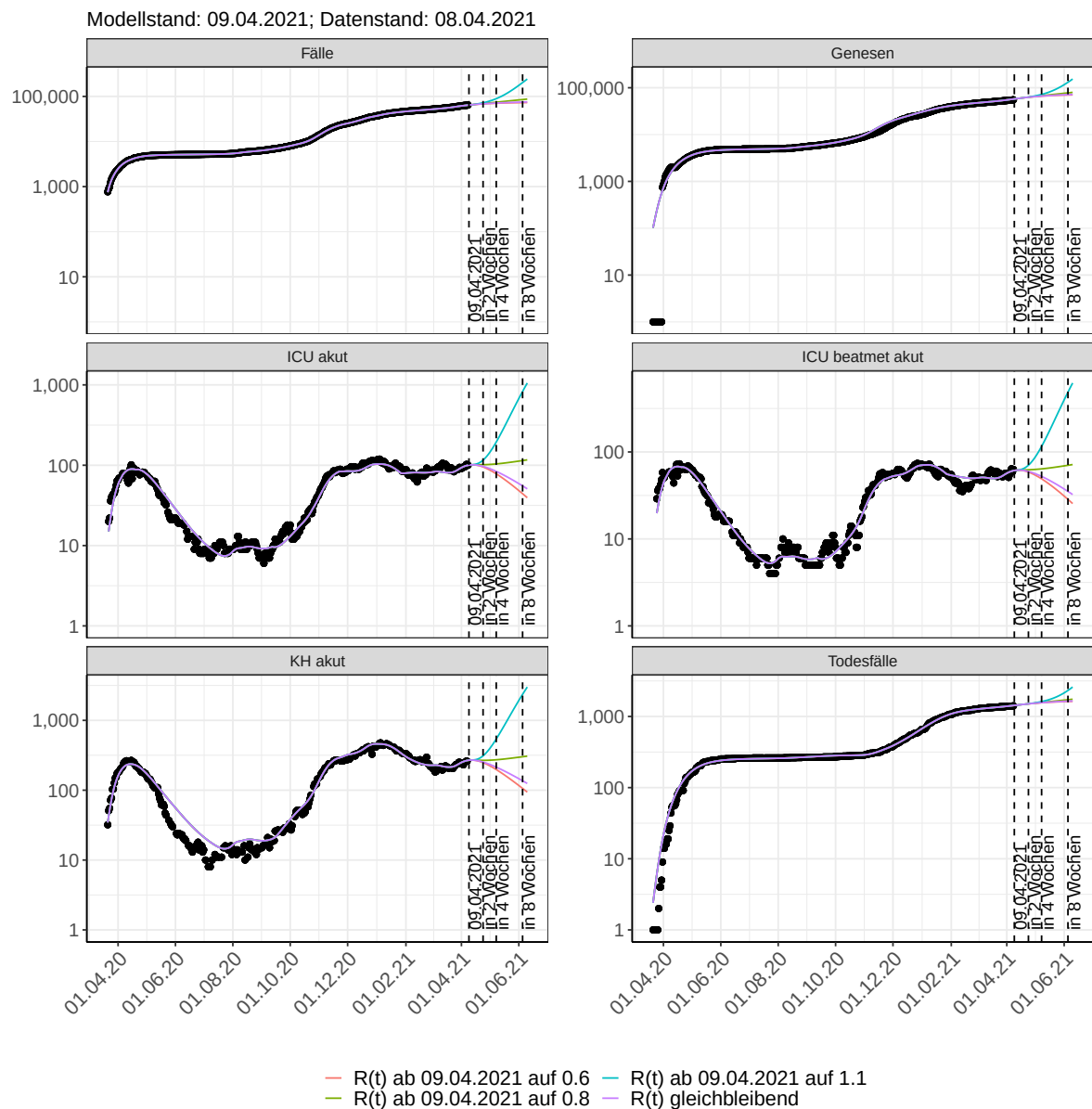
Abbildung 92: Halblogarithmische Darstellung der Modellvorhersage (Fallzahlen, Genesen, ICU Beatmet, ICU Betten, KH Betten, Todesfälle) für Hamburg unter Annahme verschiedener Szenarien nach dem 09.04.2021. Punkte: gemeldete Fallzahlen; Linien: Modellvorhersage.
