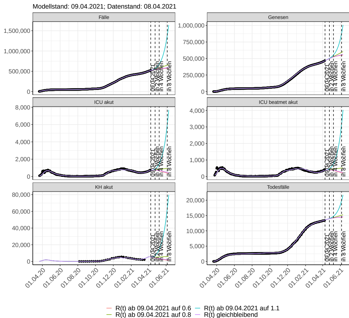
Abbildung 39: Lineare Darstellung der Modellvorhersage (Fallzahlen, Genesen, ICU Beatmet, ICU Betten, KH Betten, Todesfälle) für Bayern unter Annahme verschiedener Szenarien ab dem 09.04.2021. Punkte: gemeldete Fallzahlen; Linien: Modellvorhersage.
