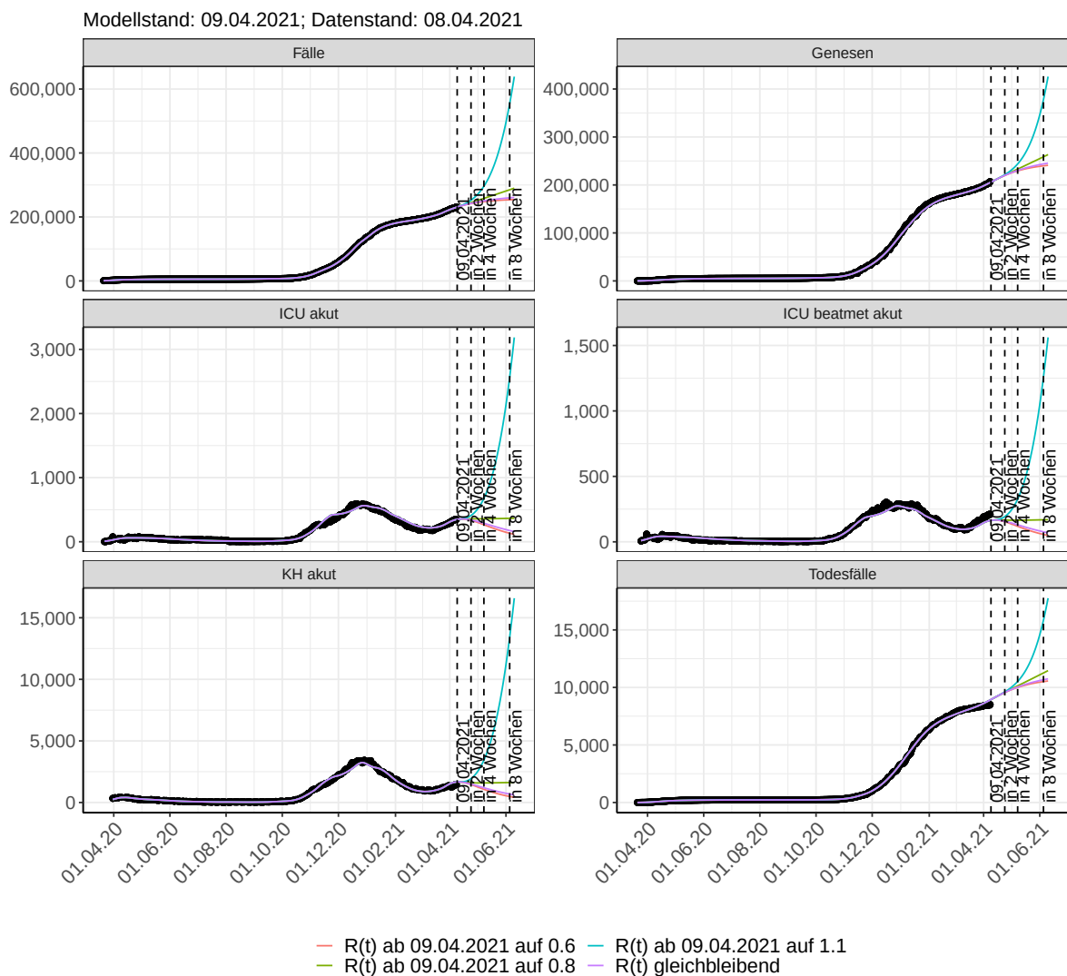
Abbildung 180: Lineare Darstellung der Modellvorhersage (Fallzahlen, Genesen, ICU Beatmet, ICU Betten, KH Betten, Todesfälle) für Sachsen unter Annahme verschiedener Szenarien ab dem 09.04.2021. Punkte: gemeldete Fallzahlen; Linien: Modellvorhersage.
