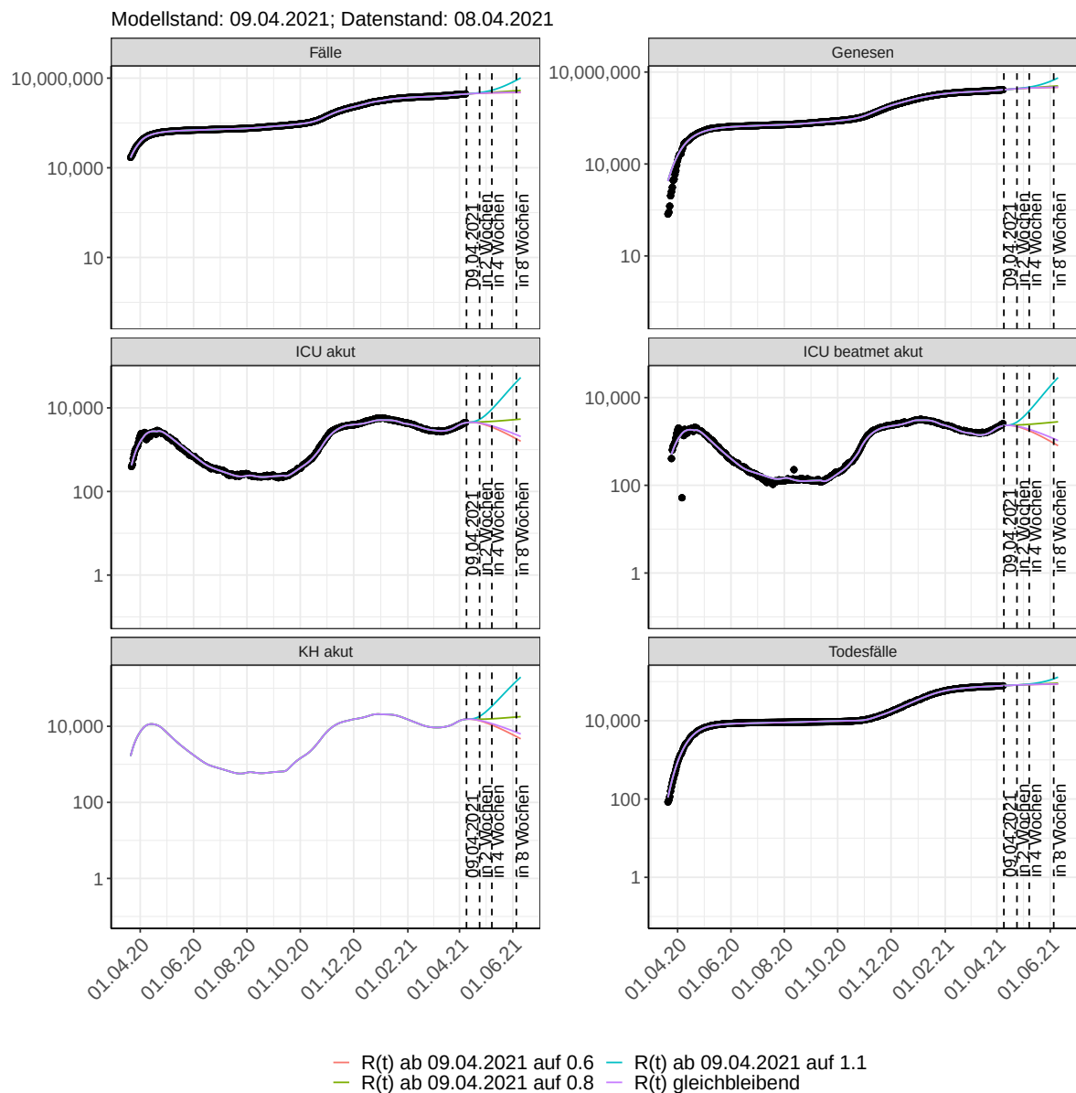
Abbildung 226: Halblogarithmische Darstellung der Modellvorhersage (Fallzahlen, Genesen, ICU Beatmet, ICU Betten, KH Betten, Todesfälle) für Deutschland unter Annahme verschiedener Szenarien ab dem 09.04.2021. Punkte: gemeldete Fallzahlen; Linien: Modellvorhersage.
