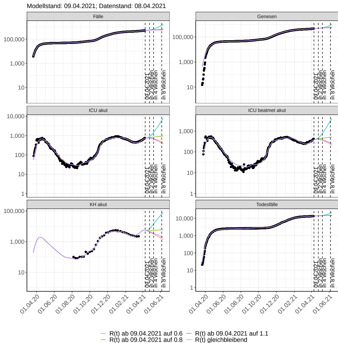
Abbildung 40: Halblogarithmische Darstellung der Modellvorhersage (Fallzahlen, Genesen, ICU Beatmet, ICU Betten, KH Betten, Todesfälle) für Bayern unter Annahme verschiedener Szenarien nach dem 09.04.2021. Punkte: gemeldete Fallzahlen; Linien: Modellvorhersage.
