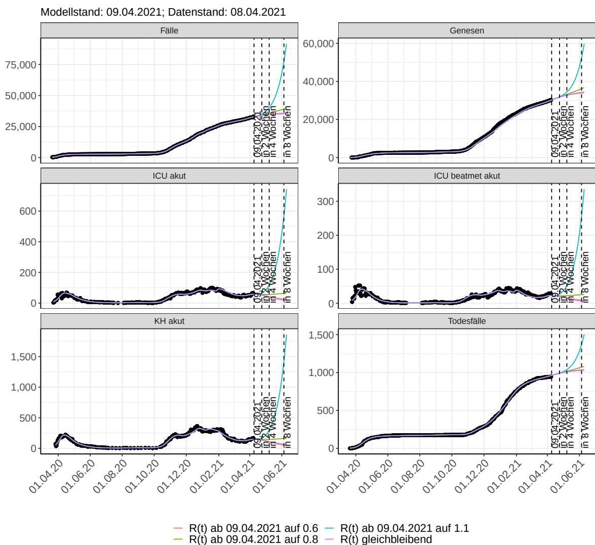
Abbildung 169: Lineare Darstellung der Modellvorhersage (Fallzahlen, Genesen, ICU Beatmet, ICU Betten, KH Betten, Todesfälle) für Saarland unter Annahme verschiedener Szenarien ab dem 09.04.2021. Punkte: gemeldete Fallzahlen; Linien: Modellvorhersage.
