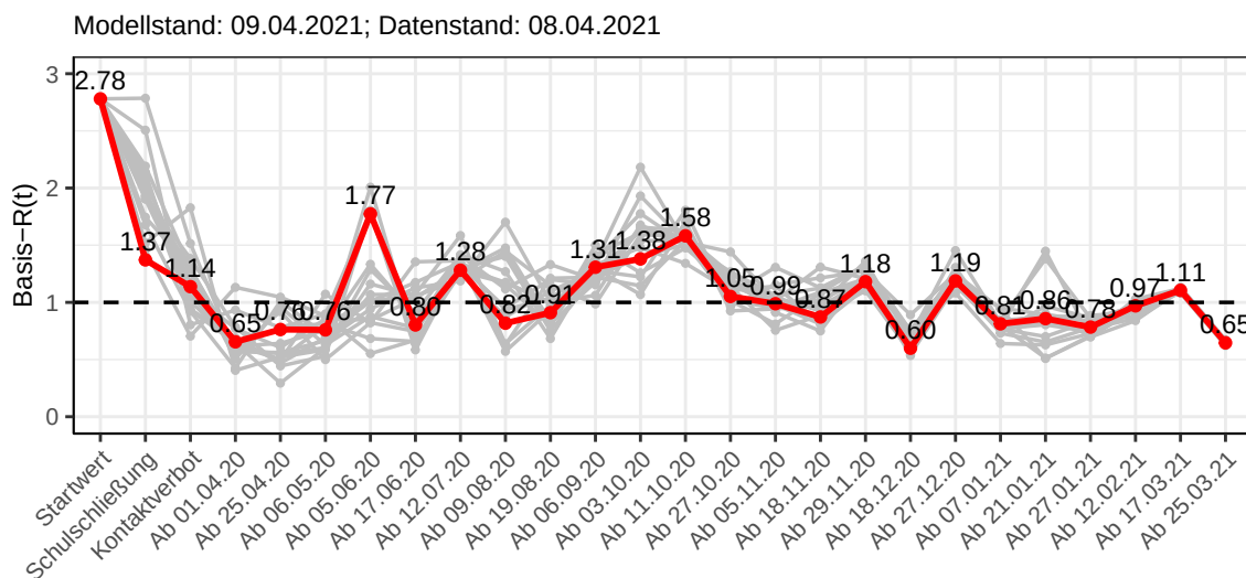
Abbildung 137: Basis- R(t) Werte vor und nach den NPIs für Nordrhein-Westfalen
