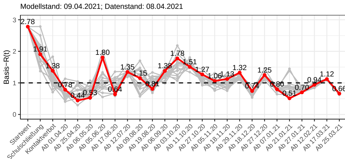
Abbildung 65: Basis- R(t) Werte vor und nach den NPIs für Brandenburg
