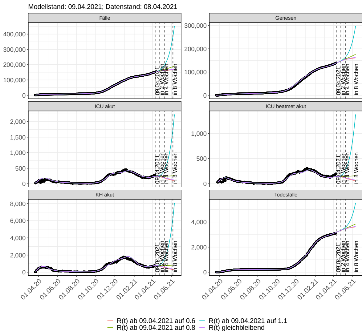
Abbildung 58: Lineare Darstellung der Modellvorhersage (Fallzahlen, Genesen, ICU Beatmet, ICU Betten, KH Betten, Todesfälle) für Berlin unter Annahme verschiedener Szenarien ab dem 09.04.2021. Punkte: gemeldete Fallzahlen; Linien: Modellvorhersage.
