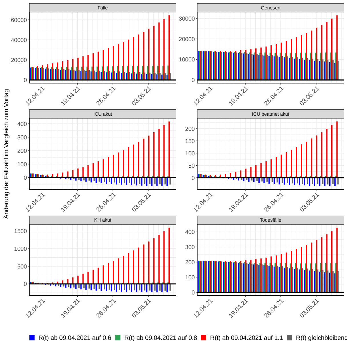
Abbildung 227: Simulation täglich neu auftretender Fälle für die nächsten 4 Wochen ab dem 09.04.2021 - Deutschland
