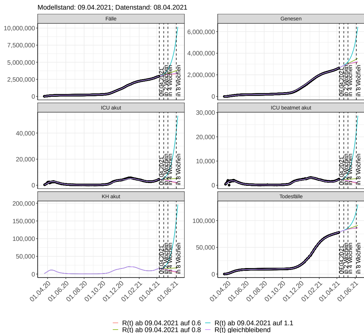
Abbildung 225: Lineare Darstellung der Modellvorhersage (Fallzahlen, Genesen, ICU Beatmet, ICU Betten, KH Betten, Todesfälle) für Deutschland unter Annahme verschiedener Szenarien ab dem 09.04.2021. Punkte: gemeldete Fallzahlen; Linien: Modellvorhersage.
