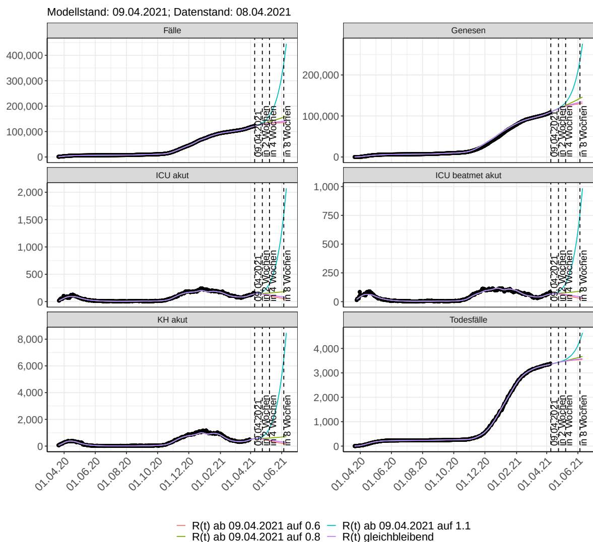
Abbildung 156: Lineare Darstellung der Modellvorhersage (Fallzahlen, Genesen, ICU Beatmet, ICU Betten, KH Betten, Todesfälle) für Rheinland-Pfalz unter Annahme verschiedener Szenarien ab dem 09.04.2021. Punkte: gemeldete Fallzahlen; Linien: Modellvorhersage.
