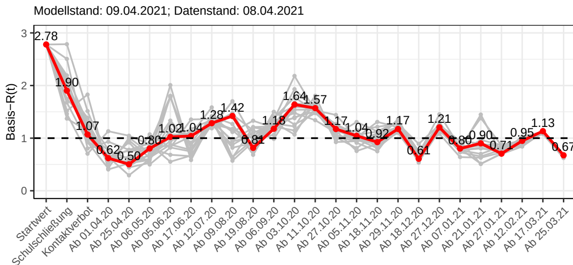
Abbildung 152: Basis- R(t) Werte vor und nach den NPIs für Rheinland-Pfalz
