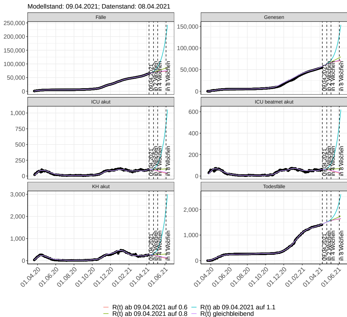
Abbildung 91: Lineare Darstellung der Modellvorhersage (Fallzahlen, Genesen, ICU Beatmet, ICU Betten, KH Betten, Todesfälle) für Hamburg unter Annahme verschiedener Szenarien ab dem 09.04.2021. Punkte: gemeldete Fallzahlen; Linien: Modellvorhersage.
