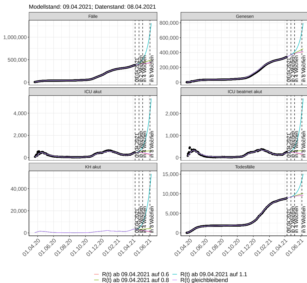
Abbildung 24: Lineare Darstellung der Modellvorhersage (Fallzahlen, Genesen, ICU Beatmet, ICU Betten, KH Betten, Todesfälle) für Baden-Württemberg unter Annahme verschiedener Szenarien ab dem 09.04.2021. Punkte: gemeldete Fallzahlen; Linien: Modellvorhersage.
