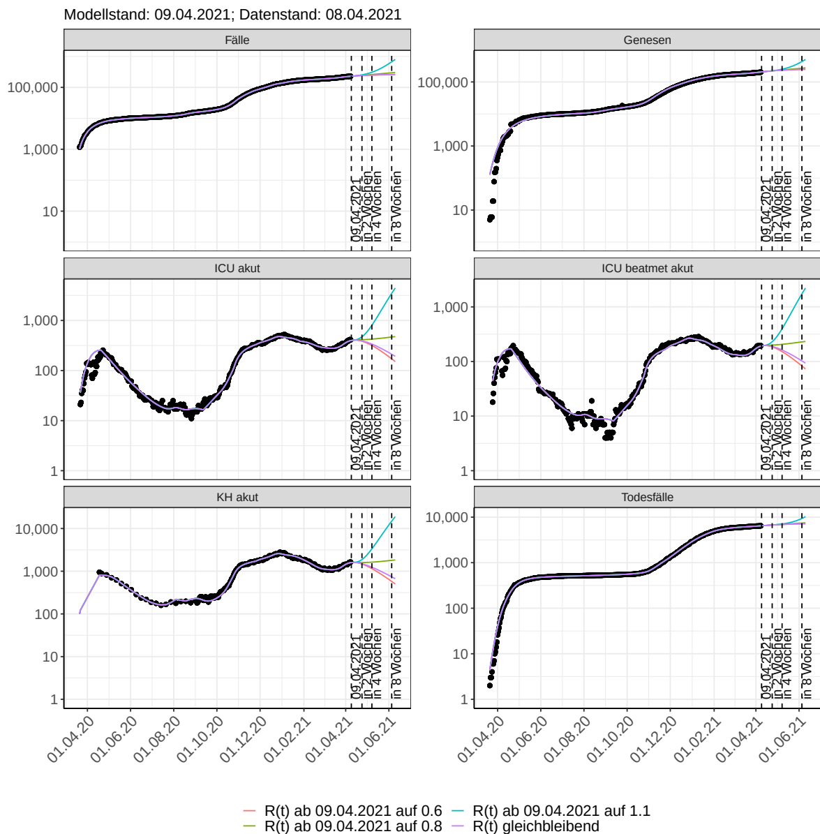
Abbildung 103: Halblogarithmische Darstellung der Modellvorhersage (Fallzahlen, Genesen, ICU Beatmet, ICU Betten, KH Betten, Todesfälle) für Hessen unter Annahme verschiedener Szenarien nach dem 09.04.2021. Punkte: gemeldete Fallzahlen; Linien: Modellvorhersage.
