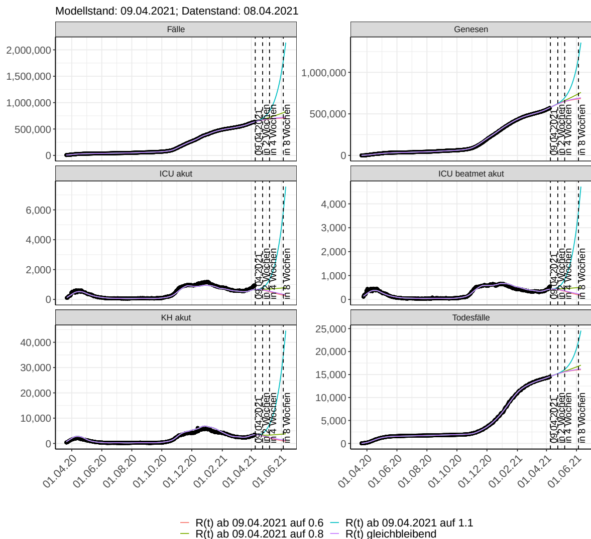
Abbildung 141: Lineare Darstellung der Modellvorhersage (Fallzahlen, Genesen, ICU Beatmet, ICU Betten, KH Betten, Todesfälle) für Nordrhein-Westfalen unter Annahme verschiedener Szenarien ab dem 09.04.2021. Punkte: gemeldete Fallzahlen; Linien: Modellvorhersage.
