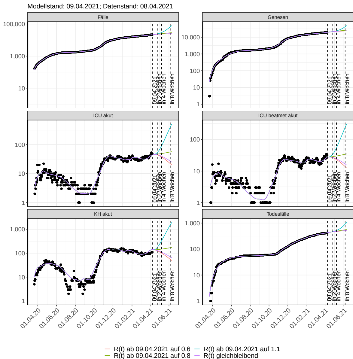
Abbildung 81: Halblogarithmische Darstellung der Modellvorhersage (Fallzahlen, Genesen, ICU Beatmet, ICU Betten, KH Betten, Todesfälle) für Bremen unter Annahme verschiedener Szenarien nach dem 09.04.2021. Punkte: gemeldete Fallzahlen; Linien: Modellvorhersage.
