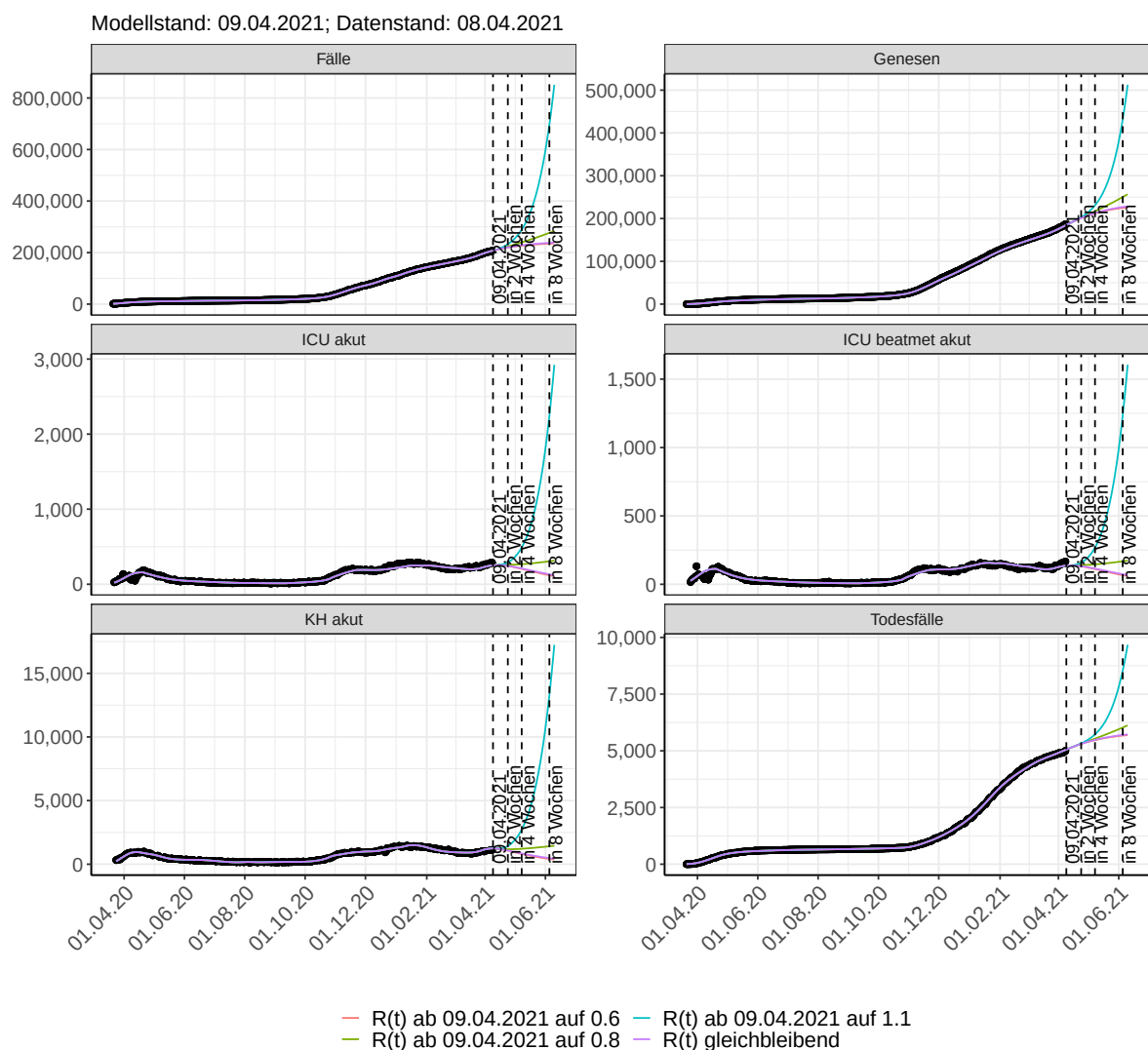
Abbildung 126: Lineare Darstellung der Modellvorhersage (Fallzahlen, Genesen, ICU Beatmet, ICU Betten, KH Betten, Todesfälle) für Niedersachsen unter Annahme verschiedener Szenarien ab dem 09.04.2021. Punkte: gemeldete Fallzahlen; Linien: Modellvorhersage.
