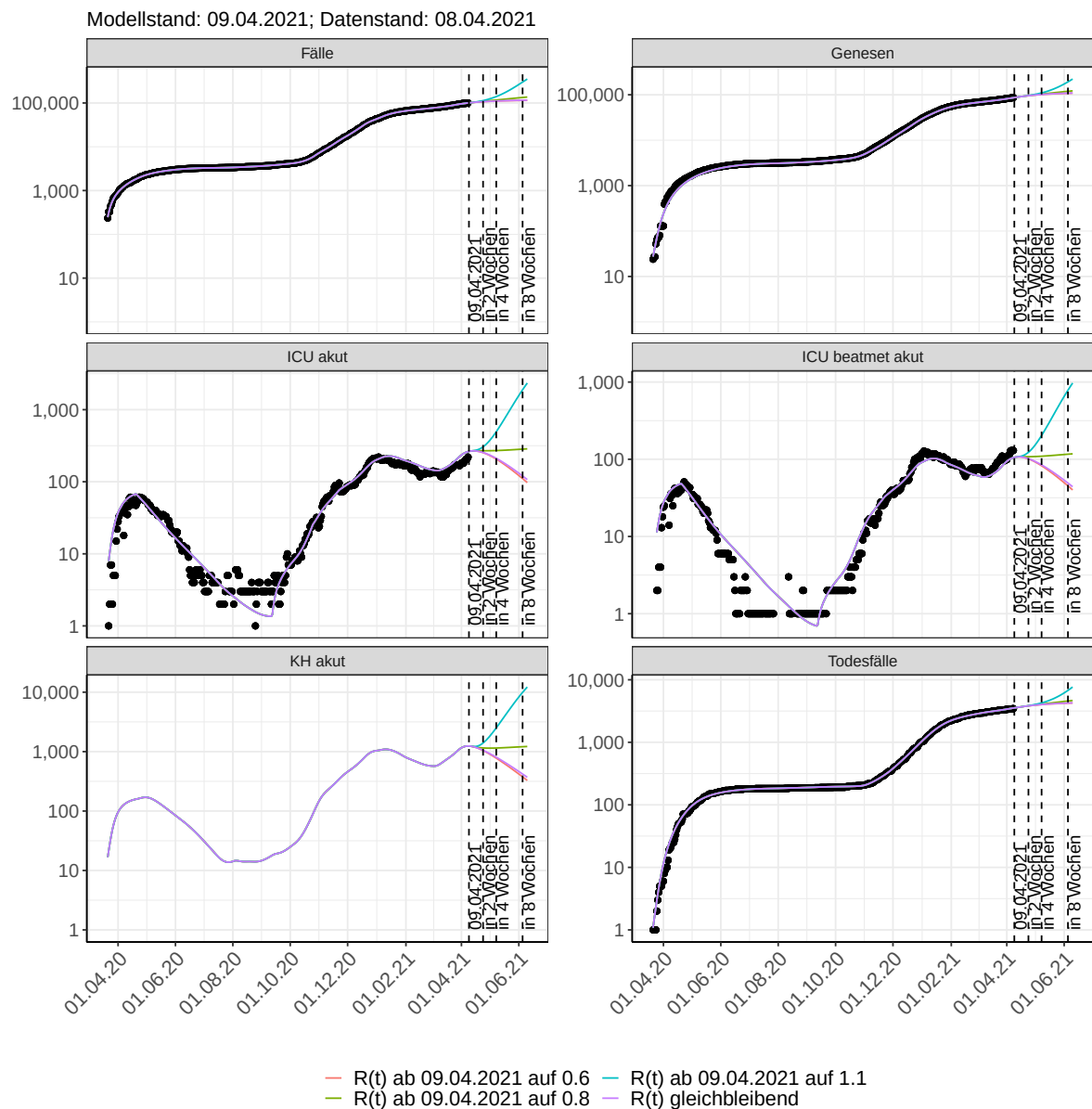
Abbildung 214: Halblogarithmische Darstellung der Modellvorhersage (Fallzahlen, Genesen, ICU Beatmet, ICU Betten, KH Betten, Todesfälle) für Thüringen unter Annahme verschiedener Szenarien nach dem 09.04.2021. Punkte: gemeldete Fallzahlen; Linien: Modellvorhersage.
