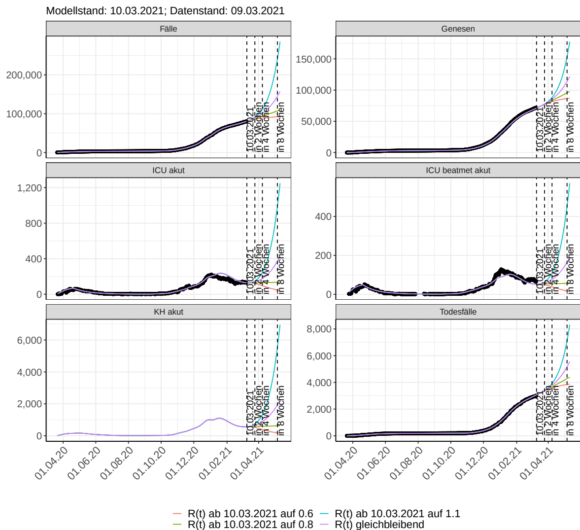
Abbildung 213: Lineare Darstellung der Modellvorhersage (Fallzahlen, Genesen, ICU Beatmet, ICU Betten, KH Betten, Todesfälle) für Thüringen unter Annahme verschiedener Szenarien ab dem 10.03.2021. Punkte: gemeldete Fallzahlen; Linien: Modellvorhersage.
