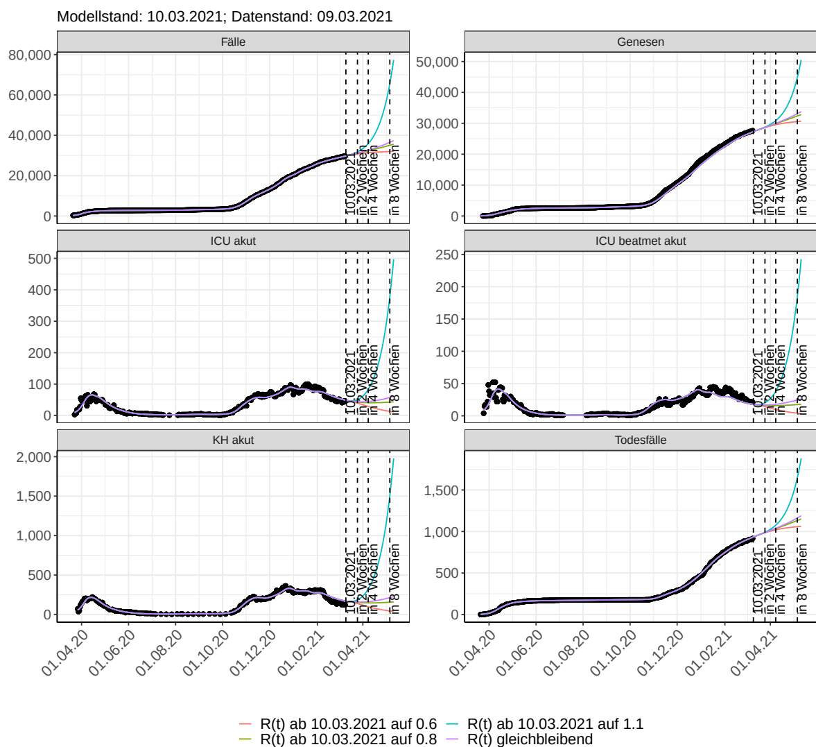
Abbildung 169: Lineare Darstellung der Modellvorhersage (Fallzahlen, Genesen, ICU Beatmet, ICU Betten, KH Betten, Todesfälle) für Saarland unter Annahme verschiedener Szenarien ab dem 10.03.2021. Punkte: gemeldete Fallzahlen; Linien: Modellvorhersage.
