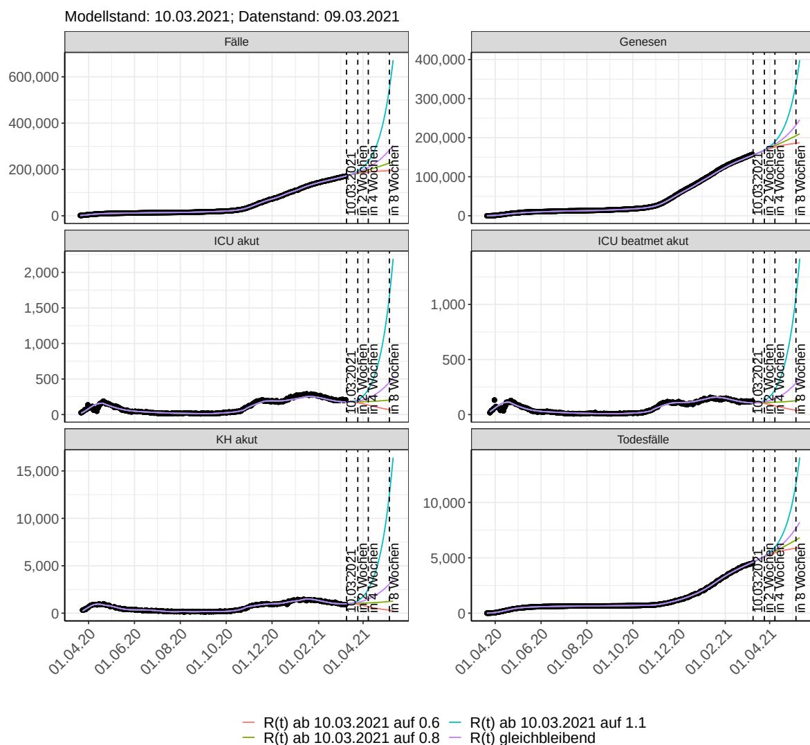
Abbildung 126: Lineare Darstellung der Modellvorhersage (Fallzahlen, Genesen, ICU Beatmet, ICU Betten, KH Betten, Todesfälle) für Niedersachsen unter Annahme verschiedener Szenarien ab dem 10.03.2021. Punkte: gemeldete Fallzahlen; Linien: Modellvorhersage.
