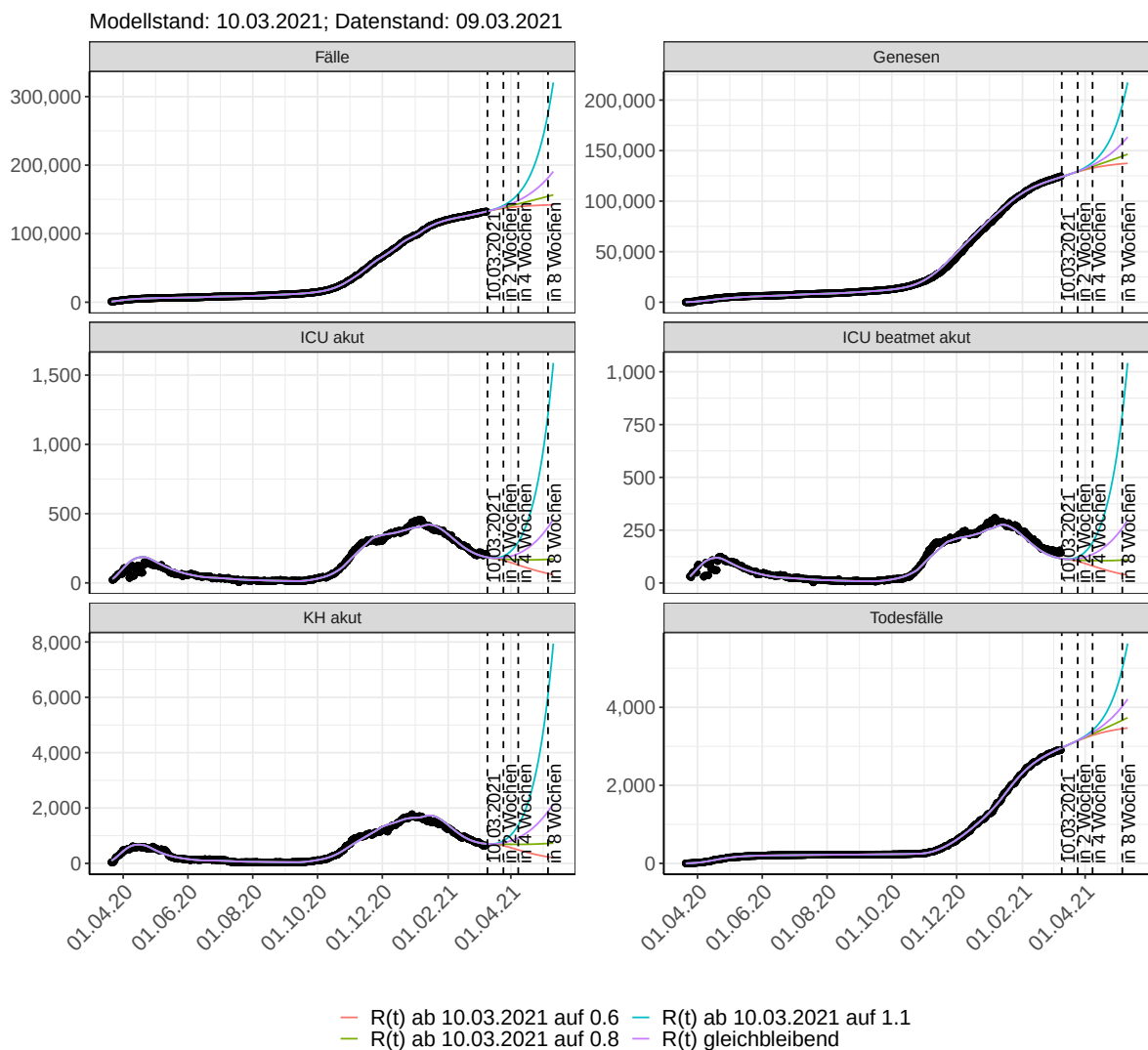
Abbildung 58: Lineare Darstellung der Modellvorhersage (Fallzahlen, Genesen, ICU Beatmet, ICU Betten, KH Betten, Todesfälle) für Berlin unter Annahme verschiedener Szenarien ab dem 10.03.2021. Punkte: gemeldete Fallzahlen; Linien: Modellvorhersage.
