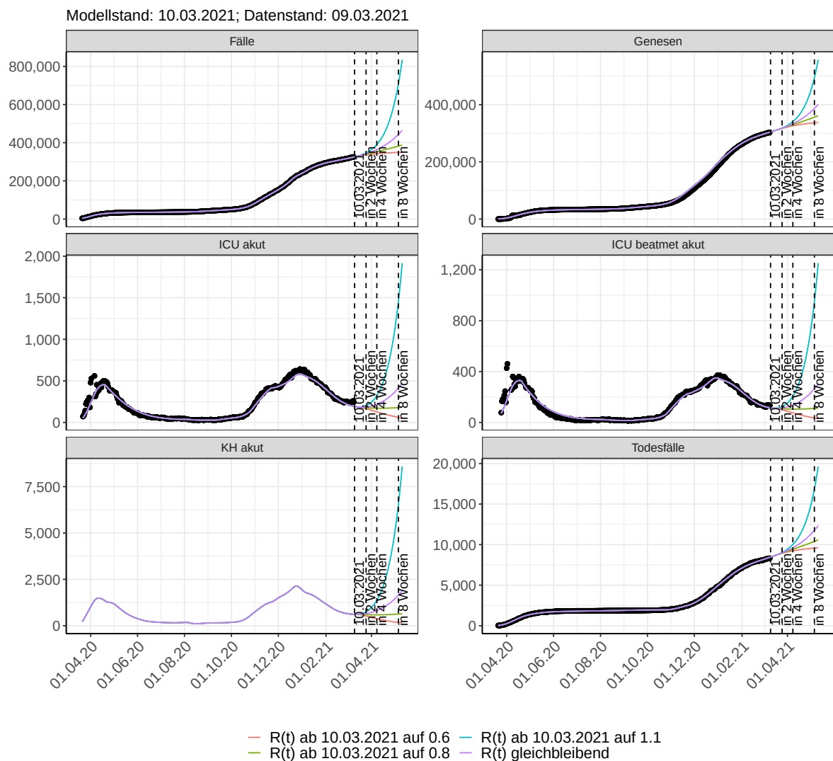
Abbildung 24: Lineare Darstellung der Modellvorhersage (Fallzahlen, Genesen, ICU Beatmet, ICU Betten, KH Betten, Todesfälle) für Baden-Württemberg unter Annahme verschiedener Szenarien ab dem 10.03.2021. Punkte: gemeldete Fallzahlen; Linien: Modellvorhersage.
