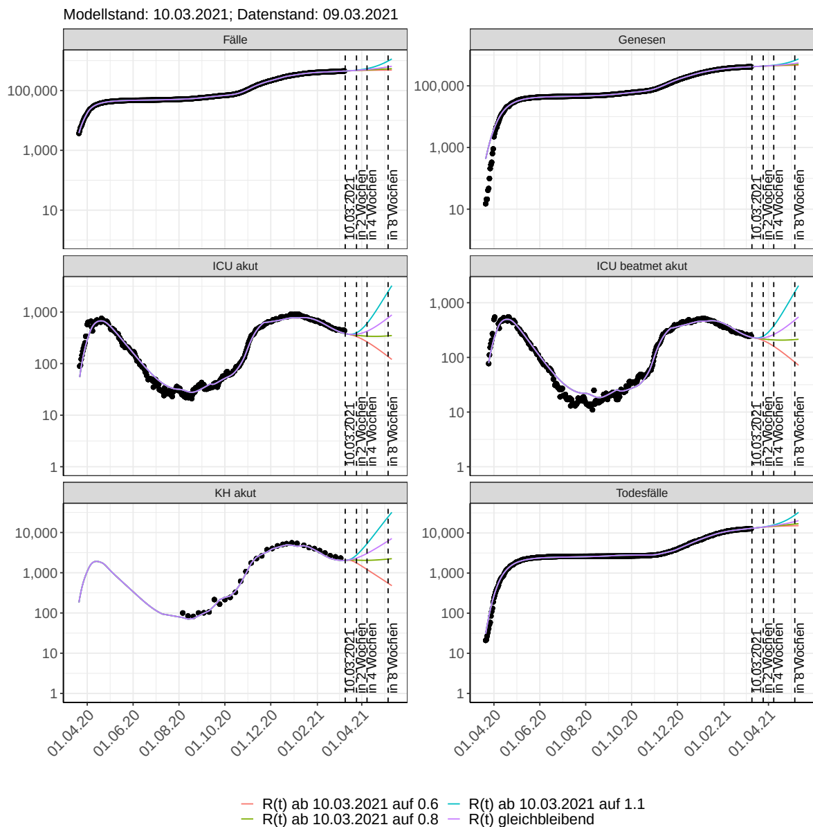
Abbildung 40: Halblogarithmische Darstellung der Modellvorhersage (Fallzahlen, Genesen, ICU Beatmet, ICU Betten, KH Betten, Todesfälle) für Bayern unter Annahme verschiedener Szenarien nach dem 10.03.2021. Punkte: gemeldete Fallzahlen; Linien: Modellvorhersage.
