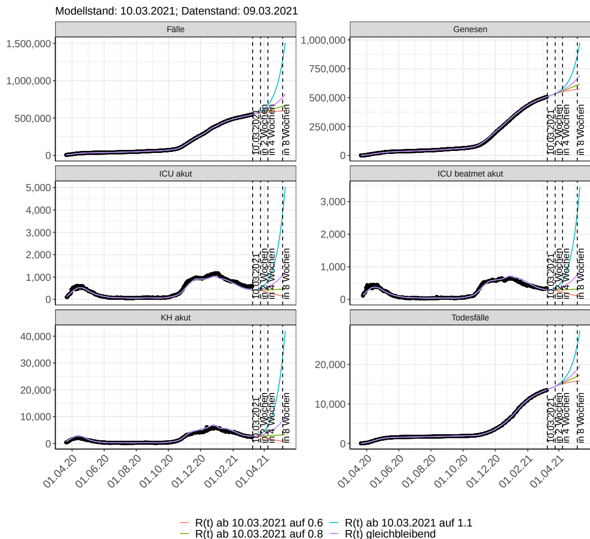
Abbildung 141: Lineare Darstellung der Modellvorhersage (Fallzahlen, Genesen, ICU Beatmet, ICU Betten, KH Betten, Todesfälle) für Nordrhein-Westfalen unter Annahme verschiedener Szenarien ab dem 10.03.2021. Punkte: gemeldete Fallzahlen; Linien: Modellvorhersage.
