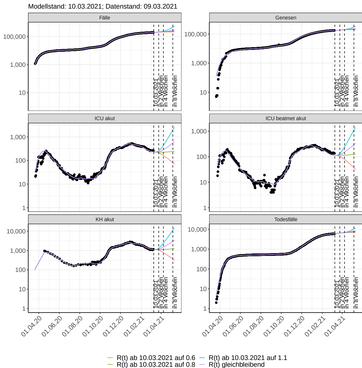
Abbildung 103: Halblogarithmische Darstellung der Modellvorhersage (Fallzahlen, Genesen, ICU Beatmet, ICU Betten, KH Betten, Todesfälle) für Hessen unter Annahme verschiedener Szenarien nach dem 10.03.2021. Punkte: gemeldete Fallzahlen; Linien: Modellvorhersage.
