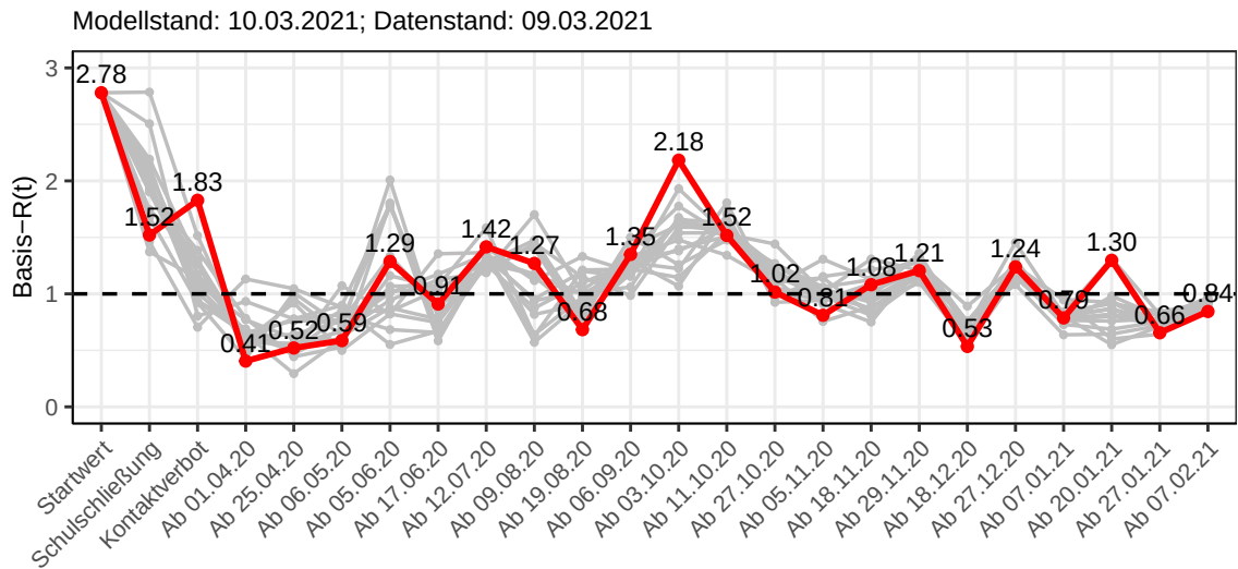
Abbildung 165: Basis- R(t) Werte vor und nach den NPIs für Saarland
