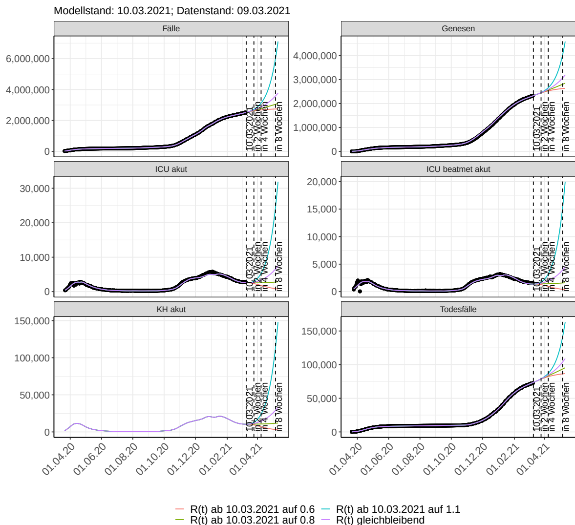
Abbildung 225: Lineare Darstellung der Modellvorhersage (Fallzahlen, Genesen, ICU Beatmet, ICU Betten, KH Betten, Todesfälle) für Deutschland unter Annahme verschiedener Szenarien ab dem 10.03.2021. Punkte: gemeldete Fallzahlen; Linien: Modellvorhersage.
