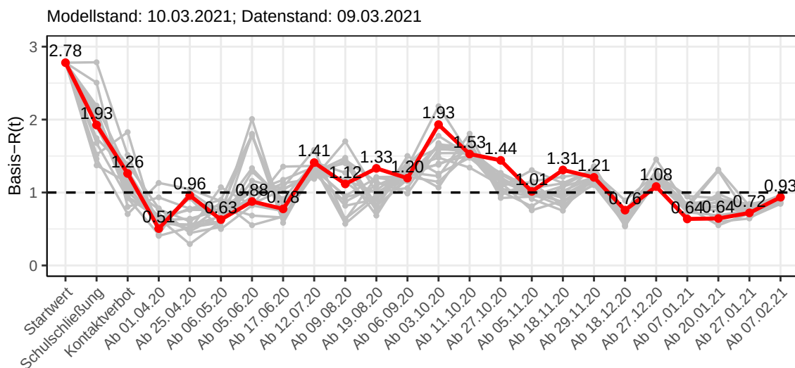
Abbildung 176: Basis- R(t) Werte vor und nach den NPIs für Sachsen
