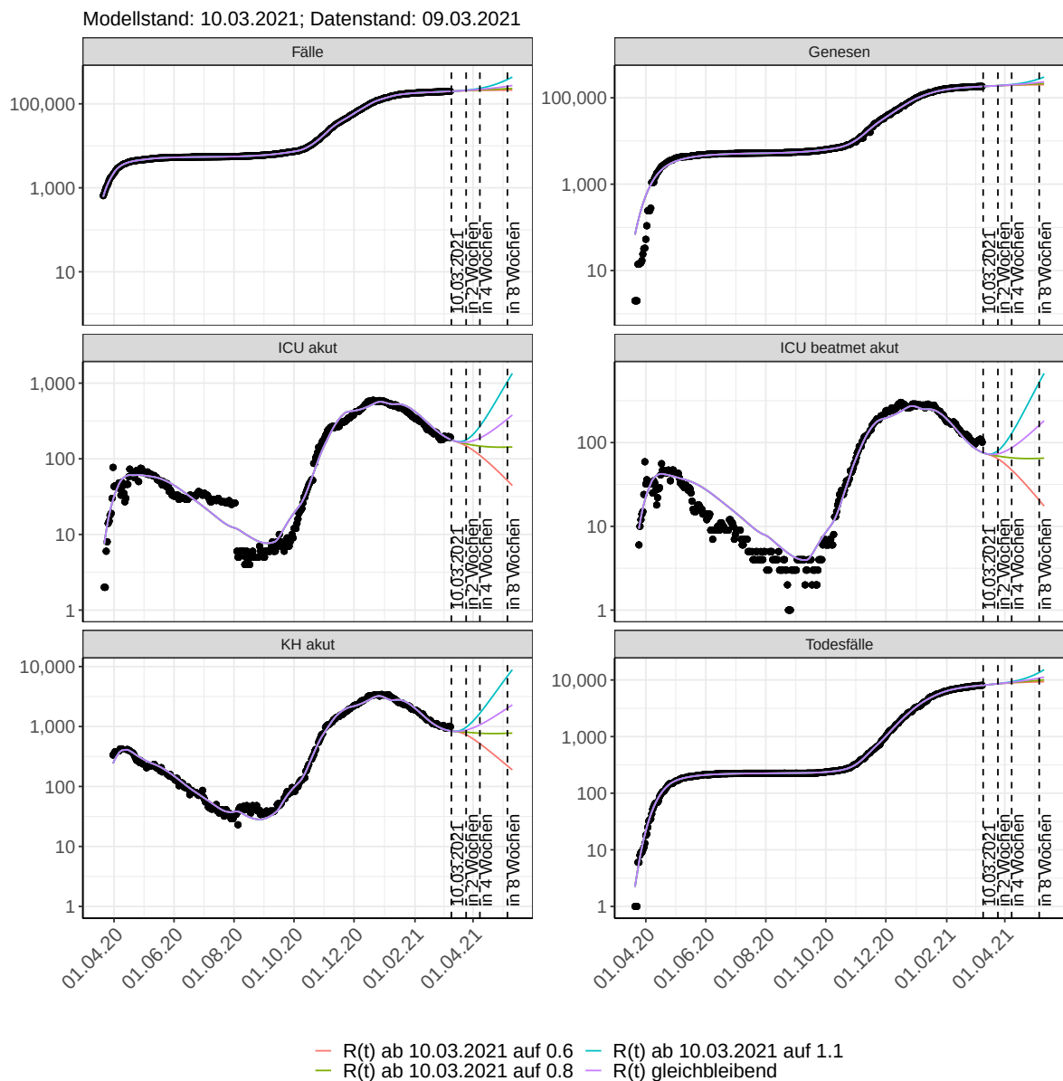
Abbildung 181: Halblogarithmische Darstellung der Modellvorhersage (Fallzahlen, Genesen, ICU Beatmet, ICU Betten, KH Betten, Todesfälle) für Sachsen unter Annahme verschiedener Szenarien nach dem 10.03.2021. Punkte: gemeldete Fallzahlen; Linien: Modellvorhersage.
