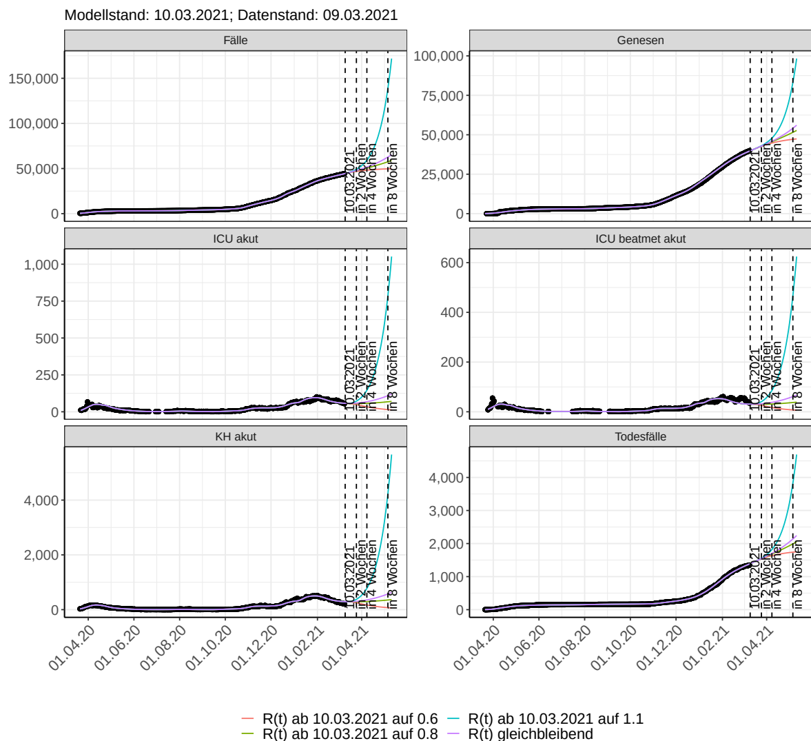
Abbildung 202: Lineare Darstellung der Modellvorhersage (Fallzahlen, Genesen, ICU Beatmet, ICU Betten, KH Betten, Todesfälle) für Schleswig-Holstein unter Annahme verschiedener Szenarien ab dem 10.03.2021. Punkte: gemeldete Fallzahlen; Linien: Modellvorhersage.
