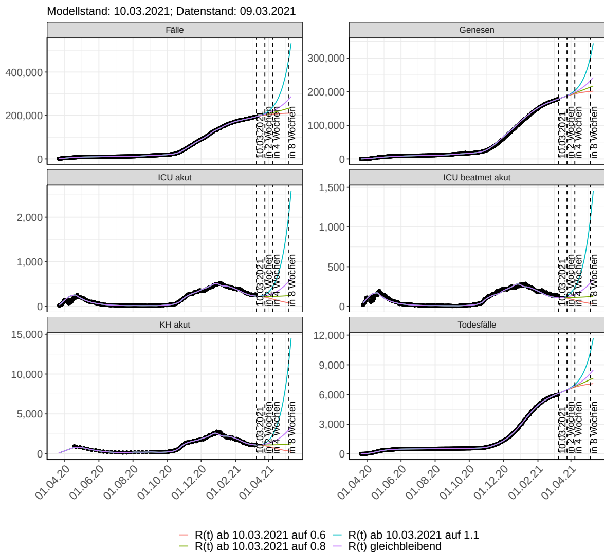
Abbildung 102: Lineare Darstellung der Modellvorhersage (Fallzahlen, Genesen, ICU Beatmet, ICU Betten, KH Betten, Todesfälle) für Hessen unter Annahme verschiedener Szenarien ab dem 10.03.2021. Punkte: gemeldete Fallzahlen; Linien: Modellvorhersage.
