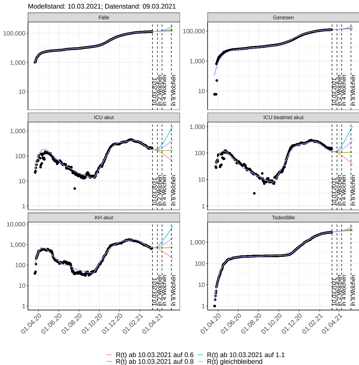
Abbildung 59: Halblogarithmische Darstellung der Modellvorhersage (Fallzahlen, Genesen, ICU Beatmet, ICU Betten, KH Betten, Todesfälle) für Berlin unter Annahme verschiedener Szenarien nach dem 10.03.2021. Punkte: gemeldete Fallzahlen; Linien: Modellvorhersage.
