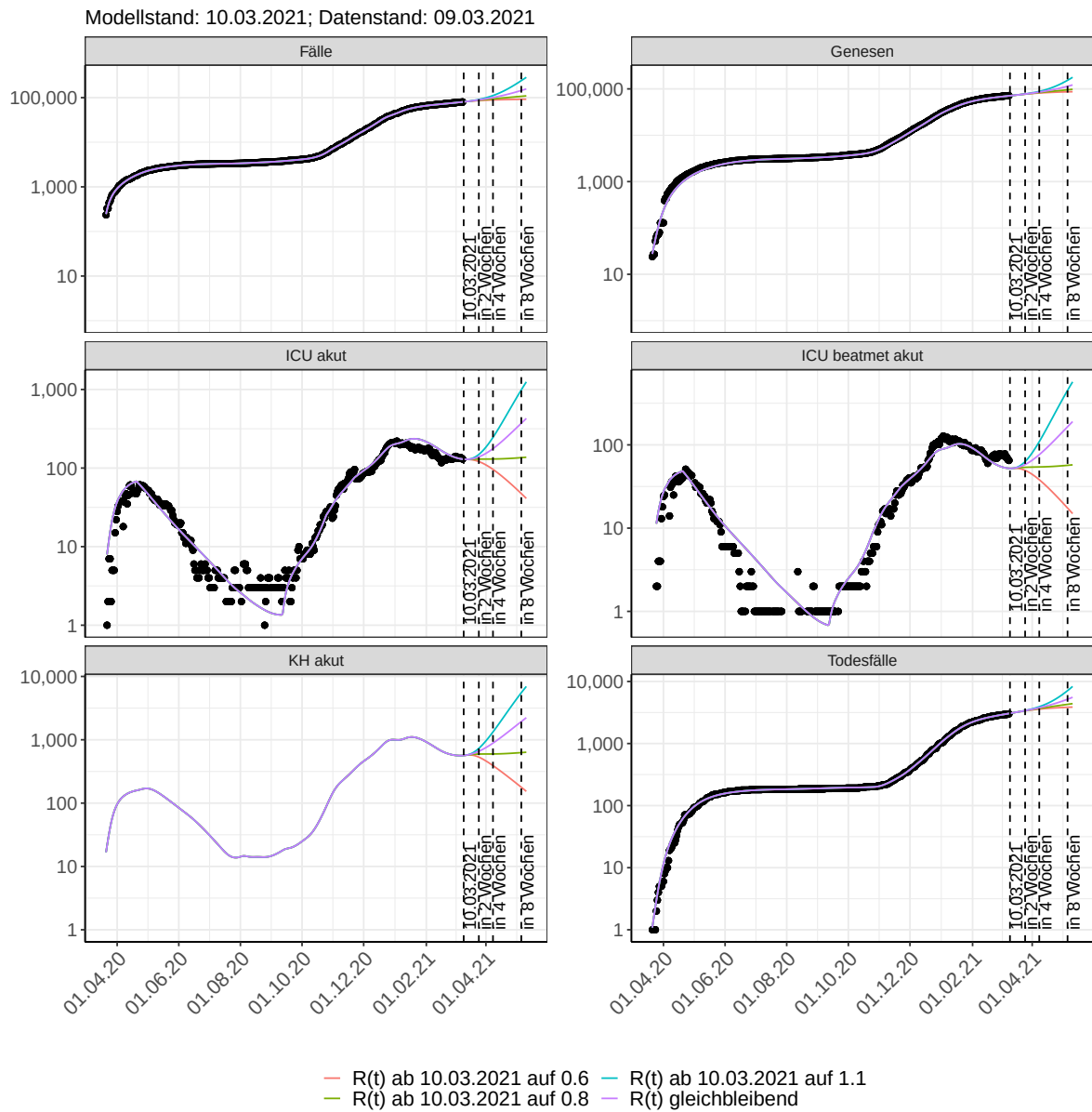
Abbildung 214: Halblogarithmische Darstellung der Modellvorhersage (Fallzahlen, Genesen, ICU Beatmet, ICU Betten, KH Betten, Todesfälle) für Thüringen unter Annahme verschiedener Szenarien nach dem 10.03.2021. Punkte: gemeldete Fallzahlen; Linien: Modellvorhersage.
