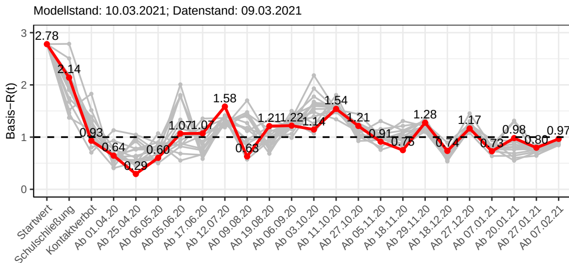
Abbildung 87: Basis- R(t) Werte vor und nach den NPIs für Hamburg
