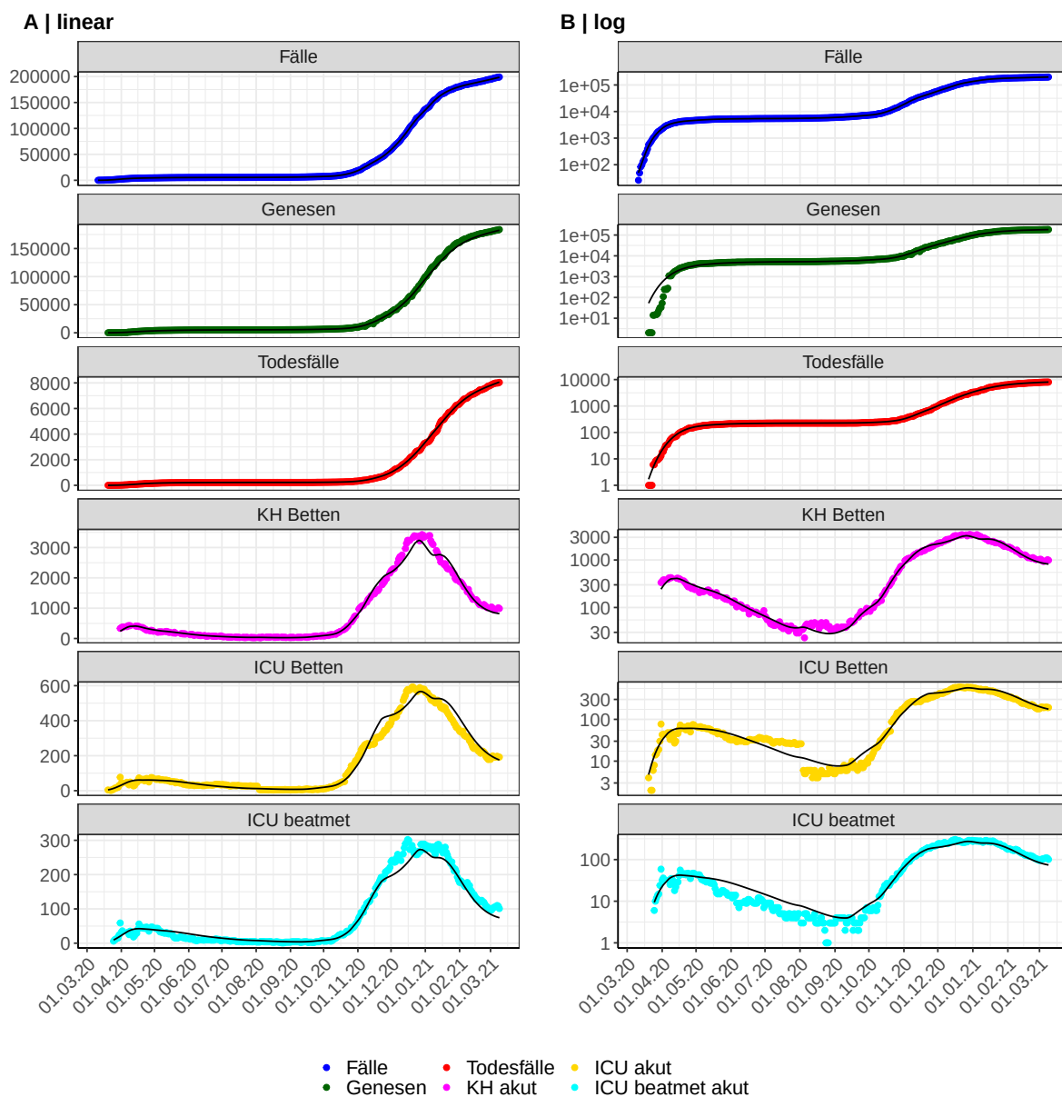
Abbildung 174: Modellbeschreibung der gemeldeten Fallzahlen, Belegung von KH Betten, Genesen und Todesfällen in Sachsen. Punkte: gemeldete Daten; Linie: Modellbeschreibung.
