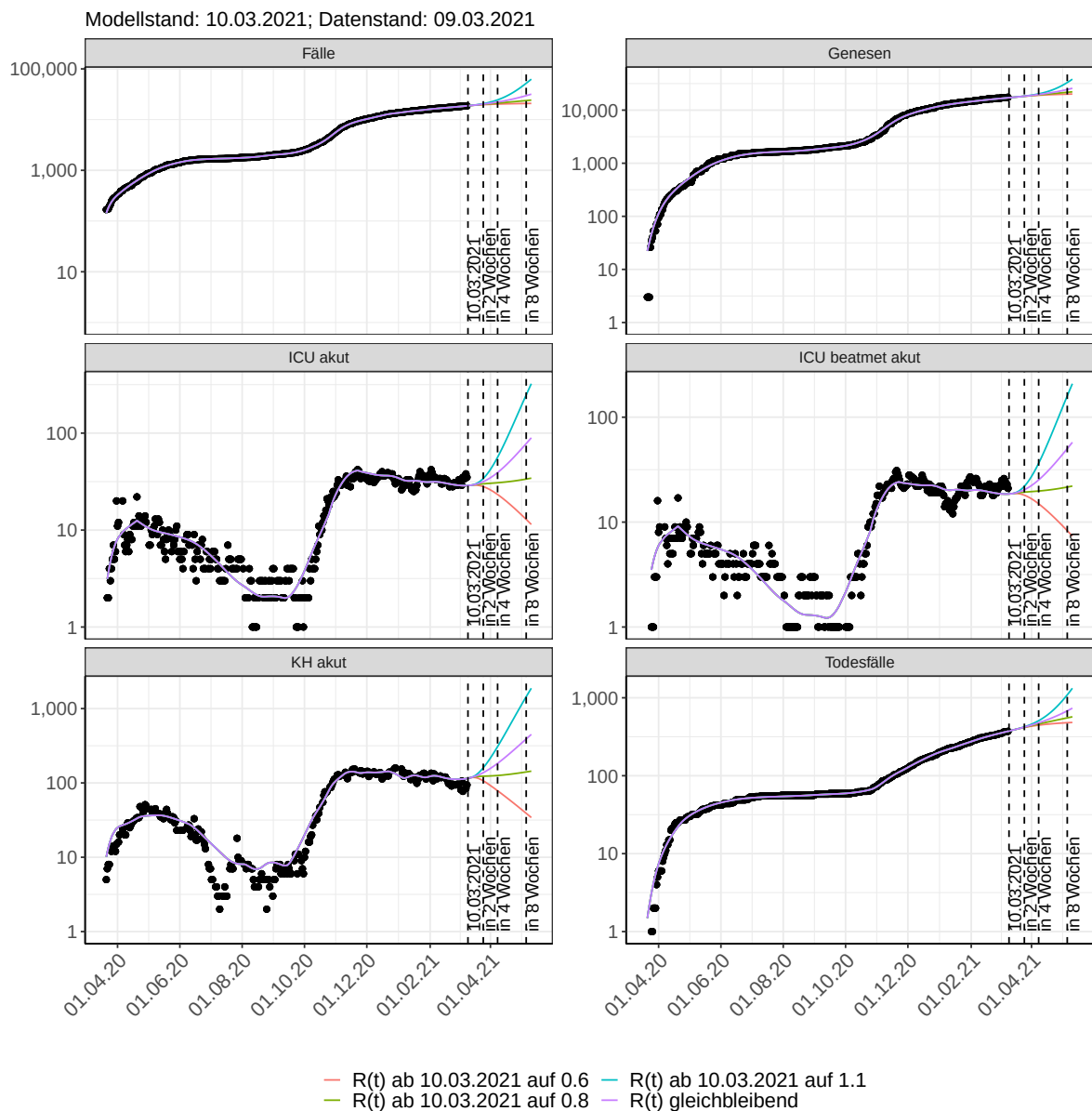
Abbildung 81: Halblogarithmische Darstellung der Modellvorhersage (Fallzahlen, Genesen, ICU Beatmet, ICU Betten, KH Betten, Todesfälle) für Bremen unter Annahme verschiedener Szenarien nach dem 10.03.2021. Punkte: gemeldete Fallzahlen; Linien: Modellvorhersage.
