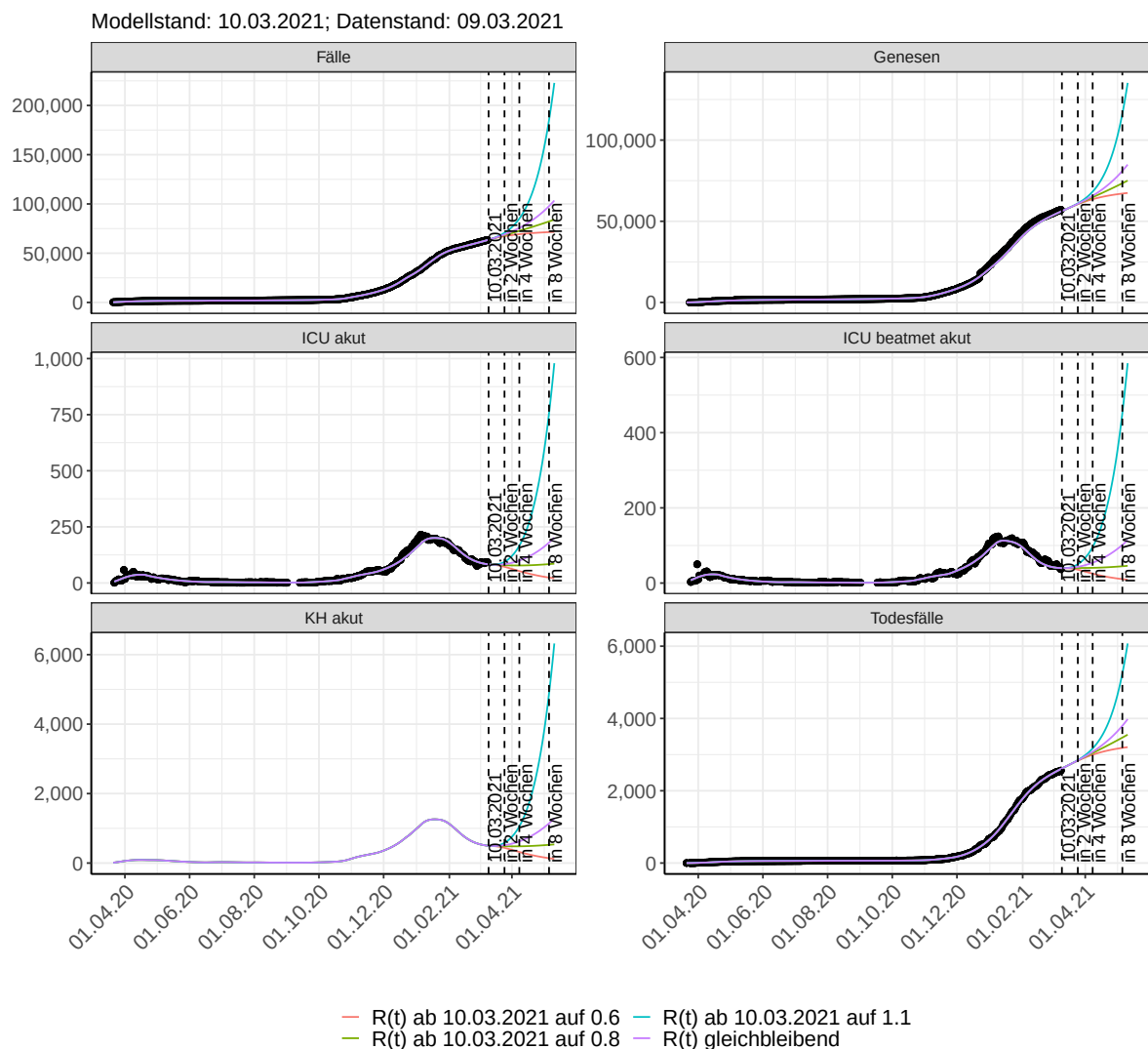
Abbildung 191: Lineare Darstellung der Modellvorhersage (Fallzahlen, Genesen, ICU Beatmet, ICU Betten, KH Betten, Todesfälle) für Sachsen-Anhalt unter Annahme verschiedener Szenarien ab dem 10.03.2021. Punkte: gemeldete Fallzahlen; Linien: Modellvorhersage.
