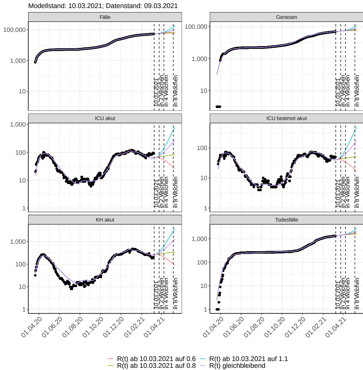
Abbildung 92: Halblogarithmische Darstellung der Modellvorhersage (Fallzahlen, Genesen, ICU Beatmet, ICU Betten, KH Betten, Todesfälle) für Hamburg unter Annahme verschiedener Szenarien nach dem 10.03.2021. Punkte: gemeldete Fallzahlen; Linien: Modellvorhersage.
