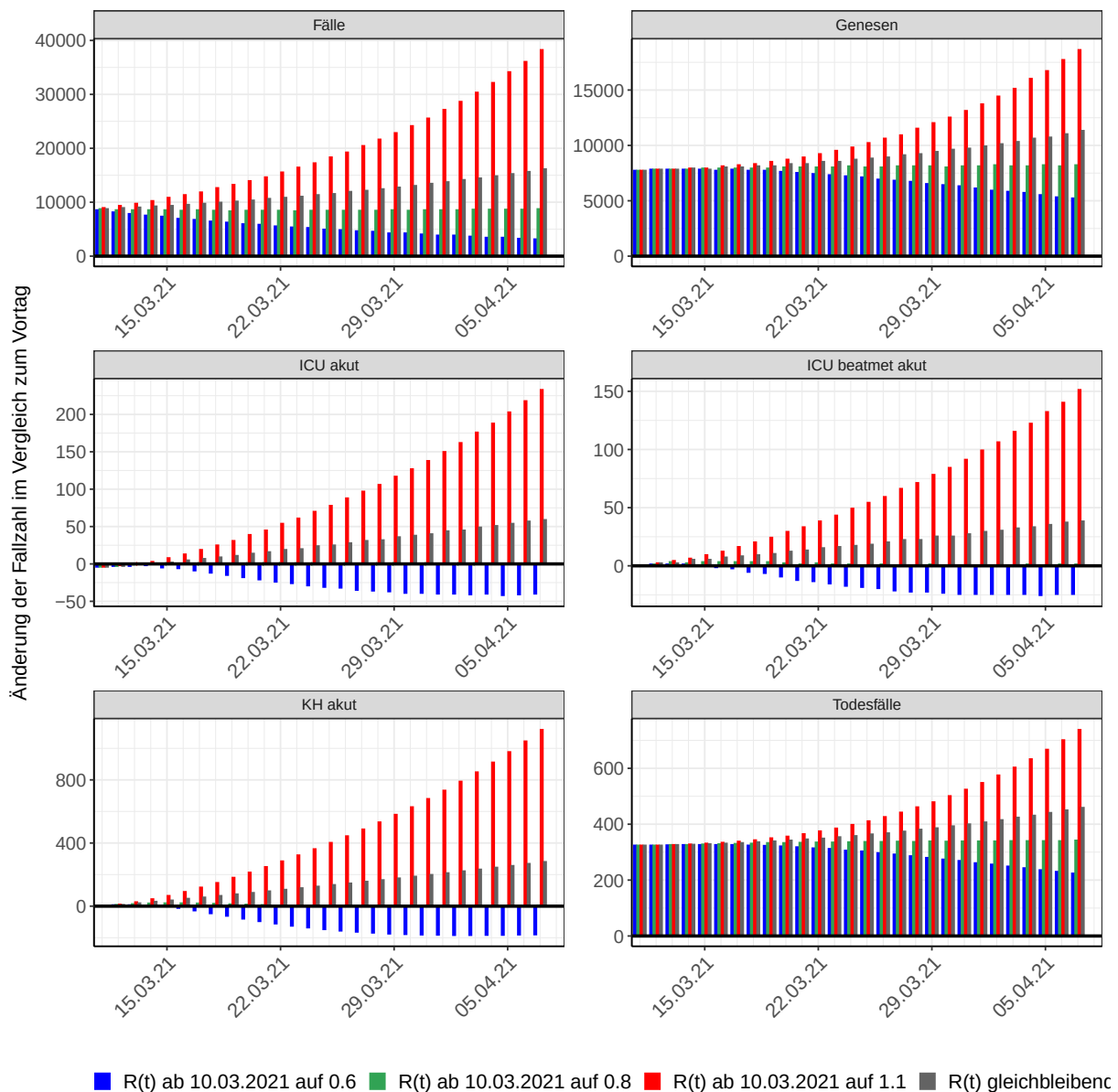
Abbildung 227: Simulation täglich neu auftretender Fälle für die nächsten 4 Wochen ab dem 10.03.2021 - Deutschland
