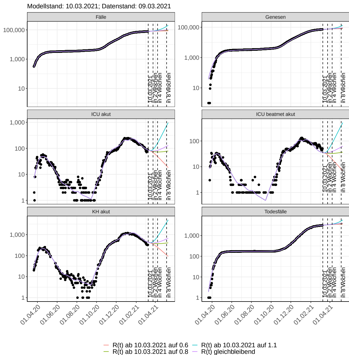
Abbildung 70: Halblogarithmische Darstellung der Modellvorhersage (Fallzahlen, Genesen, ICU Beatmet, ICU Betten, KH Betten, Todesfälle) für Brandenburg unter Annahme verschiedener Szenarien nach dem 10.03.2021. Punkte: gemeldete Fallzahlen; Linien: Modellvorhersage.
