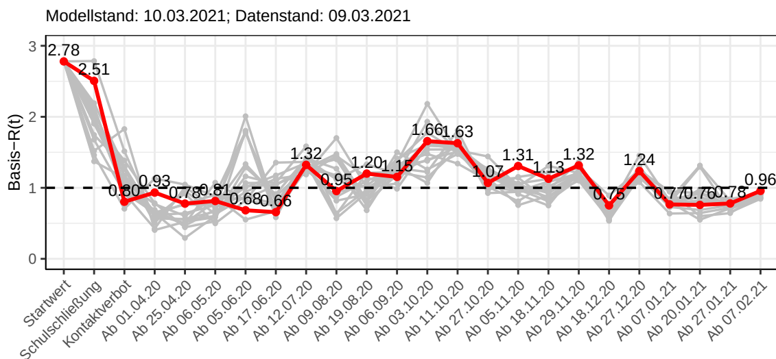
Abbildung 209: Basis- R(t) Werte vor und nach den NPIs für Thüringen
