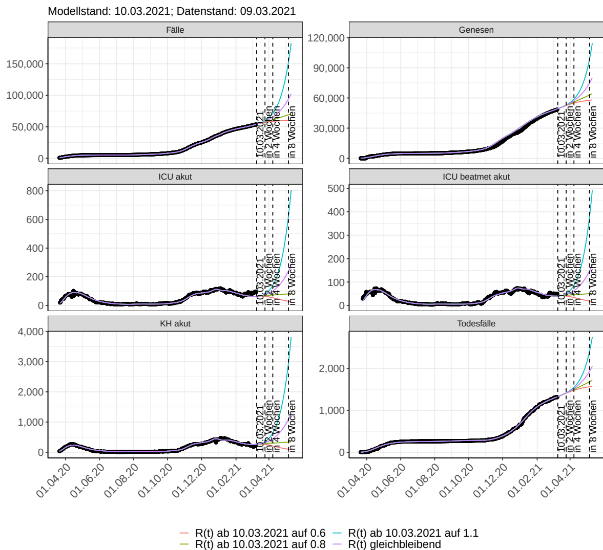
Abbildung 91: Lineare Darstellung der Modellvorhersage (Fallzahlen, Genesen, ICU Beatmet, ICU Betten, KH Betten, Todesfälle) für Hamburg unter Annahme verschiedener Szenarien ab dem 10.03.2021. Punkte: gemeldete Fallzahlen; Linien: Modellvorhersage.
