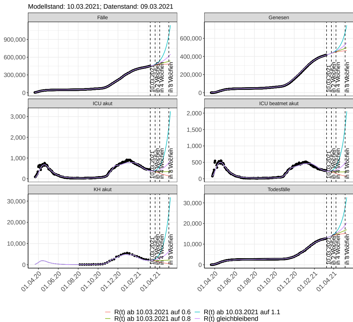
Abbildung 39: Lineare Darstellung der Modellvorhersage (Fallzahlen, Genesen, ICU Beatmet, ICU Betten, KH Betten, Todesfälle) für Bayern unter Annahme verschiedener Szenarien ab dem 10.03.2021. Punkte: gemeldete Fallzahlen; Linien: Modellvorhersage.
