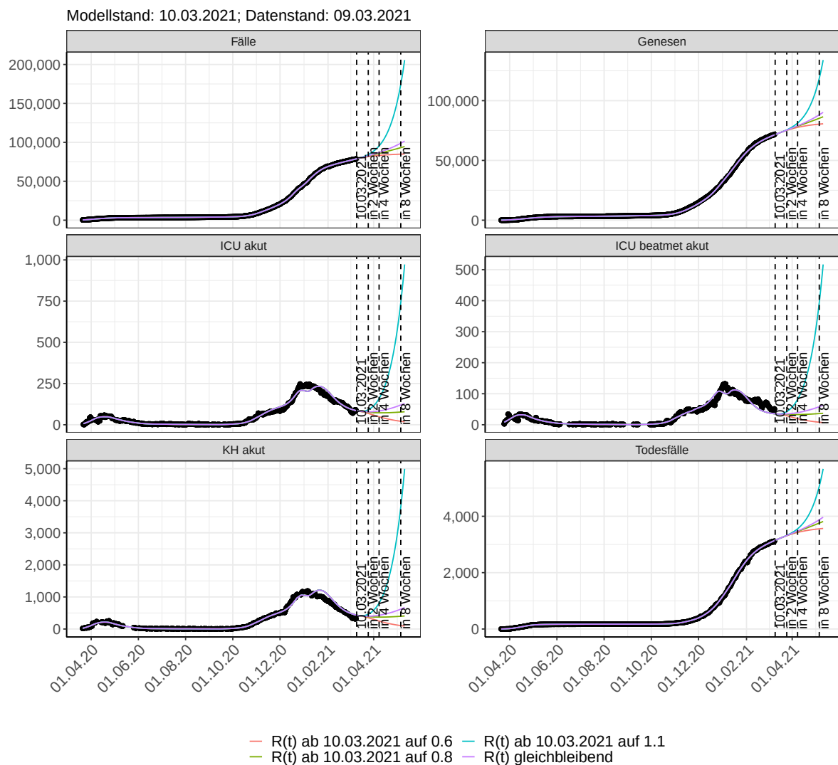
Abbildung 69: Lineare Darstellung der Modellvorhersage (Fallzahlen, Genesen, ICU Beatmet, ICU Betten, KH Betten, Todesfälle) für Brandenburg unter Annahme verschiedener Szenarien ab dem 10.03.2021. Punkte: gemeldete Fallzahlen; Linien: Modellvorhersage.
