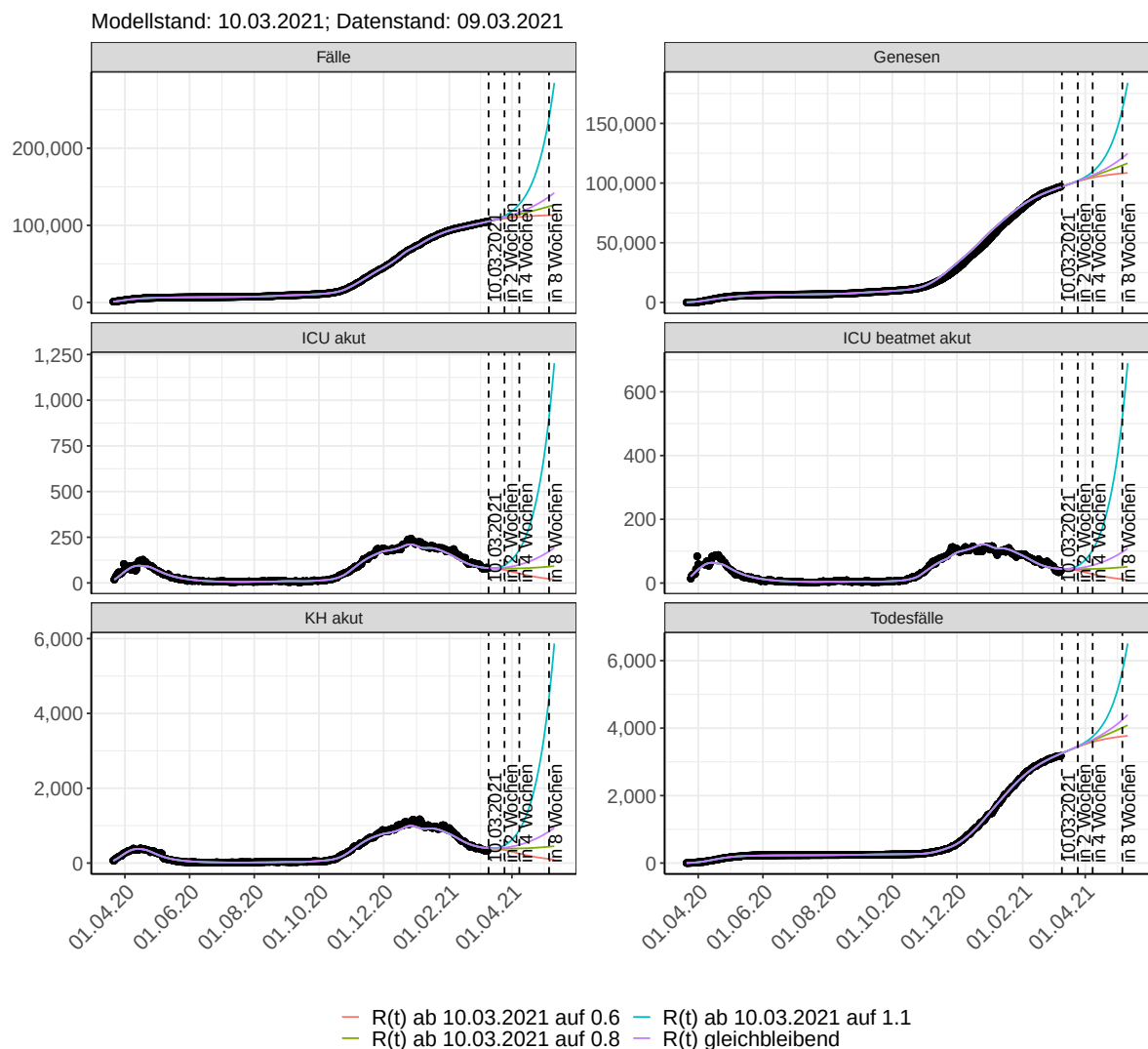
Abbildung 156: Lineare Darstellung der Modellvorhersage (Fallzahlen, Genesen, ICU Beatmet, ICU Betten, KH Betten, Todesfälle) für Rheinland-Pfalz unter Annahme verschiedener Szenarien ab dem 10.03.2021. Punkte: gemeldete Fallzahlen; Linien: Modellvorhersage.
