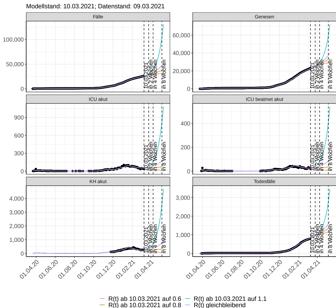
Abbildung 115: Lineare Darstellung der Modellvorhersage (Fallzahlen, Genesen, ICU Beatmet, ICU Betten, KH Betten, Todesfälle) für Mecklenburg-Vorpommern unter Annahme verschiedener Szenarien ab dem 10.03.2021. Punkte: gemeldete Fallzahlen; Linien: Modellvorhersage.
