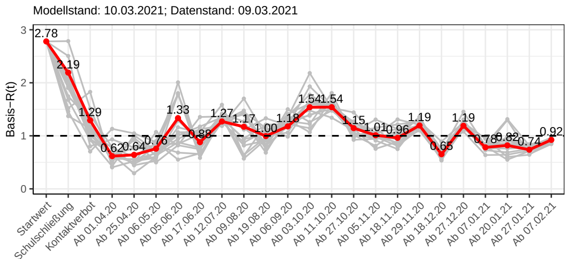
Abbildung 222: Basis- R(t) Werte vor und nach den NPIs für Deutschland
