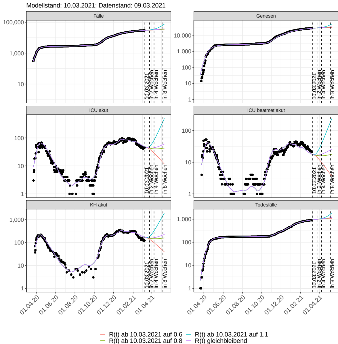
Abbildung 170: Halblogarithmische Darstellung der Modellvorhersage (Fallzahlen, Genesen, ICU Beatmet, ICU Betten, KH Betten, Todesfälle) für Saarland unter Annahme verschiedener Szenarien nach dem 10.03.2021. Punkte: gemeldete Fallzahlen; Linien: Modellvorhersage.
