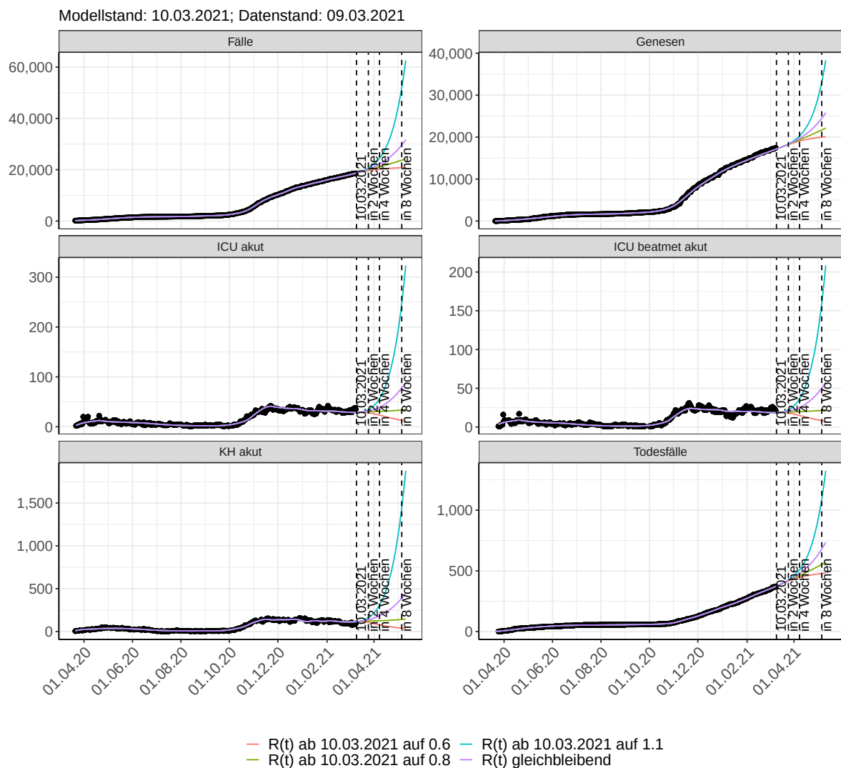
Abbildung 80: Lineare Darstellung der Modellvorhersage (Fallzahlen, Genesen, ICU Beatmet, ICU Betten, KH Betten, Todesfälle) für Bremen unter Annahme verschiedener Szenarien ab dem 10.03.2021. Punkte: gemeldete Fallzahlen; Linien: Modellvorhersage.
