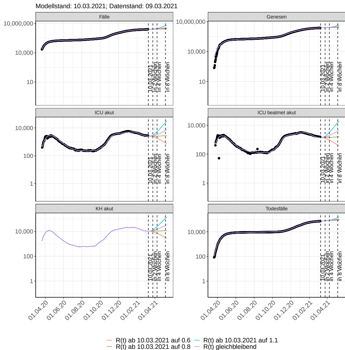
Abbildung 226: Halblogarithmische Darstellung der Modellvorhersage (Fallzahlen, Genesen, ICU Beatmet, ICU Betten, KH Betten, Todesfälle) für Deutschland unter Annahme verschiedener Szenarien ab dem 10.03.2021. Punkte: gemeldete Fallzahlen; Linien: Modellvorhersage.
