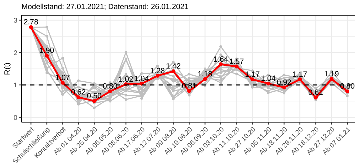
Abbildung 152: R(t) Werte vor und nach den NPIs für Rheinland-Pfalz
