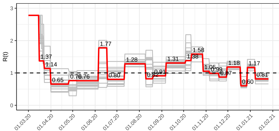
Abbildung 138: R(t) Werte über die Zeit für Nordrhein-Westfalen
