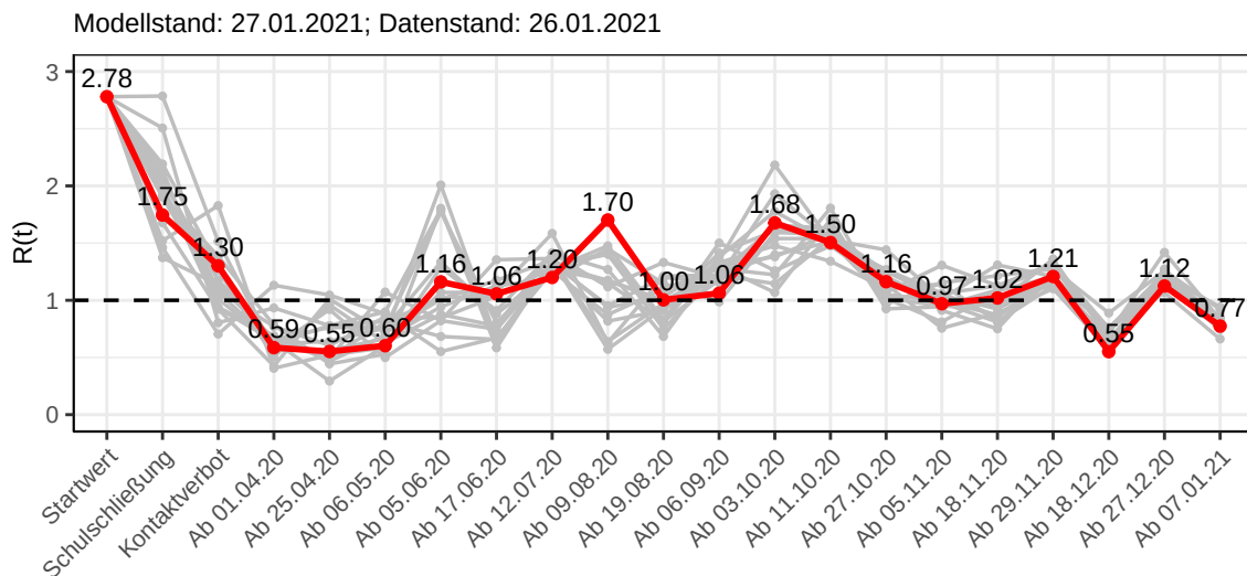
Abbildung 20: R(t) Werte vor und nach den NPIs für Baden-Württemberg
