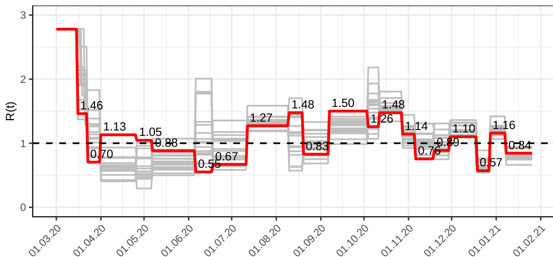
Abbildung 77: R(t) Werte über die Zeit für Bremen
