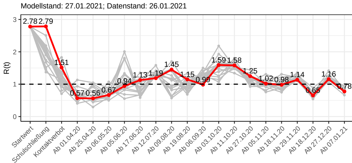
Abbildung 35: R(t) Werte vor und nach den NPIs für Bayern
