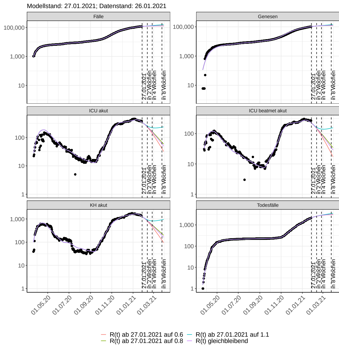
Abbildung 59: Halblogarithmische Darstellung der Modellvorhersage (Fallzahlen, Genesen, ICU Beatmet, ICU Betten, KH Betten, Todesfälle) für Berlin unter Annahme verschiedener Szenarien nach dem 27.01.2021. Punkte: gemeldete Fallzahlen; Linien: Modellvorhersage.
