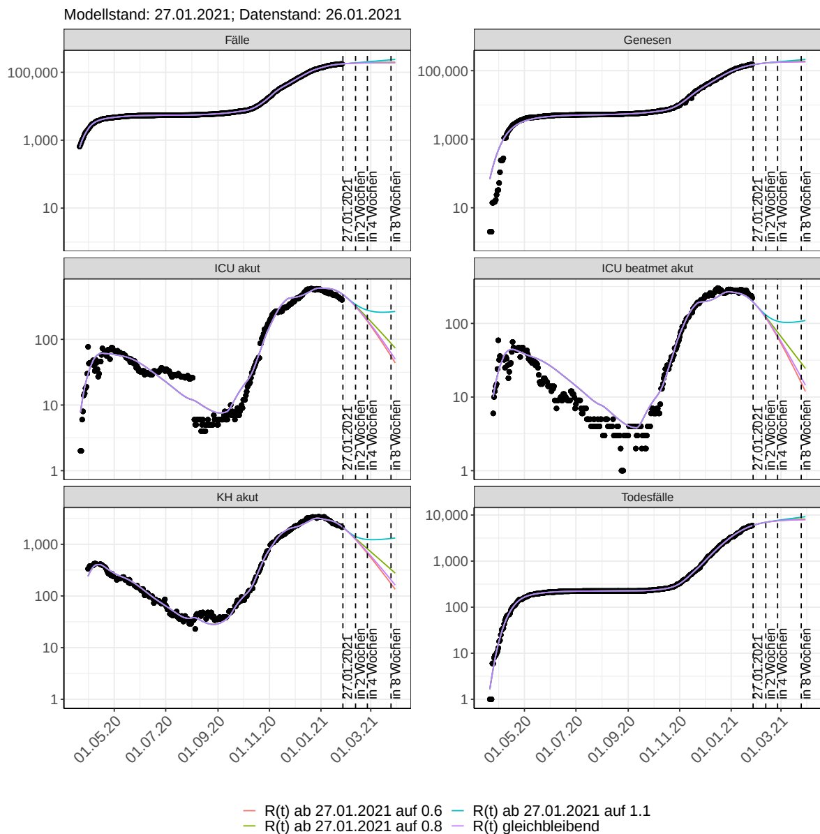
Abbildung 181: Halblogarithmische Darstellung der Modellvorhersage (Fallzahlen, Genesen, ICU Beatmet, ICU Betten, KH Betten, Todesfälle) für Sachsen unter Annahme verschiedener Szenarien nach dem 27.01.2021. Punkte: gemeldete Fallzahlen; Linien: Modellvorhersage.
