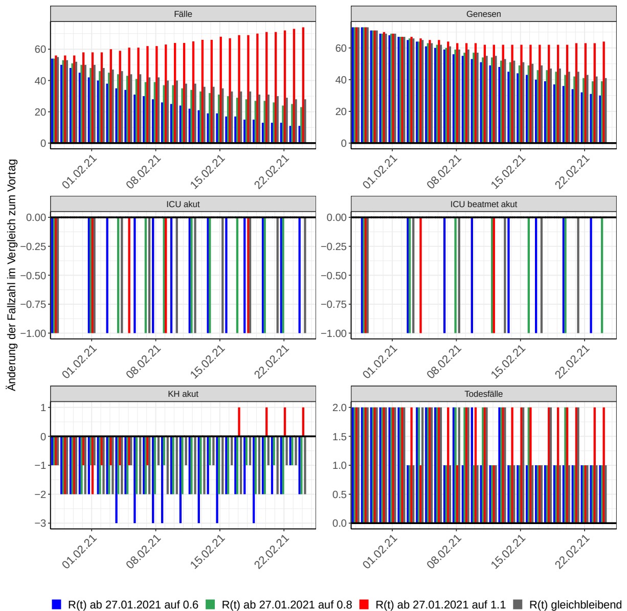
Abbildung 82: Simulation täglich neu auftretender Fälle für die nächsten 4 Wochen - Bremen
