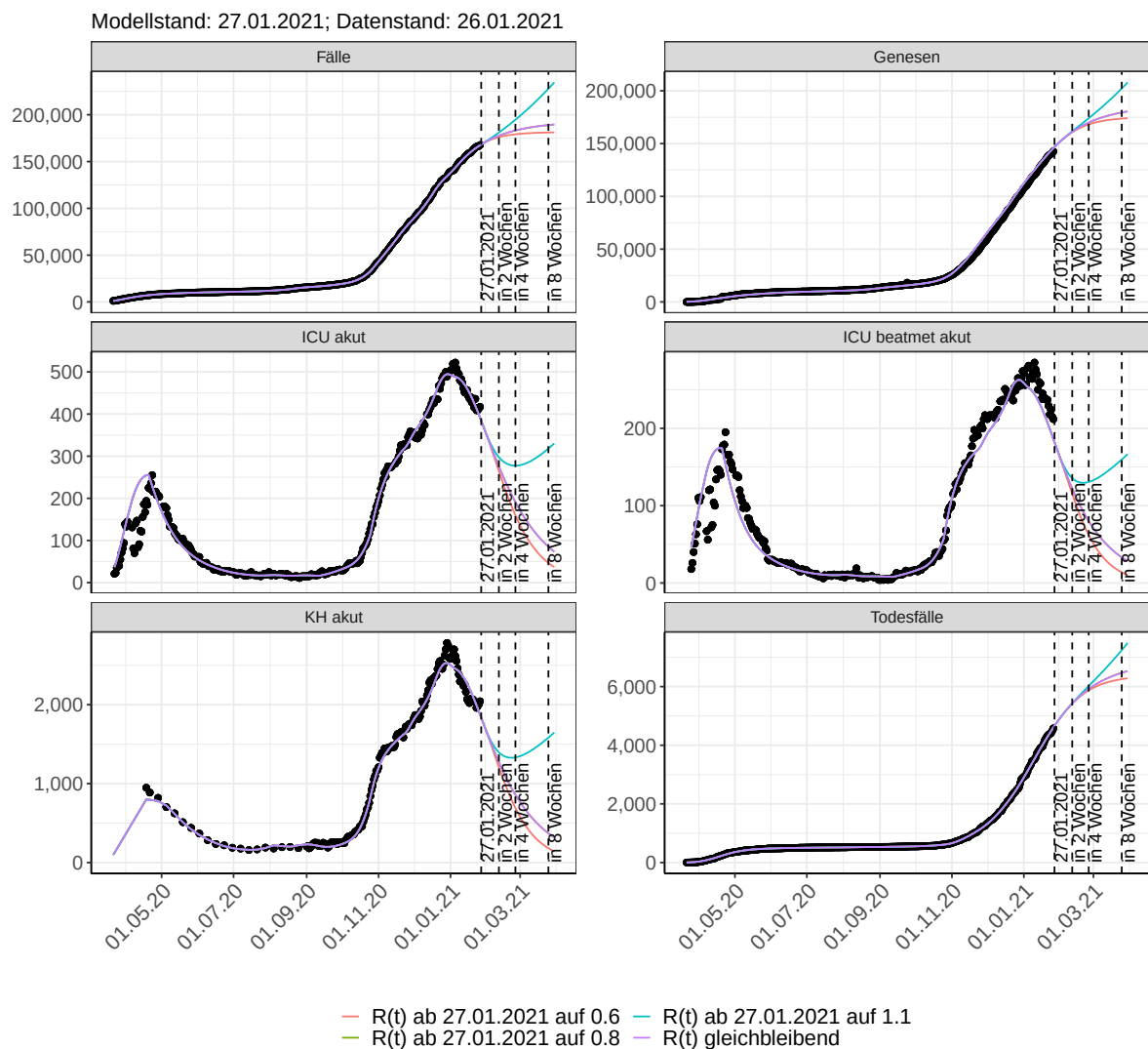
Abbildung 102: Lineare Darstellung der Modellvorhersage (Fallzahlen, Genesen, ICU Beatmet, ICU Betten, KH Betten, Todesfälle) für Hessen unter Annahme verschiedener Szenarien ab dem 27.01.2021. Punkte: gemeldete Fallzahlen; Linien: Modellvorhersage.
