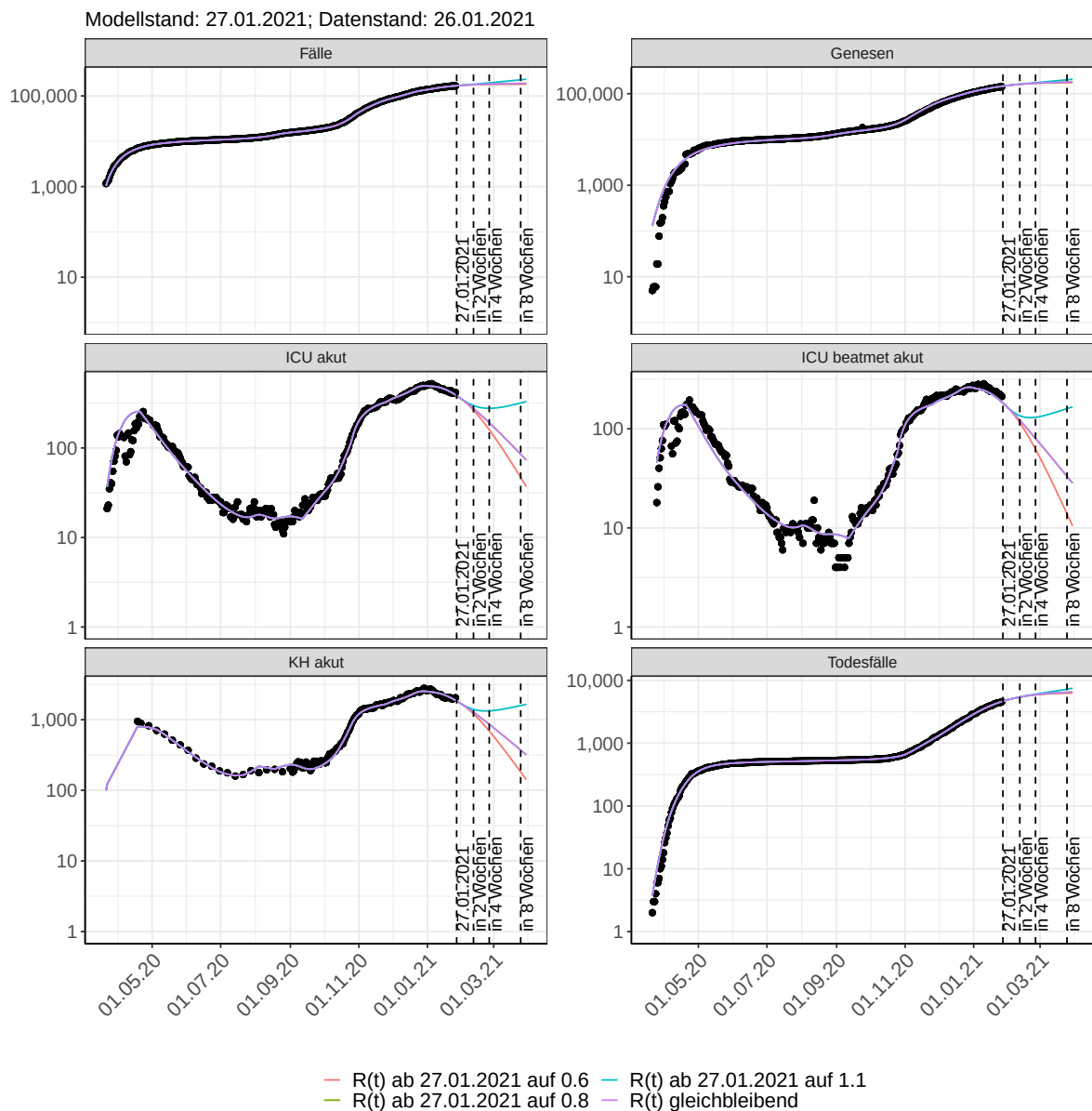
Abbildung 103: Halblogarithmische Darstellung der Modellvorhersage (Fallzahlen, Genesen, ICU Beatmet, ICU Betten, KH Betten, Todesfälle) für Hessen unter Annahme verschiedener Szenarien nach dem 27.01.2021. Punkte: gemeldete Fallzahlen; Linien: Modellvorhersage.
