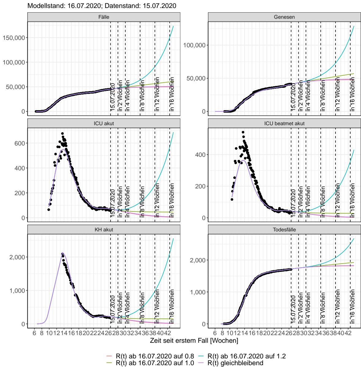
Abbildung 118: Lineare Darstellung der Modellvorhersage (Fallzahlen, Genesen, ICU Beatmet, ICU Betten, KH Betten, Todesfälle) für Nordrhein-Westfalen unter Annahme verschiedener Szenarien ab dem 16.07.2020. Punkte: gemeldete Fallzahlen; Linien: Modellvorhersage.
