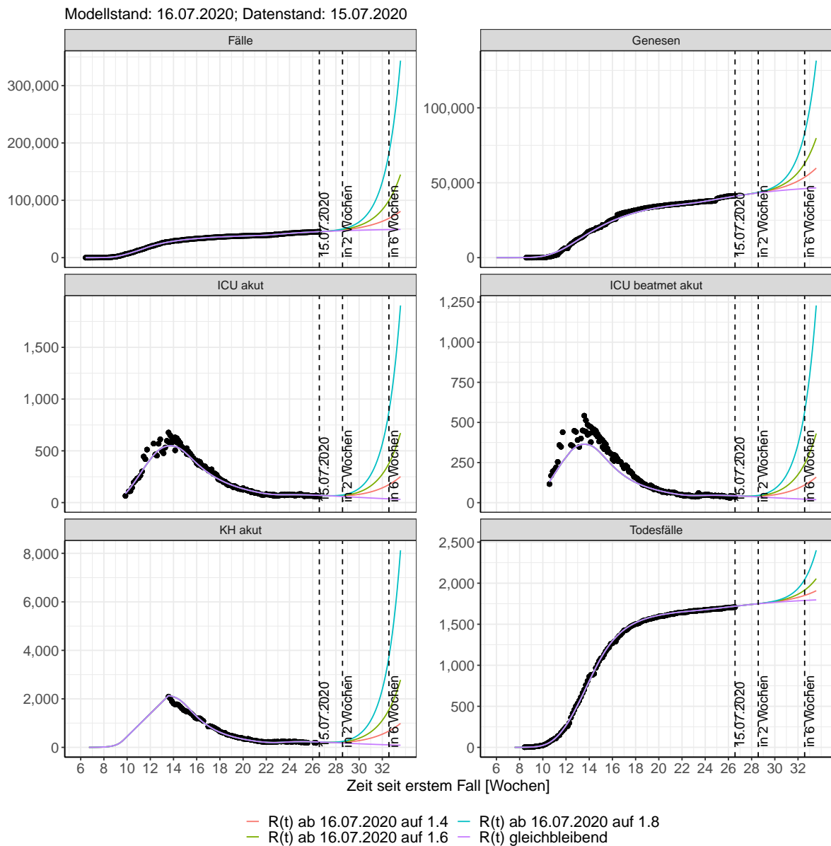
Abbildung 116: Lineare Darstellung der Modellvorhersage (Fallzahlen, Genesen, ICU Beatmet, ICU Betten, KH Betten, Todesfälle) für Nordrhein-Westfalen unter Annahme verschiedener Szenarien ab dem 16.07.2020. Punkte: gemeldete Fallzahlen; Linien: Modellvorhersage.
