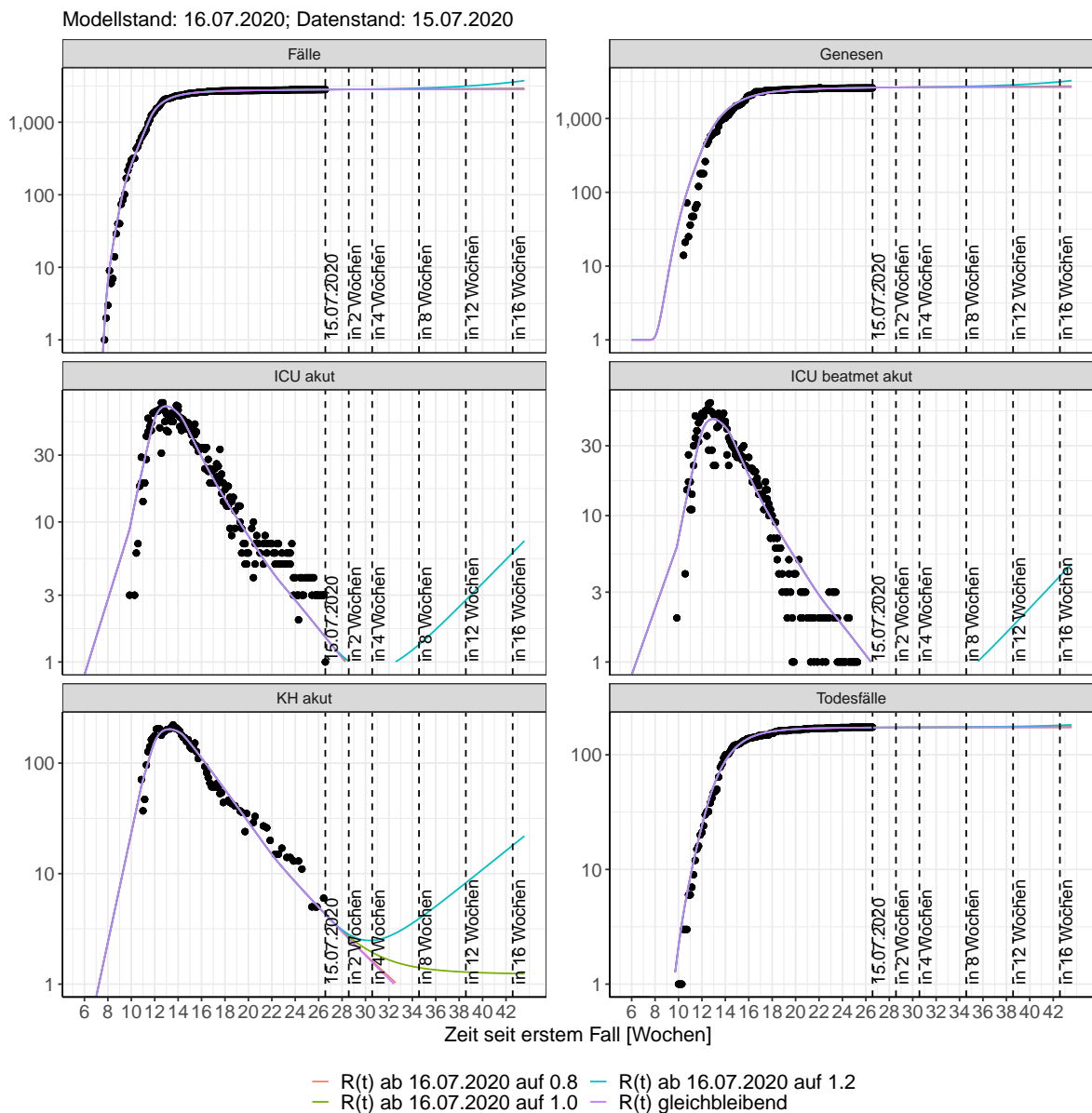
Abbildung 141: Halblogarithmische Darstellung der Modellvorhersage (Fallzahlen, Genesen, ICU Beatmet, ICU Betten, KH Betten, Todesfälle) für Saarland unter Annahme verschiedener Szenarien nach dem 16.07.2020. Punkte: gemeldete Fallzahlen; Linien: Modellvorhersage.
