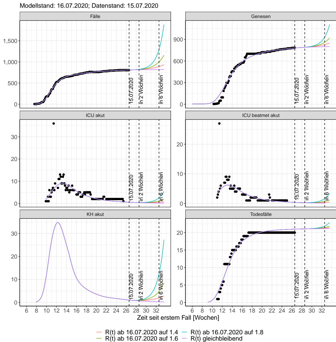
Abbildung 94: Lineare Darstellung der Modellvorhersage (Fallzahlen, Genesen, ICU Beatmet, ICU Betten, KH Betten, Todesfälle) für Mecklenburg-Vorpommern unter Annahme verschiedener Szenarien ab dem 16.07.2020. Punkte: gemeldete Fallzahlen; Linien: Modellvorhersage.
