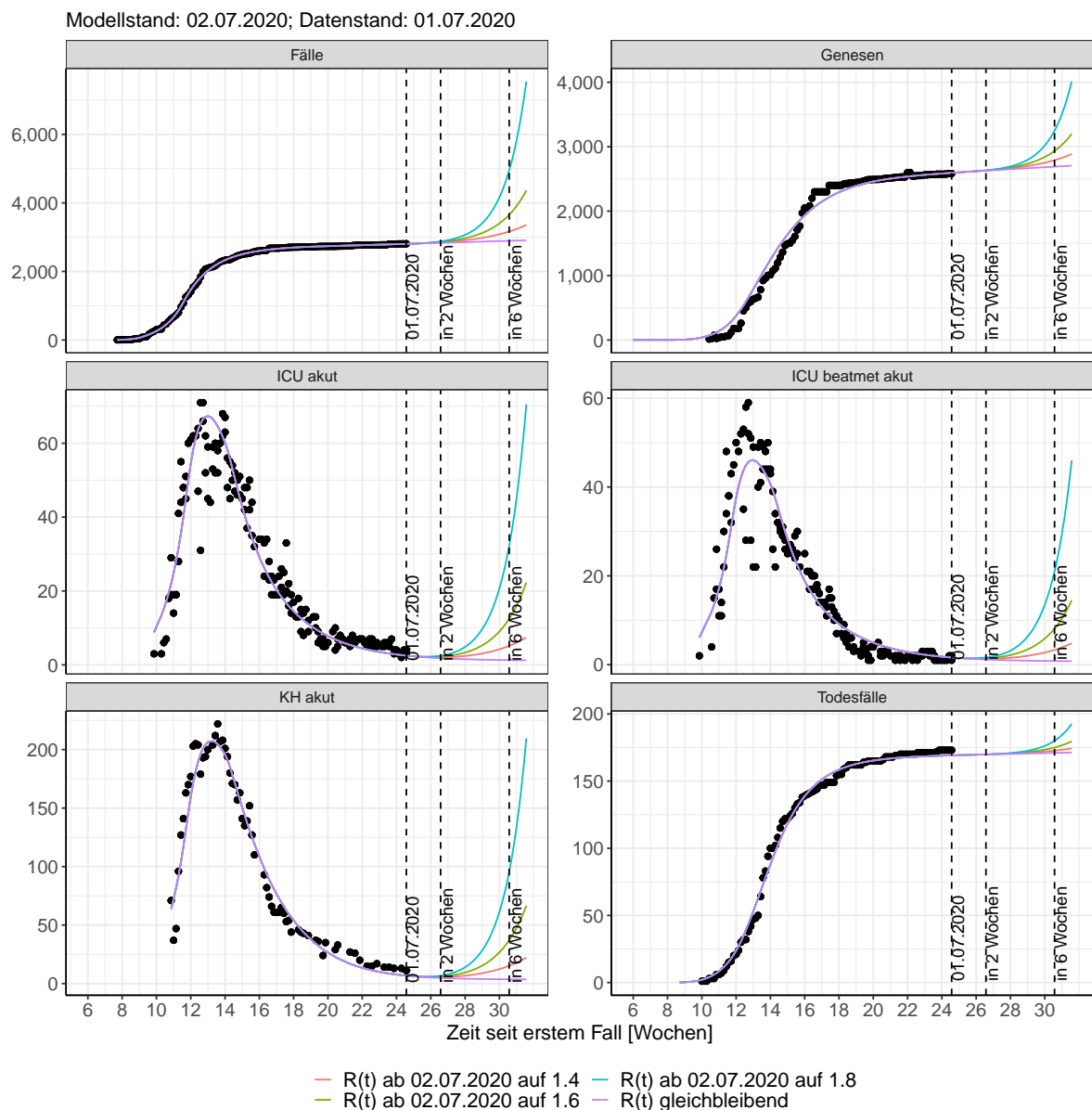
Abbildung 138: Lineare Darstellung der Modellvorhersage (Fallzahlen, Genesen, ICU Beatmet, ICU Betten, KH Betten, Todesfälle) für Saarland unter Annahme verschiedener Szenarien ab dem 02.07.2020. Punkte: gemeldete Fallzahlen; Linien: Modellvorhersage.
