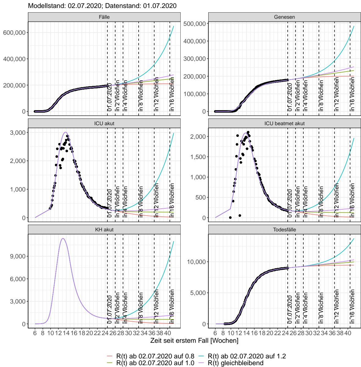
Abbildung 195: Lineare Darstellung der Modellvorhersage (Fallzahlen, Genesen, ICU Beatmet, ICU Betten, KH Betten, Todesfälle) für Deutschland unter Annahme verschiedener Szenarien ab dem 02.07.2020. Punkte: gemeldete Fallzahlen;Linien: Modellvorhersage.
