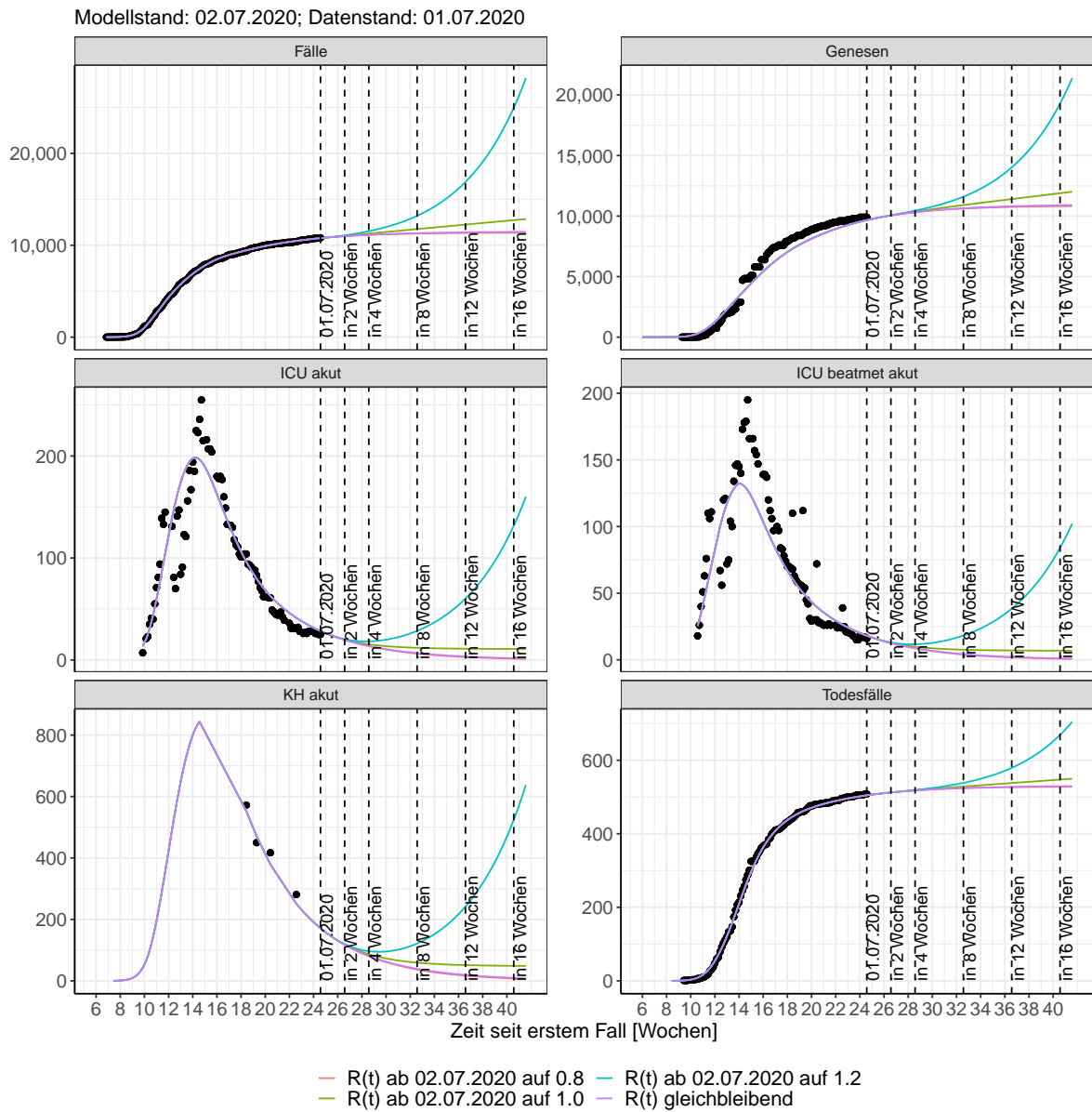
Abbildung 85: Lineare Darstellung der Modellvorhersage (Fallzahlen, Genesen, ICU Beatmet, ICU Betten, KH Betten, Todesfälle) für Hessen unter Annahme verschiedener Szenarien ab dem 02.07.2020. Punkte: gemeldete Fallzahlen; Linien: Modellvorhersage.
