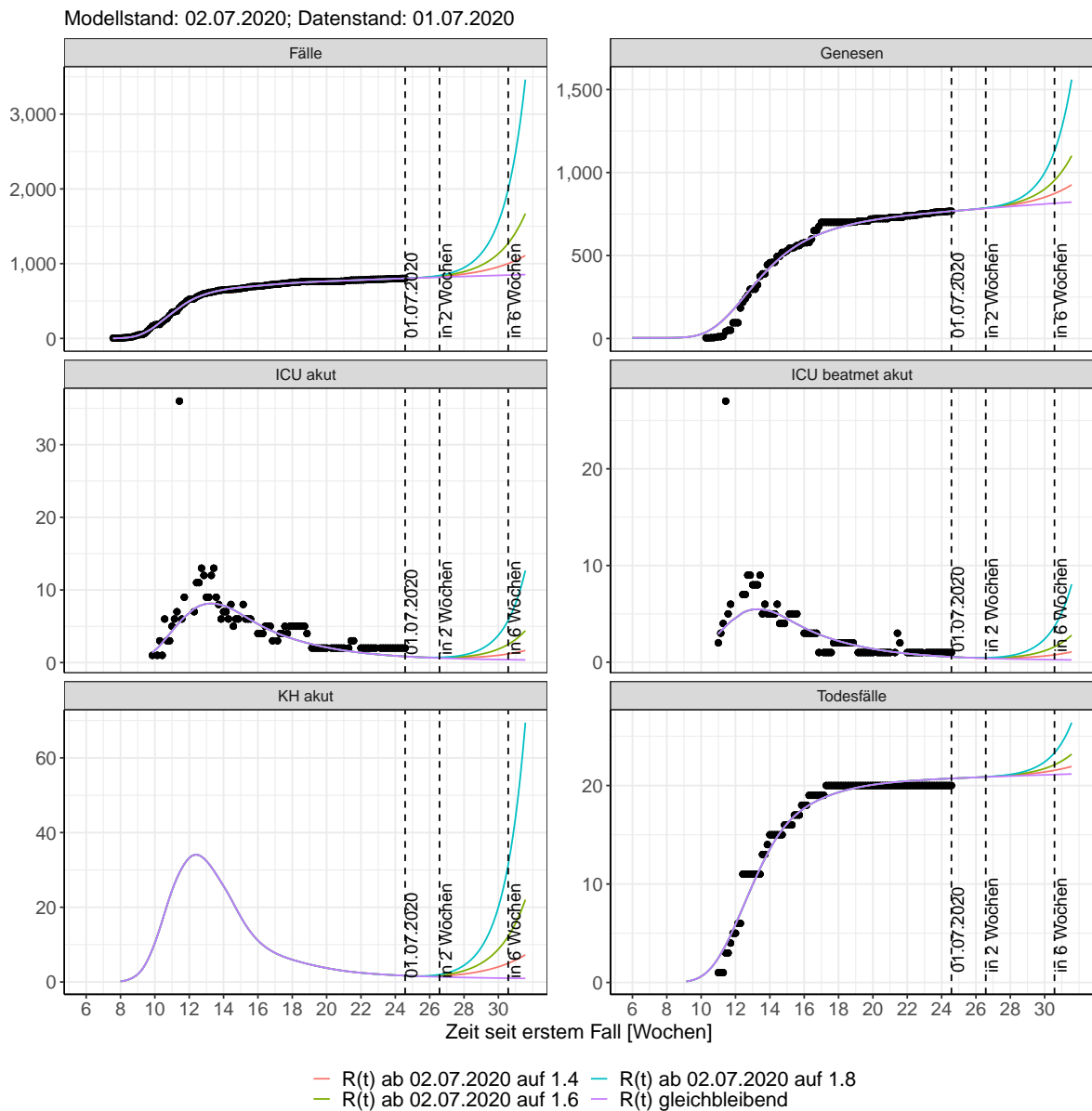
Abbildung 94: Lineare Darstellung der Modellvorhersage (Fallzahlen, Genesen, ICU Beatmet, ICU Betten, KH Betten, Todesfälle) für Mecklenburg-Vorpommern unter Annahme verschiedener Szenarien ab dem 02.07.2020. Punkte: gemeldete Fallzahlen; Linien: Modellvorhersage.
