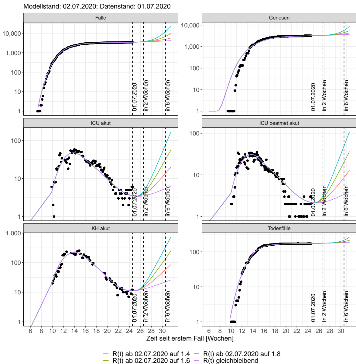
Abbildung 51: Halblogarithmische Darstellung der Modellvorhersage (Fallzahlen, Genesen, ICU Beatmet, ICU Betten, KH Betten, Todesfälle) für Brandenburg unter Annahme verschiedener Szenarien nach dem 02.07.2020. Punkte: gemeldete Fallzahlen; Linien: Modellvorhersage.
