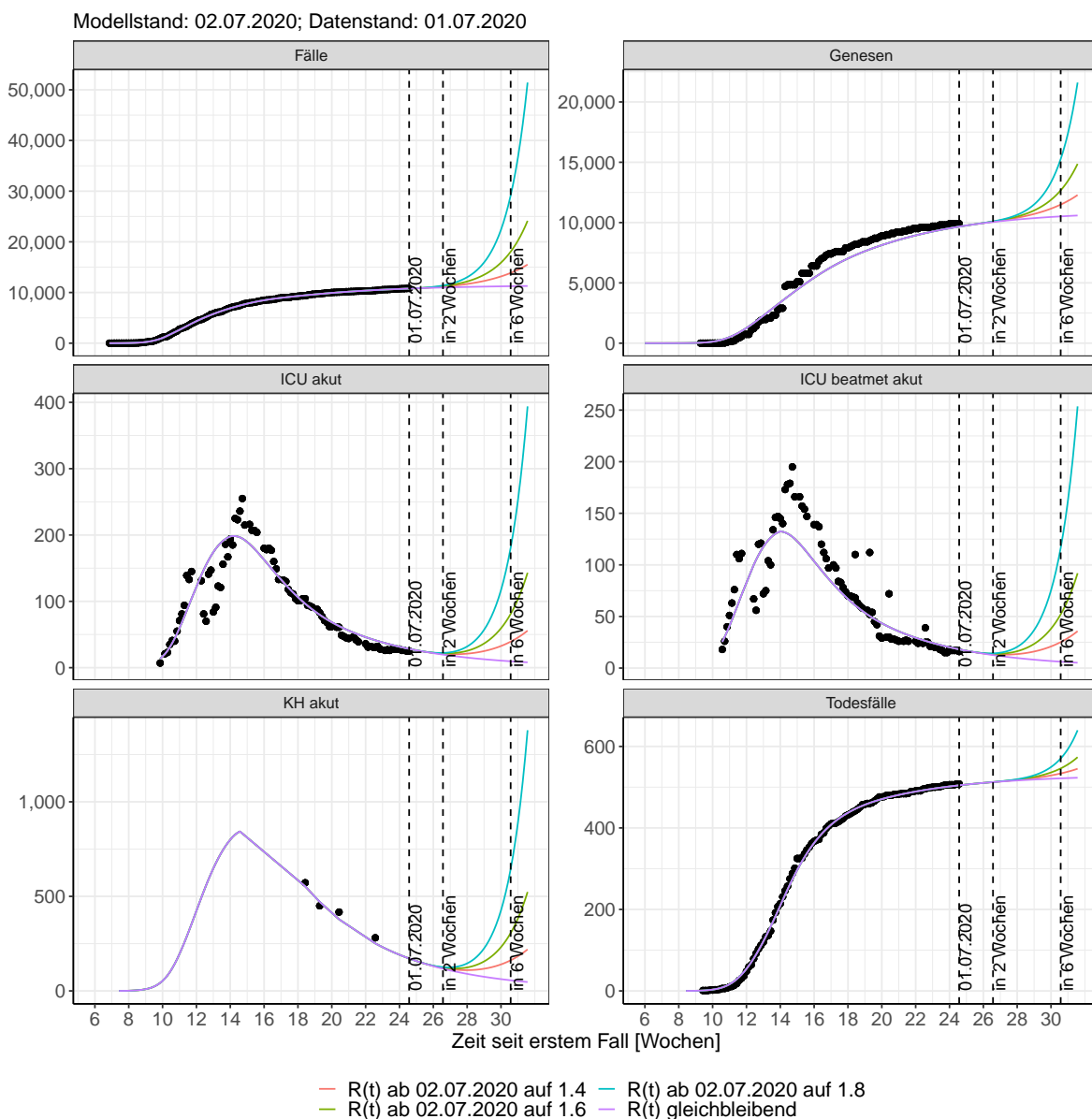
Abbildung 83: Lineare Darstellung der Modellvorhersage (Fallzahlen, Genesen, ICU Beatmet, ICU Betten, KH Betten, Todesfälle) für Hessen unter Annahme verschiedener Szenarien ab dem 02.07.2020. Punkte: gemeldete Fallzahlen; Linien: Modellvorhersage.
