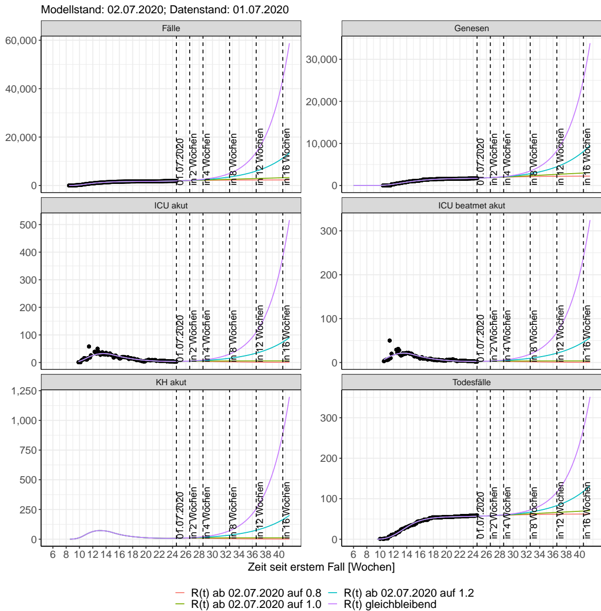
Abbildung 162: Lineare Darstellung der Modellvorhersage (Fallzahlen, Genesen, ICU Beatmet, ICU Betten, KH Betten, Todesfälle) für Sachsen-Anhalt unter Annahme verschiedener Szenarien ab dem 02.07.2020. Punkte: gemeldete Fallzahlen; Linien: Modellvorhersage.
