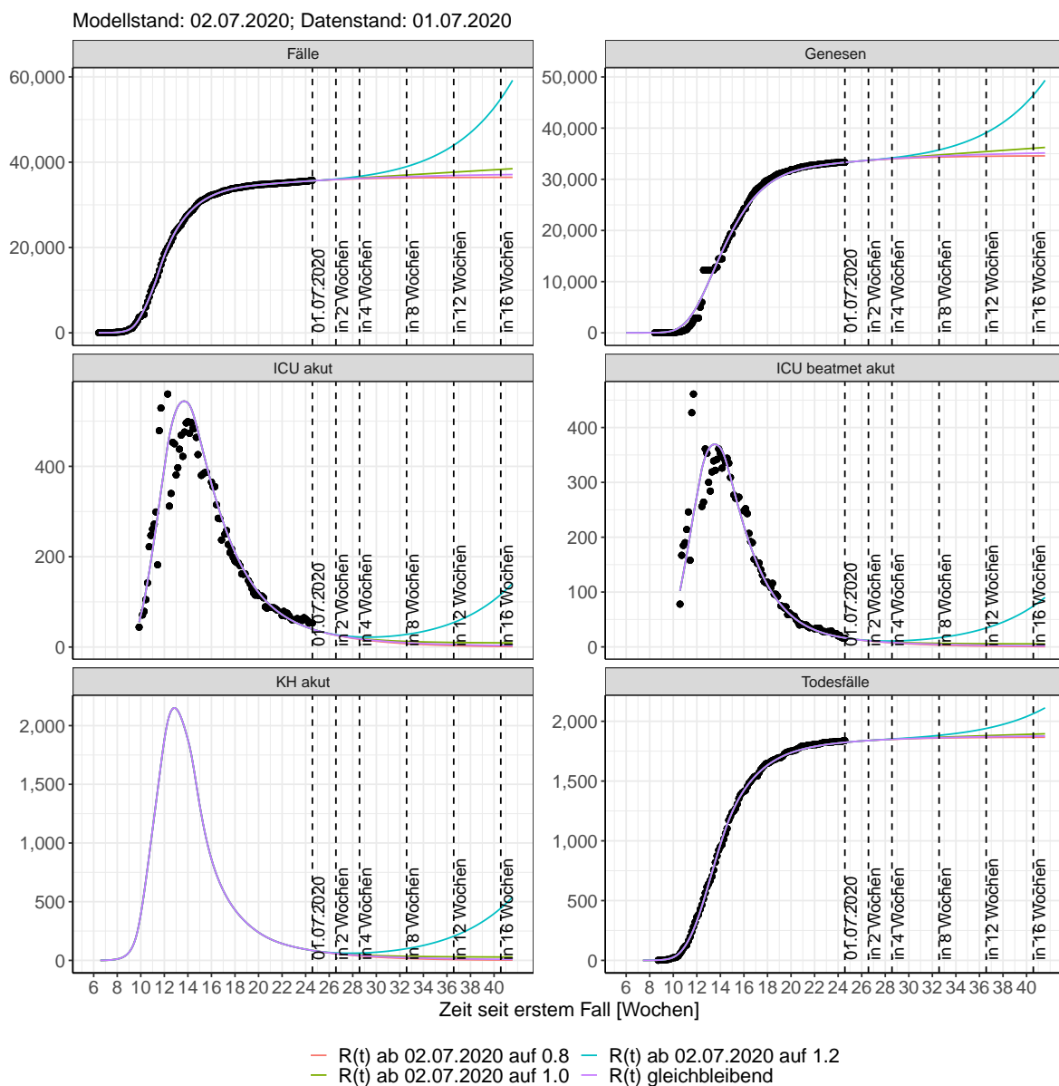
Abbildung 19: Lineare Darstellung der Modellvorhersage (Fallzahlen, Genesen, ICU Beatmet, ICU Betten, KH Betten, Todesfälle) für Baden-Württemberg unter Annahme verschiedener Szenarien ab dem 02.07.2020. Punkte: gemeldete Fallzahlen; Linien: Modellvorhersage.
