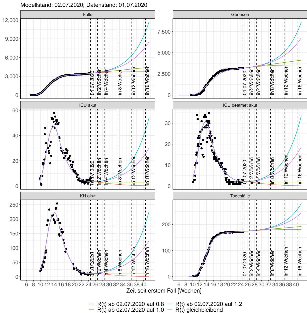
Abbildung 52: Lineare Darstellung der Modellvorhersage (Fallzahlen, Genesen, ICU Beatmet, ICU Betten, KH Betten, Todesfälle) für Brandenburg unter Annahme verschiedener Szenarien ab dem 02.07.2020. Punkte: gemeldete Fallzahlen; Linien: Modellvorhersage.
