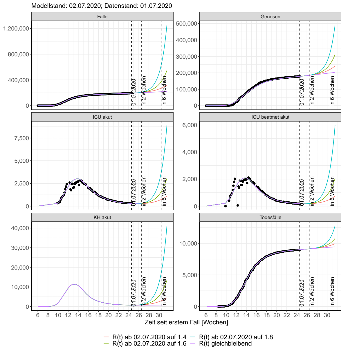
Abbildung 193: Lineare Darstellung der Modellvorhersage (Fallzahlen, Genesen, ICU Beatmet, ICU Betten, KH Betten, Todesfälle) für Deutschland unter Annahme verschiedener Szenarien ab dem 02.07.2020. Punkte: gemeldete Fallzahlen; Linien: Modellvorhersage.
