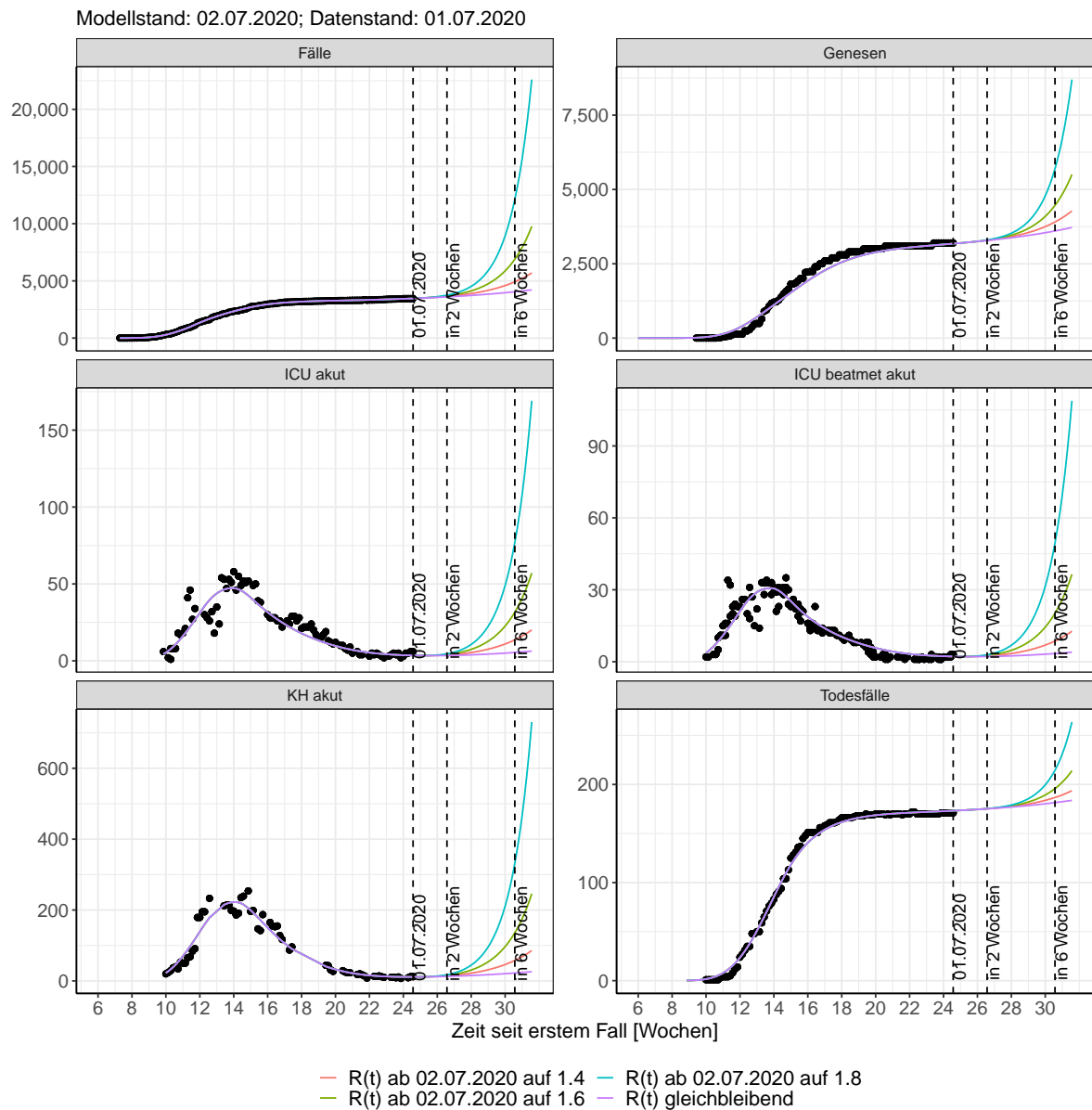
Abbildung 50: Lineare Darstellung der Modellvorhersage (Fallzahlen, Genesen, ICU Beatmet, ICU Betten, KH Betten, Todesfälle) für Brandenburg unter Annahme verschiedener Szenarien ab dem 02.07.2020. Punkte: gemeldete Fallzahlen; Linien: Modellvorhersage.
