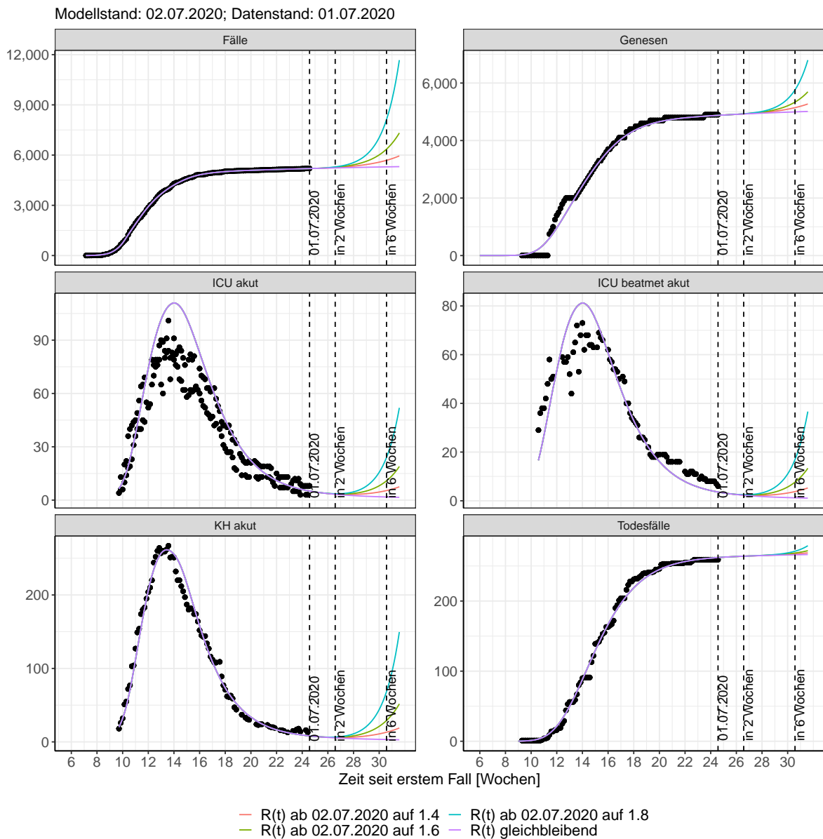
Abbildung 72: Lineare Darstellung der Modellvorhersage (Fallzahlen, Genesen, ICU Beatmet, ICU Betten, KH Betten, Todesfälle) für Hamburg unter Annahme verschiedener Szenarien ab dem 02.07.2020. Punkte: gemeldete Fallzahlen; Linien: Modellvorhersage.
