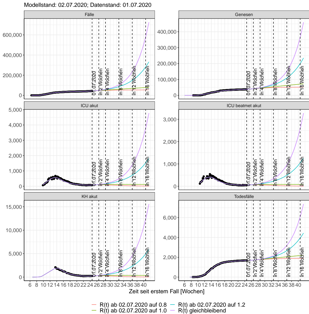
Abbildung 118: Lineare Darstellung der Modellvorhersage (Fallzahlen, Genesen, ICU Beatmet, ICU Betten, KH Betten, Todesfälle) für Nordrhein-Westfalen unter Annahme verschiedener Szenarien ab dem 02.07.2020. Punkte: gemeldete Fallzahlen; Linien: Modellvorhersage.
