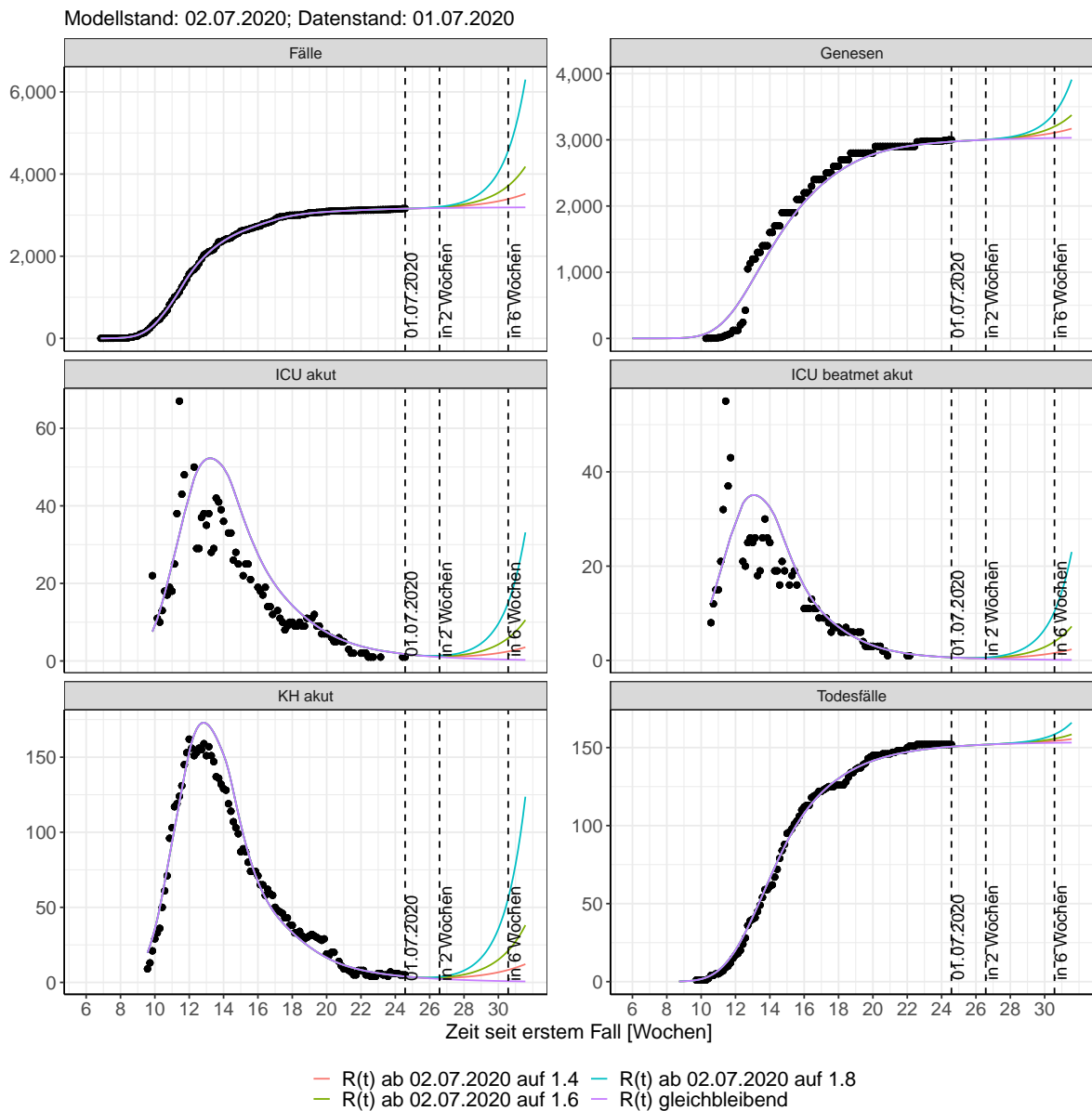
Abbildung 171: Lineare Darstellung der Modellvorhersage (Fallzahlen, Genesen, ICU Beatmet, ICU Betten, KH Betten, Todesfälle) für Schleswig-Holstein unter Annahme verschiedener Szenarien ab dem 02.07.2020. Punkte: gemeldete Fallzahlen; Linien: Modellvorhersage.
