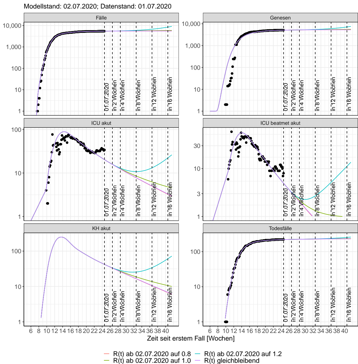
Abbildung 152: Halblogarithmische Darstellung der Modellvorhersage (Fallzahlen, Genesen, ICU Beatmet, ICU Betten, KH Betten, Todesfälle) für Sachsen unter Annahme verschiedener Szenarien nach dem 02.07.2020. Punkte: gemeldete Fallzahlen; Linien: Modellvorhersage.
