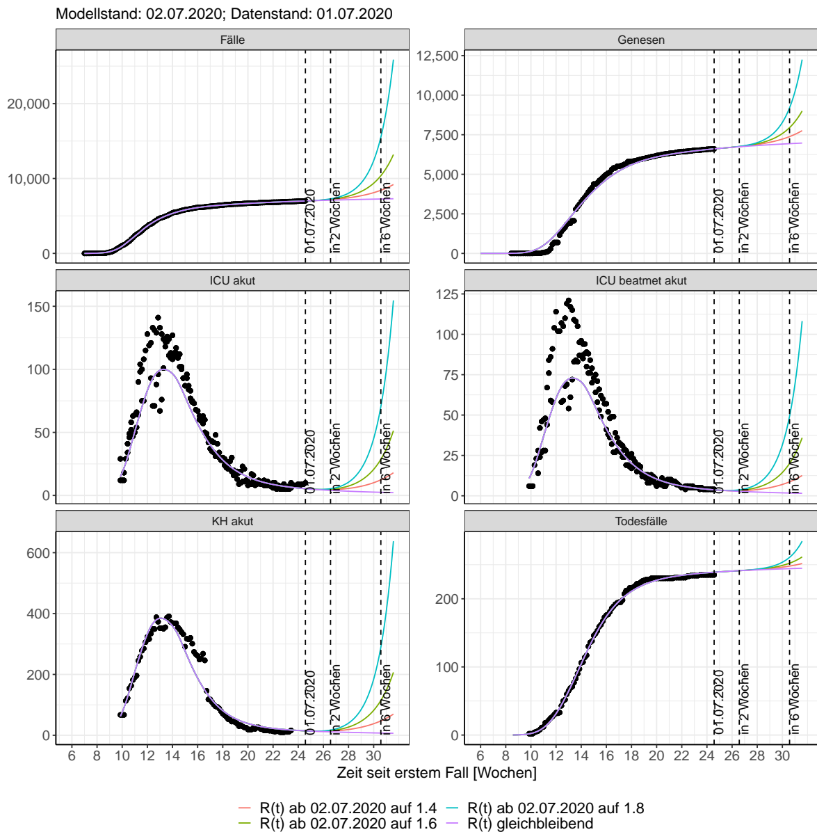
Abbildung 127: Lineare Darstellung der Modellvorhersage (Fallzahlen, Genesen, ICU Beatmet, ICU Betten, KH Betten, Todesfälle) für Rheinland-Pfalz unter Annahme verschiedener Szenarien ab dem 02.07.2020. Punkte: gemeldete Fallzahlen; Linien: Modellvorhersage.
