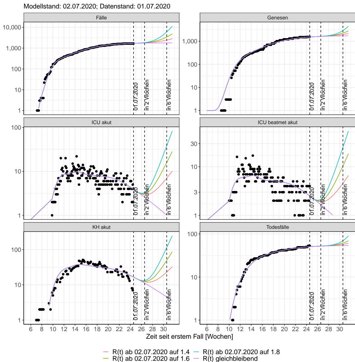
Abbildung 62: Halblogarithmische Darstellung der Modellvorhersage (Fallzahlen, Genesen, ICU Beatmet, ICU Betten, KH Betten, Todesfälle) für Bremen unter Annahme verschiedener Szenarien nach dem 02.07.2020. Punkte: gemeldete Fallzahlen; Linien: Modellvorhersage.
