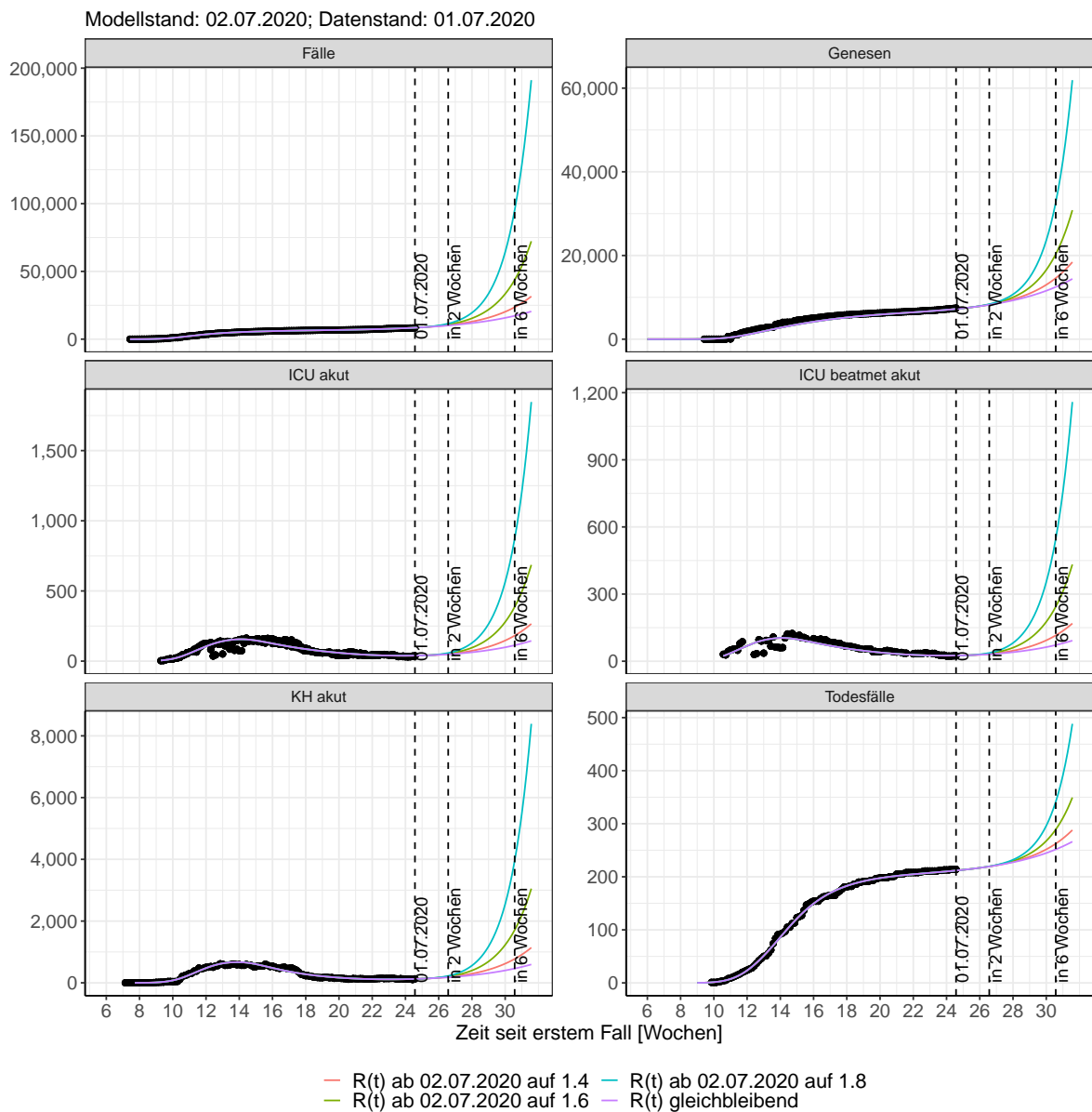
Abbildung 39: Lineare Darstellung der Modellvorhersage (Fallzahlen, Genesen, ICU Beatmet, ICU Betten, KH Betten, Todesfälle) für Berlin unter Annahme verschiedener Szenarien ab dem 02.07.2020. Punkte: gemeldete Fallzahlen; Linien: Modellvorhersage.
