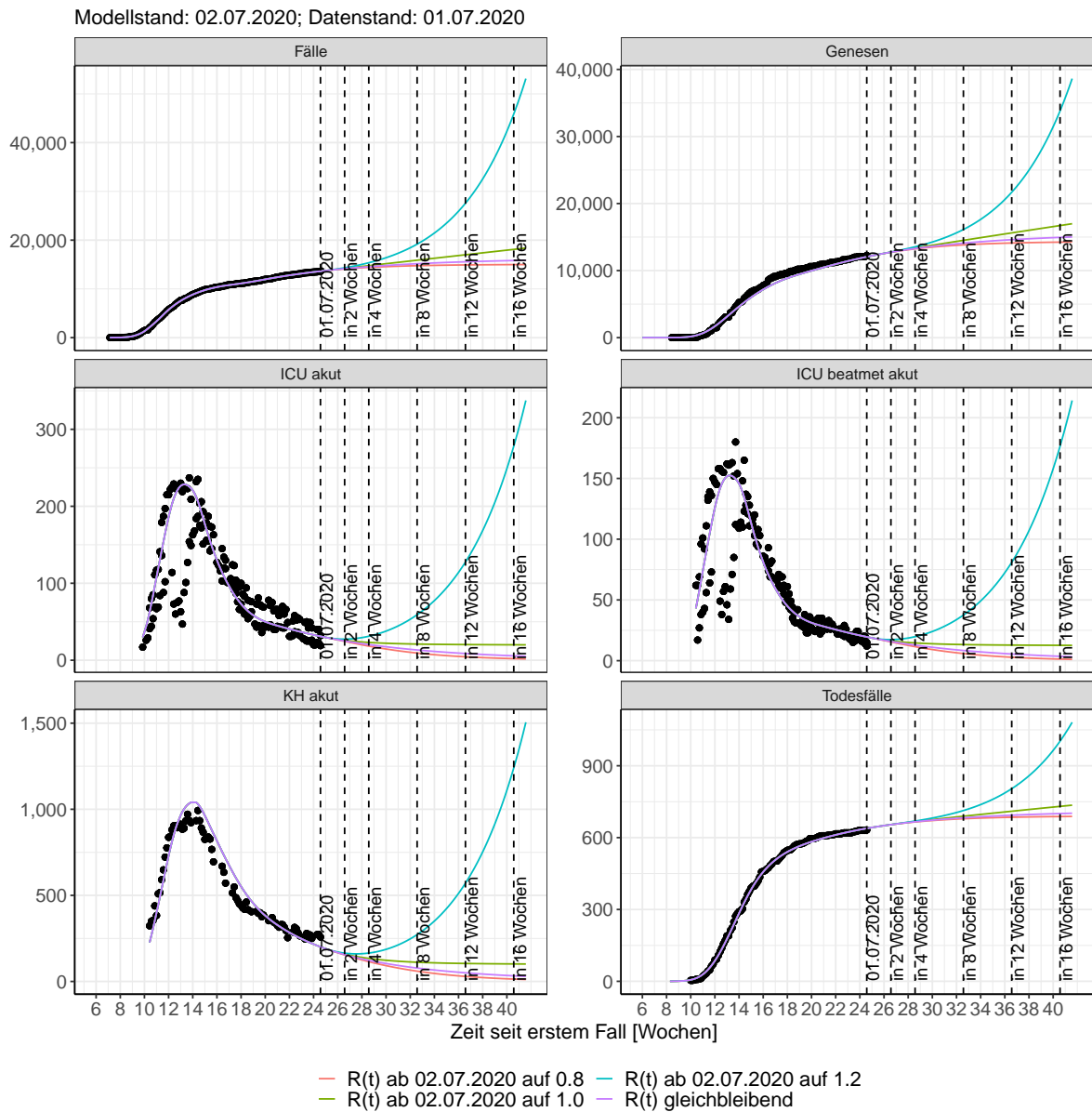
Abbildung 107: Lineare Darstellung der Modellvorhersage (Fallzahlen, Genesen, ICU Beatmet, ICU Betten, KH Betten, Todesfälle) für Niedersachsen unter Annahme verschiedener Szenarien ab dem 02.07.2020. Punkte: gemeldete Fallzahlen; Linien: Modellvorhersage.
