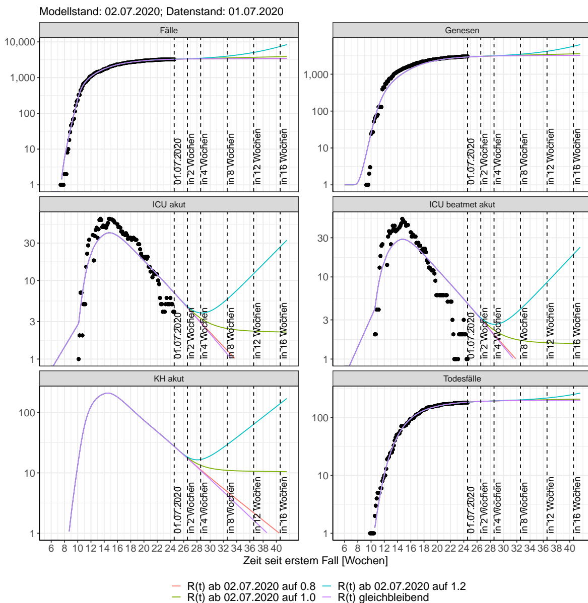
Abbildung 185: Halblogarithmische Darstellung der Modellvorhersage (Fallzahlen, Genesen, ICU Beatmet, ICU Betten, KH Betten, Todesfälle) für Thüringen unter Annahme verschiedener Szenarien nach dem 02.07.2020. Punkte: gemeldete Fallzahlen; Linien: Modellvorhersage.
