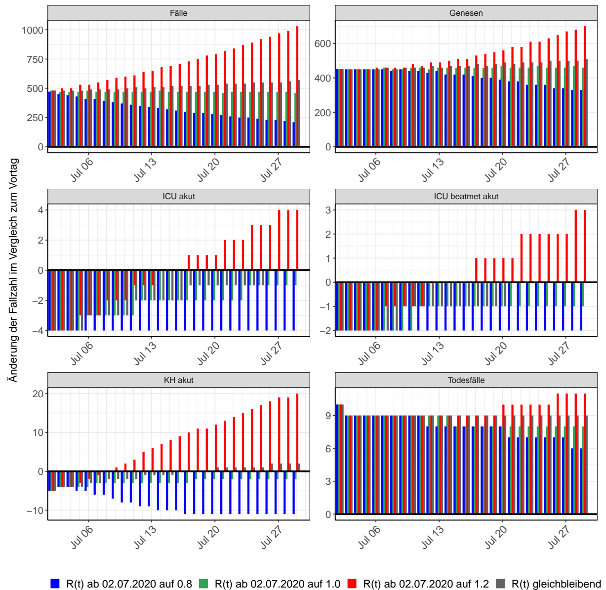
Abbildung 197: Simulation täglich neu auftretender Fälle für die nächsten 4 Wochen - Deutschland
