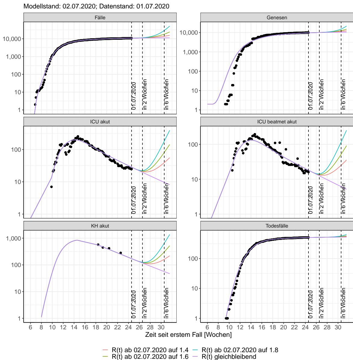
Abbildung 84: Halblogarithmische Darstellung der Modellvorhersage (Fallzahlen, Genesen, ICU Beatmet, ICU Betten, KH Betten, Todesfälle) für Hessen unter Annahme verschiedener Szenarien nach dem 02.07.2020. Punkte: gemeldete Fallzahlen; Linien: Modellvorhersage.
