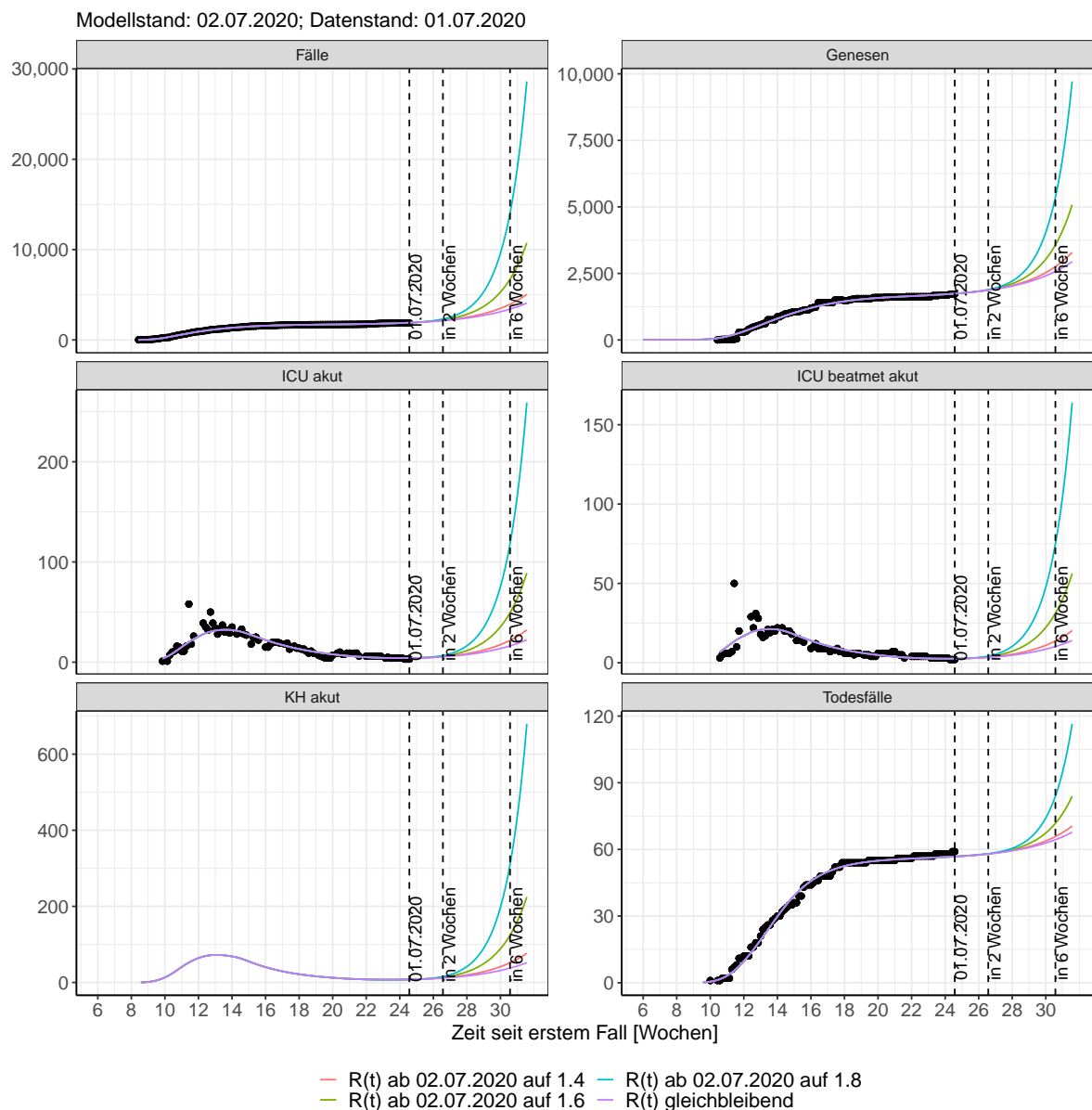
Abbildung 160: Lineare Darstellung der Modellvorhersage (Fallzahlen, Genesen, ICU Beatmet, ICU Betten, KH Betten, Todesfälle) für Sachsen-Anhalt unter Annahme verschiedener Szenarien ab dem 02.07.2020. Punkte: gemeldete Fallzahlen; Linien: Modellvorhersage.
