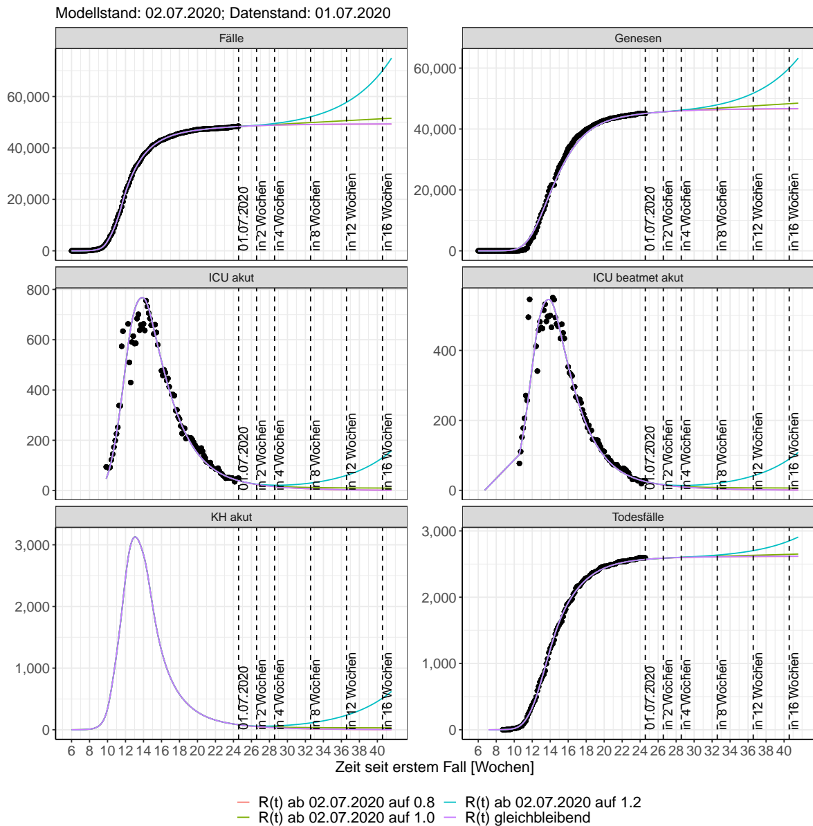
Abbildung 30: Lineare Darstellung der Modellvorhersage (Fallzahlen, Genesen, ICU Beatmet, ICU Betten, KH Betten, Todesfälle) für Bayern unter Annahme verschiedener Szenarien ab dem 02.07.2020. Punkte: gemeldete Fallzahlen; Linien: Modellvorhersage.
