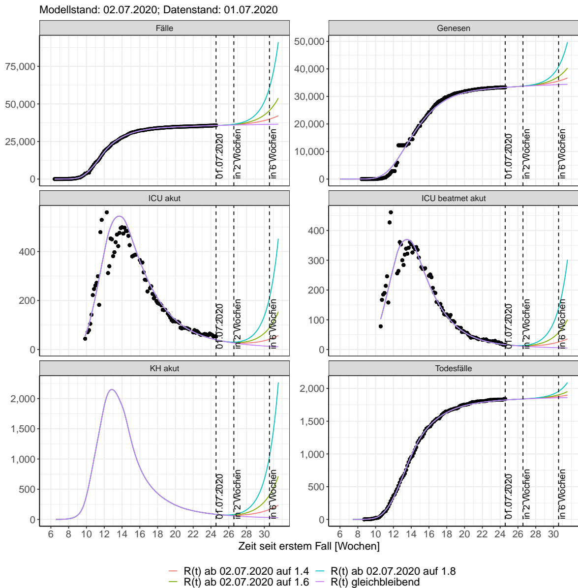
Abbildung 17: Lineare Darstellung der Modellvorhersage (Fallzahlen, Genesen, ICU Beatmet, ICU Betten, KH Betten, Todesfälle) für Baden-Württemberg unter Annahme verschiedener Szenarien ab dem 02.07.2020. Punkte: gemeldete Fallzahlen; Linien: Modellvorhersage.
