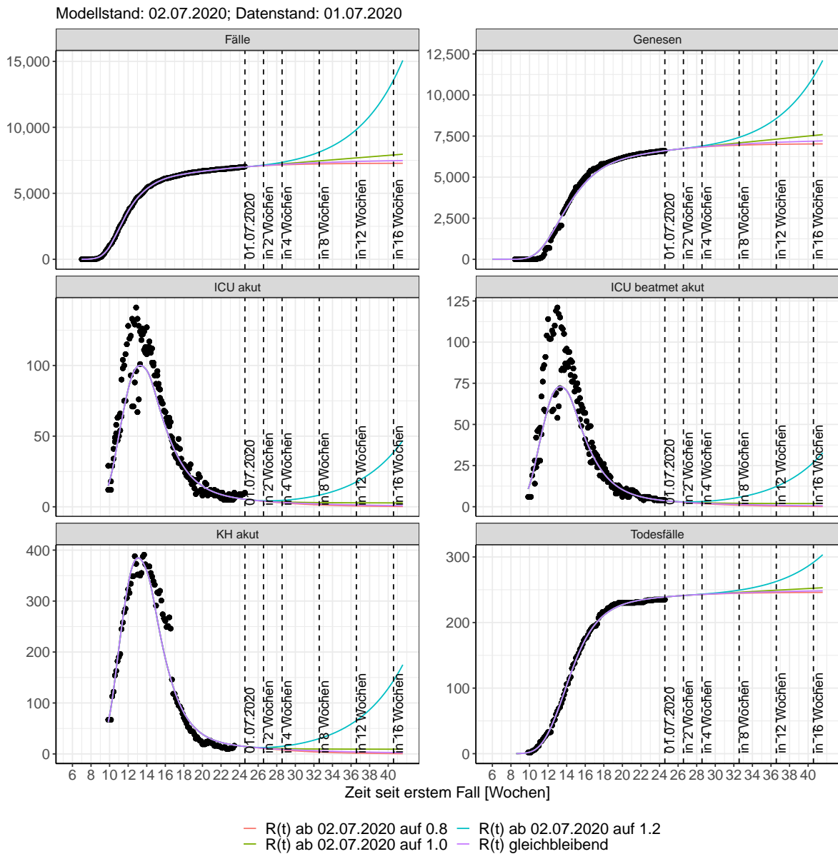
Abbildung 129: Lineare Darstellung der Modellvorhersage (Fallzahlen, Genesen, ICU Beatmet, ICU Betten, KH Betten, Todesfälle) für Rheinland-Pfalz unter Annahme verschiedener Szenarien ab dem 02.07.2020. Punkte: gemeldete Fallzahlen; Linien: Modellvorhersage.
