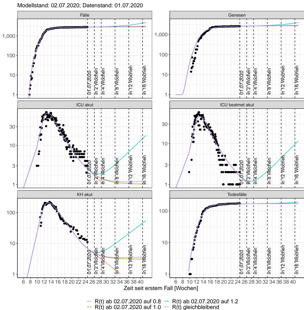
Abbildung 141: Halblogarithmische Darstellung der Modellvorhersage (Fallzahlen, Genesen, ICU Beatmet, ICU Betten, KH Betten, Todesfälle) für Saarland unter Annahme verschiedener Szenarien nach dem 02.07.2020. Punkte: gemeldete Fallzahlen; Linien: Modellvorhersage.
