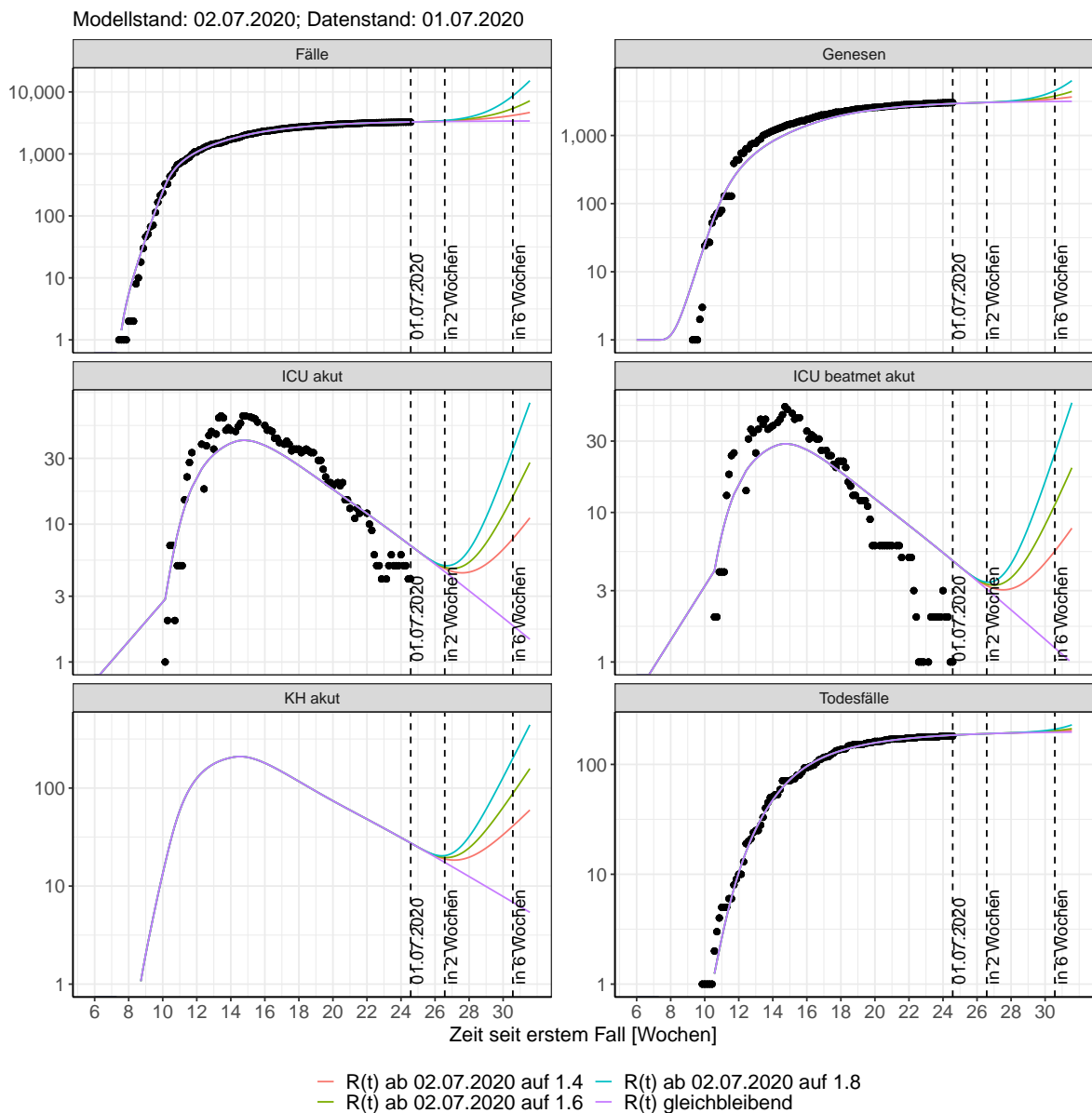
Abbildung 183: Halblogarithmische Darstellung der Modellvorhersage (Fallzahlen, Genesen, ICU Beatmet, ICU Betten, KH Betten, Todesfälle) für Thüringen unter Annahme verschiedener Szenarien nach dem 02.07.2020. Punkte: gemeldete Fallzahlen; Linien: Modellvorhersage.
