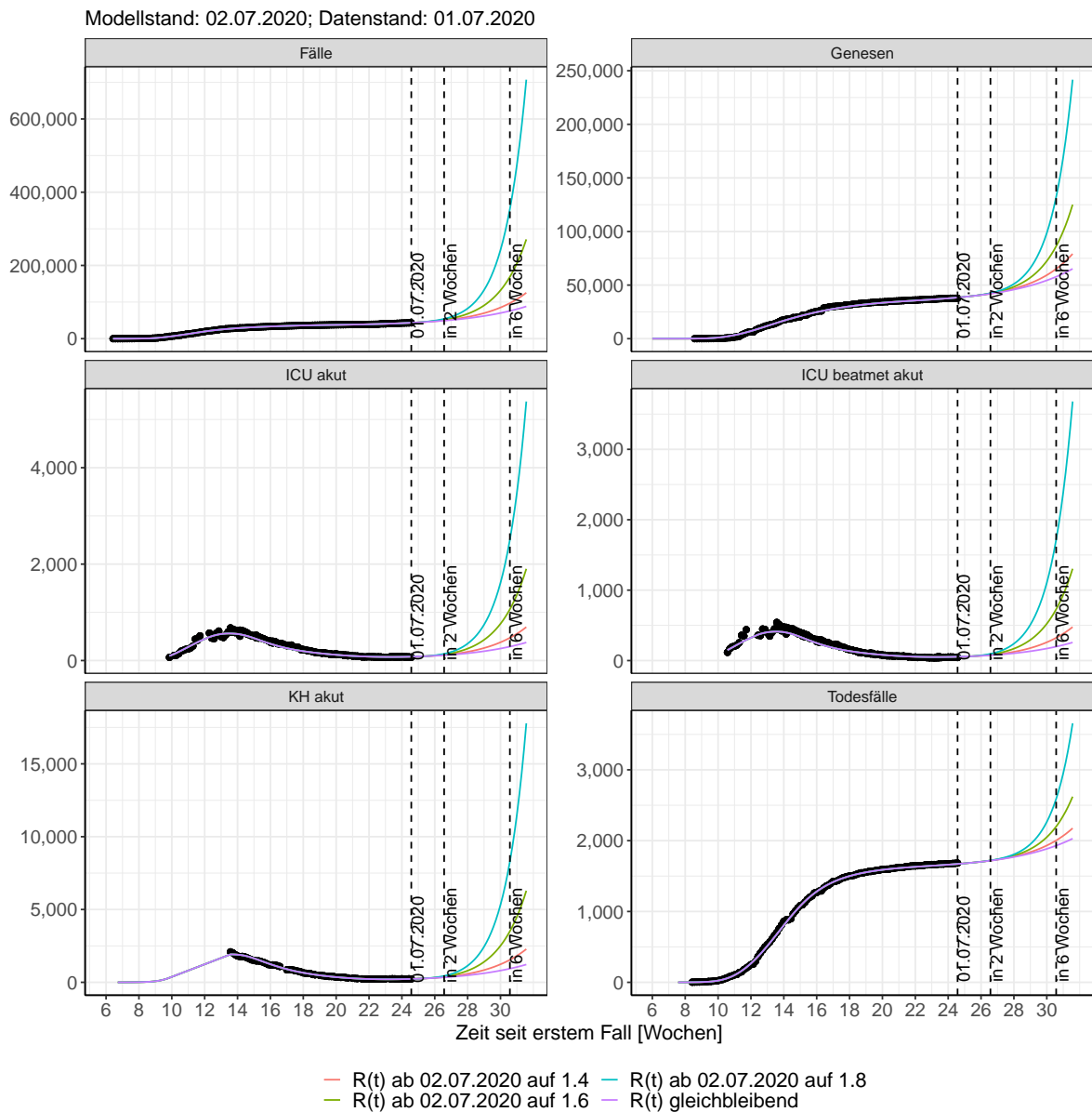
Abbildung 116: Lineare Darstellung der Modellvorhersage (Fallzahlen, Genesen, ICU Beatmet, ICU Betten, KH Betten, Todesfälle) für Nordrhein-Westfalen unter Annahme verschiedener Szenarien ab dem 02.07.2020. Punkte: gemeldete Fallzahlen; Linien: Modellvorhersage.
