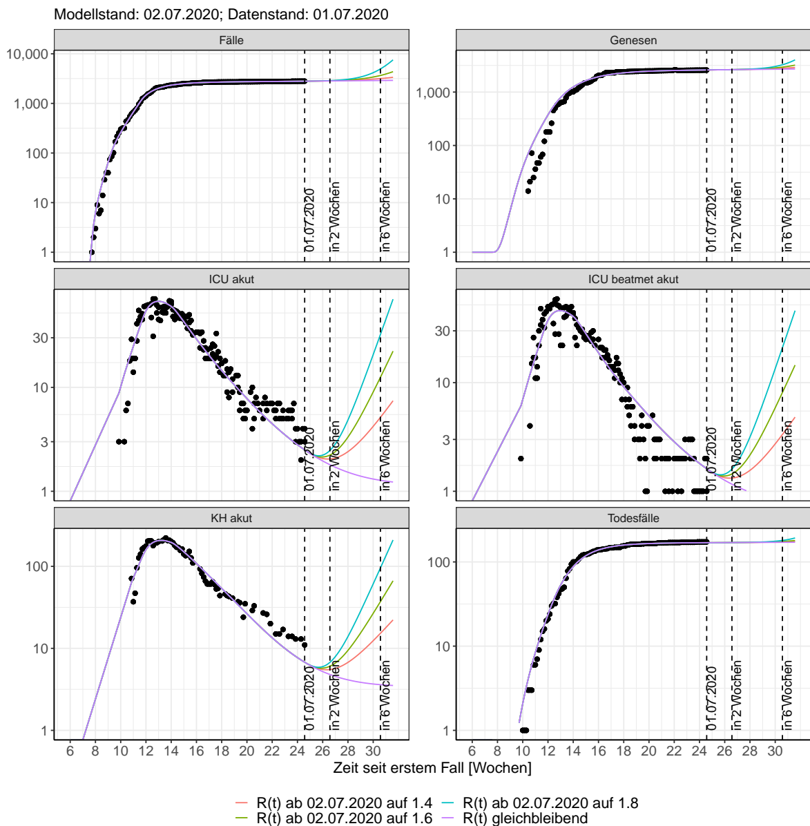
Abbildung 139: Halblogarithmische Darstellung der Modellvorhersage (Fallzahlen, Genesen, ICU Beatmet, ICU Betten, KH Betten, Todesfälle) für Saarland unter Annahme verschiedener Szenarien nach dem 02.07.2020. Punkte: gemeldete Fallzahlen; Linien: Modellvorhersage.
