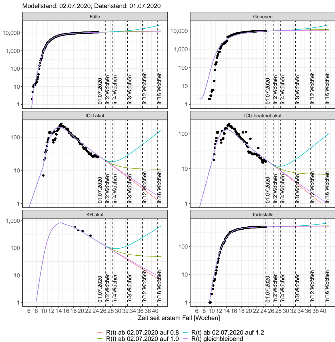
Abbildung 86: Halblogarithmische Darstellung der Modellvorhersage (Fallzahlen, Genesen, ICU Beatmet, ICU Betten, KH Betten, Todesfälle) für Hessen unter Annahme verschiedener Szenarien nach dem 02.07.2020. Punkte: gemeldete Fallzahlen; Linien: Modellvorhersage.
