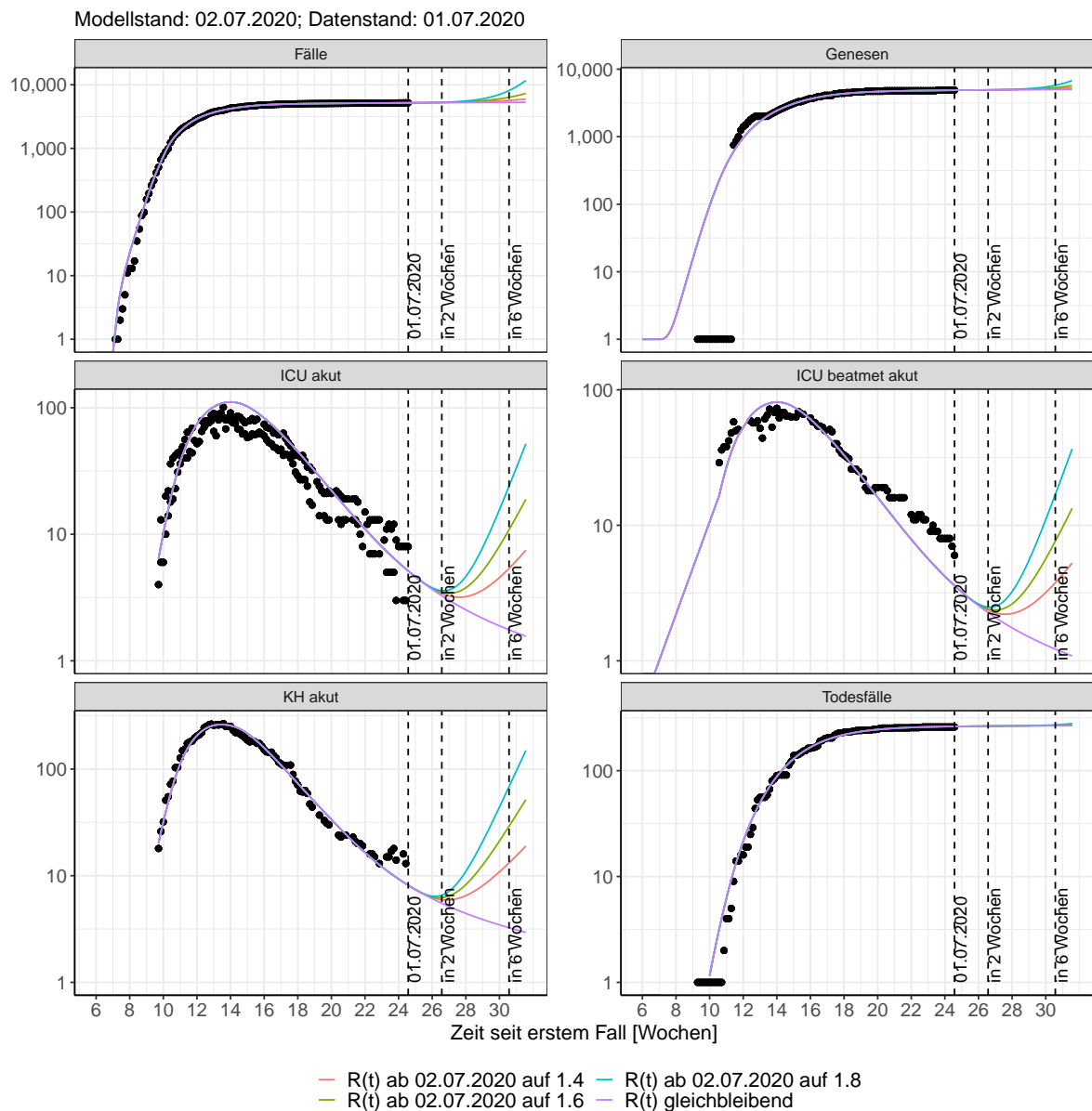
Abbildung 73: Halblogarithmische Darstellung der Modellvorhersage (Fallzahlen, Genesen, ICU Beatmet, ICU Betten, KH Betten, Todesfälle) für Hamburg unter Annahme verschiedener Szenarien nach dem 02.07.2020. Punkte: gemeldete Fallzahlen; Linien: Modellvorhersage.
