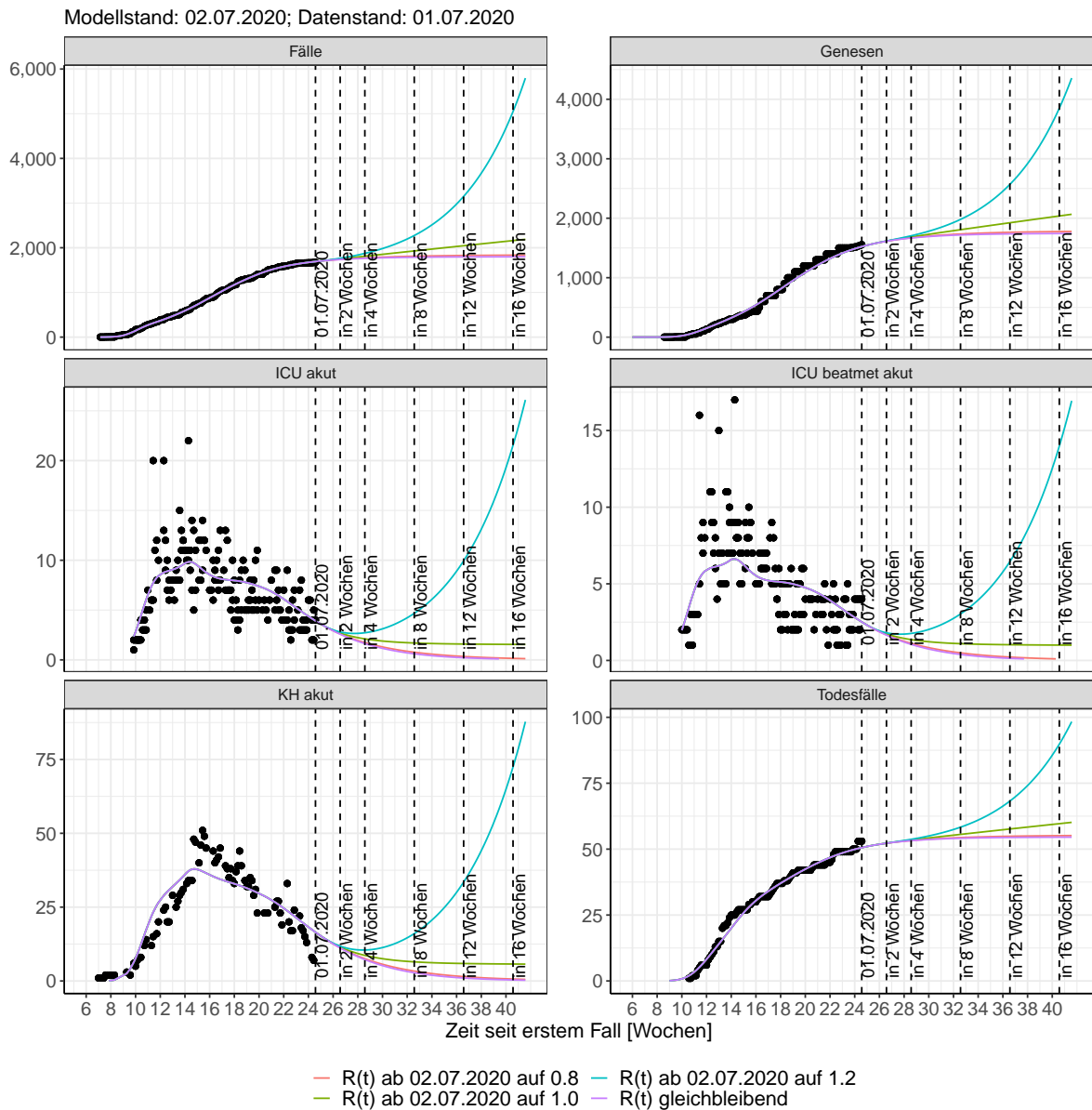
Abbildung 63: Lineare Darstellung der Modellvorhersage (Fallzahlen, Genesen, ICU Beatmet, ICU Betten, KH Betten, Todesfälle) für Bremen unter Annahme verschiedener Szenarien ab dem 02.07.2020. Punkte: gemeldete Fallzahlen; Linien: Modellvorhersage.
