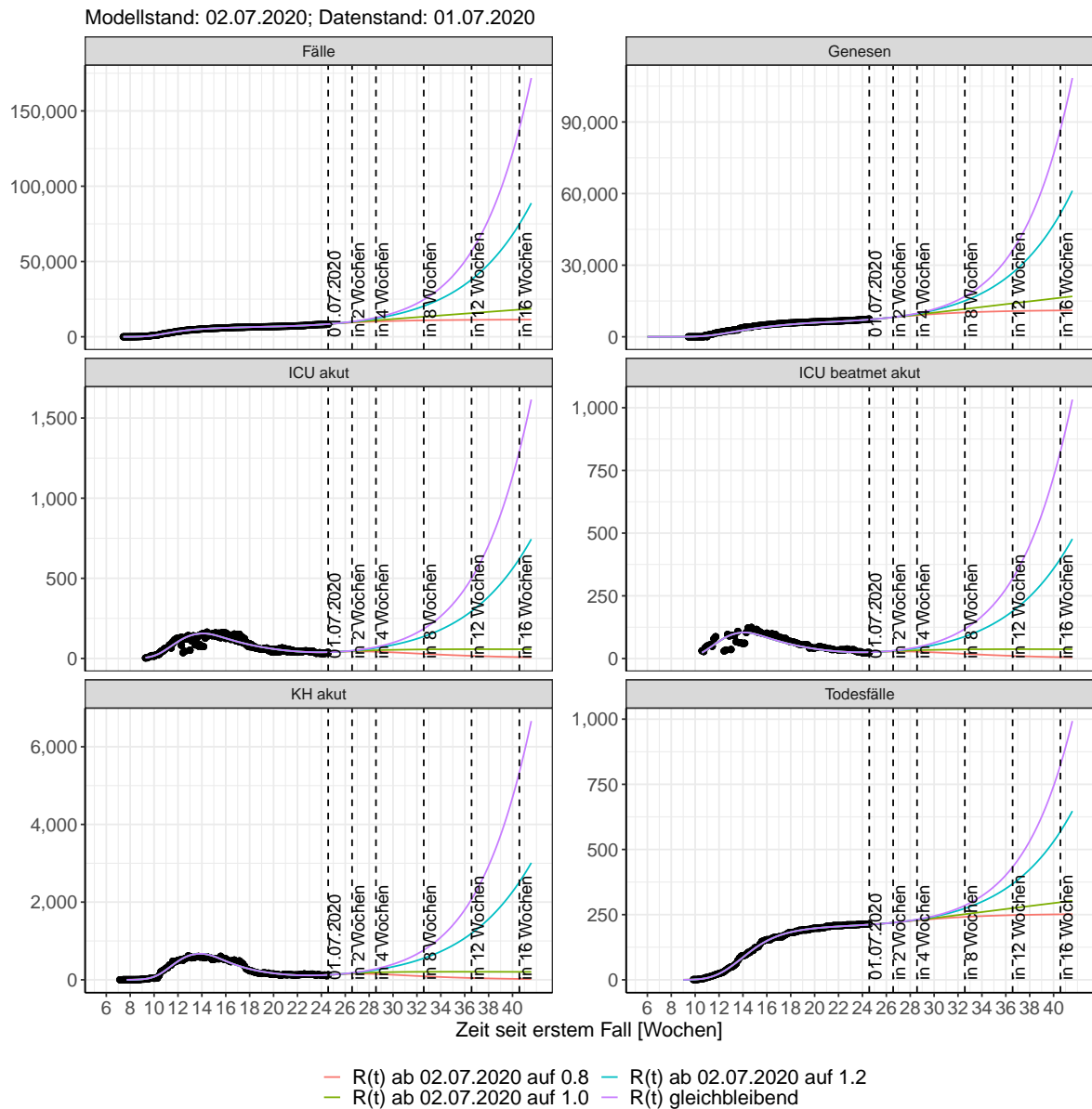
Abbildung 41: Lineare Darstellung der Modellvorhersage (Fallzahlen, Genesen, ICU Beatmet, ICU Betten, KH Betten, Todesfälle) für Berlin unter Annahme verschiedener Szenarien ab dem 02.07.2020. Punkte: gemeldete Fallzahlen; Linien: Modellvorhersage.
