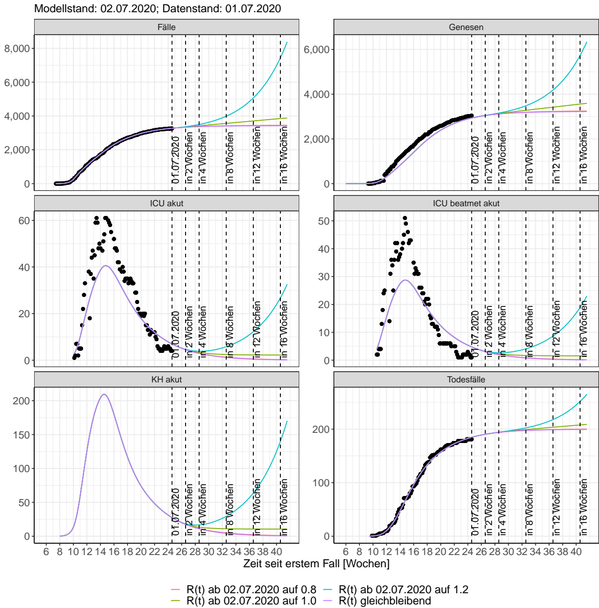
Abbildung 184: Lineare Darstellung der Modellvorhersage (Fallzahlen, Genesen, ICU Beatmet, ICU Betten, KH Betten, Todesfälle) für Thüringen unter Annahme verschiedener Szenarien ab dem 02.07.2020. Punkte: gemeldete Fallzahlen; Linien: Modellvorhersage.
