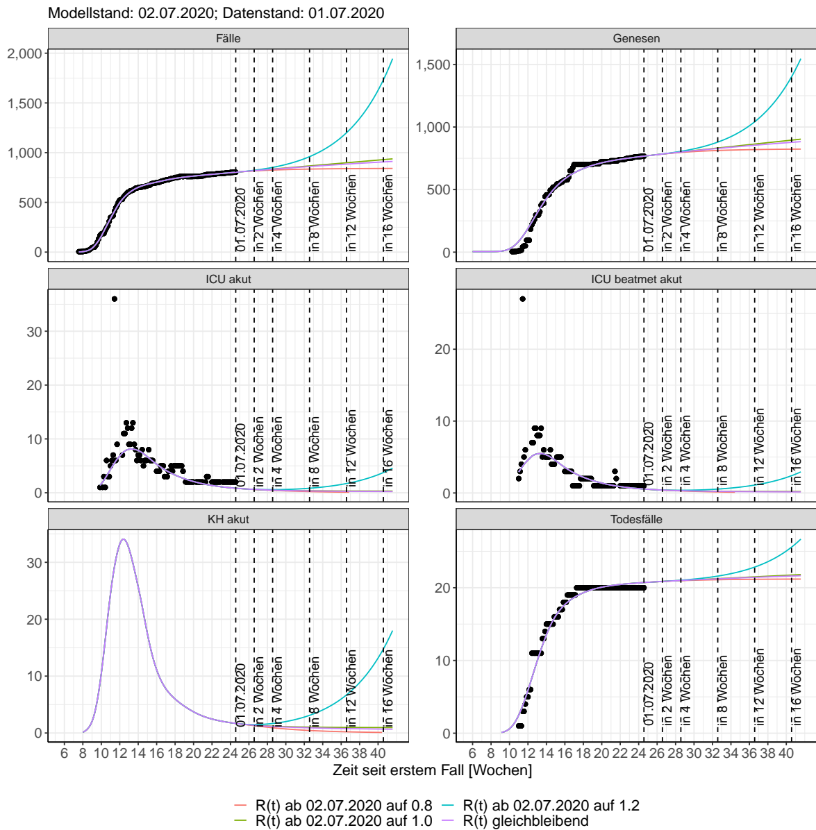
Abbildung 96: Lineare Darstellung der Modellvorhersage (Fallzahlen, Genesen, ICU Beatmet, ICU Betten, KH Betten, Todesfälle) für Mecklenburg-Vorpommern unter Annahme verschiedener Szenarien ab dem 02.07.2020. Punkte: gemeldete Fallzahlen; Linien: Modellvorhersage.
