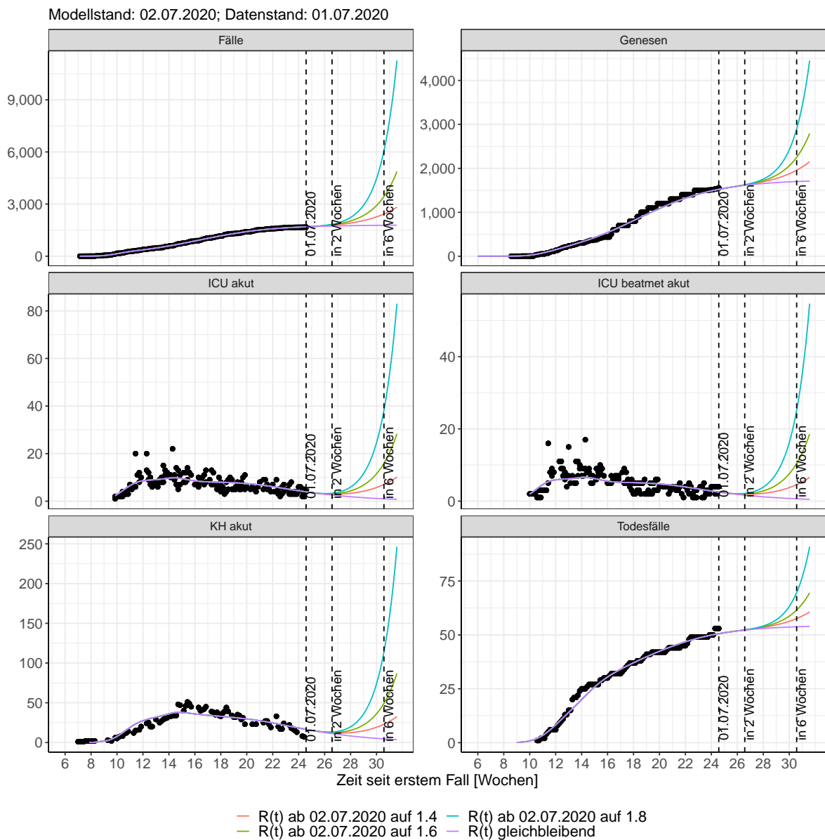
Abbildung 61: Lineare Darstellung der Modellvorhersage (Fallzahlen, Genesen, ICU Beatmet, ICU Betten, KH Betten, Todesfälle) für Bremen unter Annahme verschiedener Szenarien ab dem 02.07.2020. Punkte: gemeldete Fallzahlen; Linien: Modellvorhersage.
