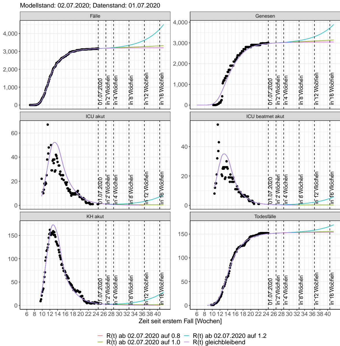
Abbildung 173: Lineare Darstellung der Modellvorhersage (Fallzahlen, Genesen, ICU Beatmet, ICU Betten, KH Betten, Todesfälle) für Schleswig-Holstein unter Annahme verschiedener Szenarien ab dem 02.07.2020. Punkte: gemeldete Fallzahlen; Linien: Modellvorhersage.
