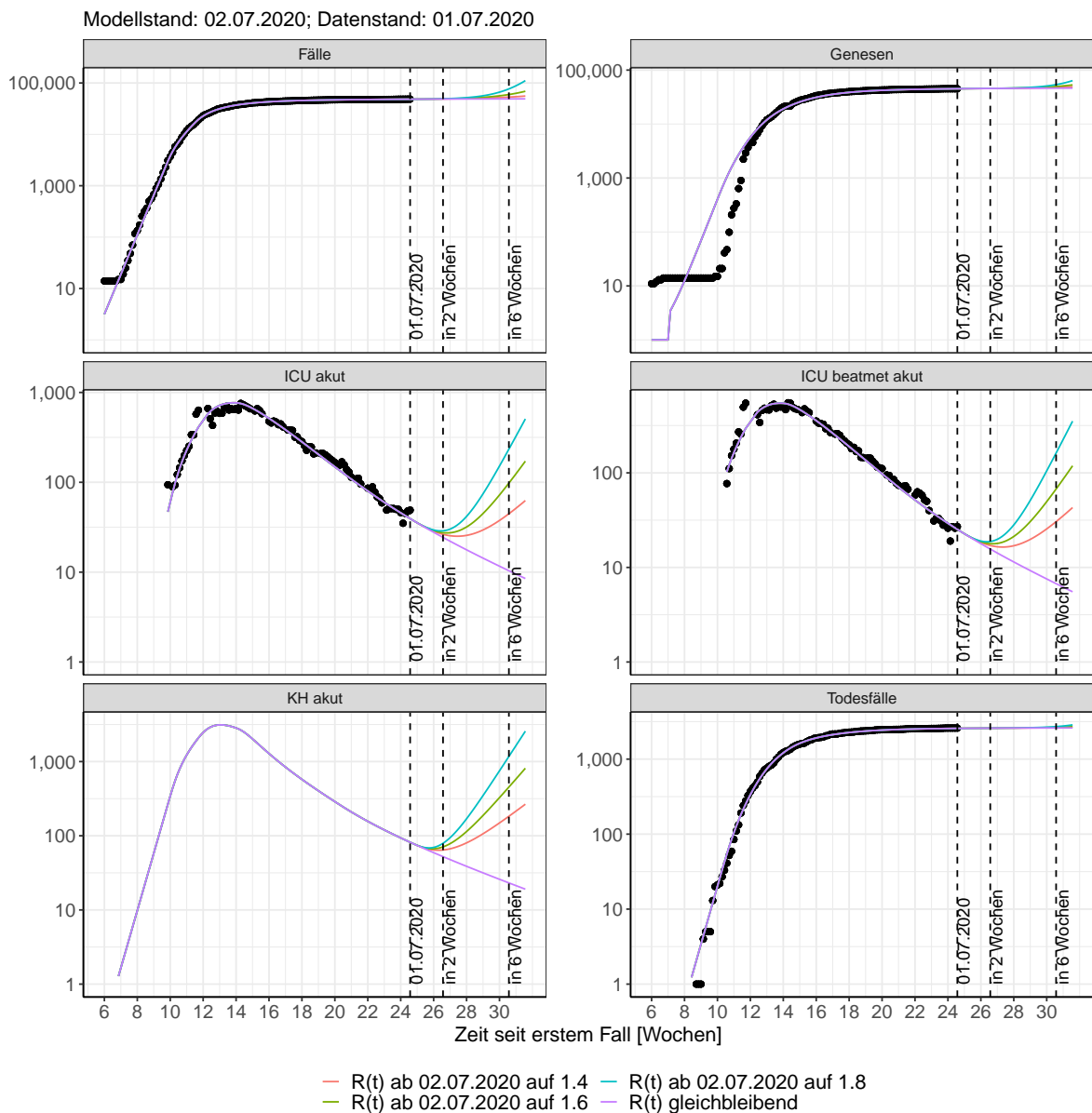
Abbildung 29: Halblogarithmische Darstellung der Modellvorhersage (Fallzahlen, Genesen, ICU Beatmet, ICU Betten, KH Betten, Todesfälle) für Bayern unter Annahme verschiedener Szenarien nach dem 02.07.2020. Punkte: gemeldete Fallzahlen; Linien: Modellvorhersage.
