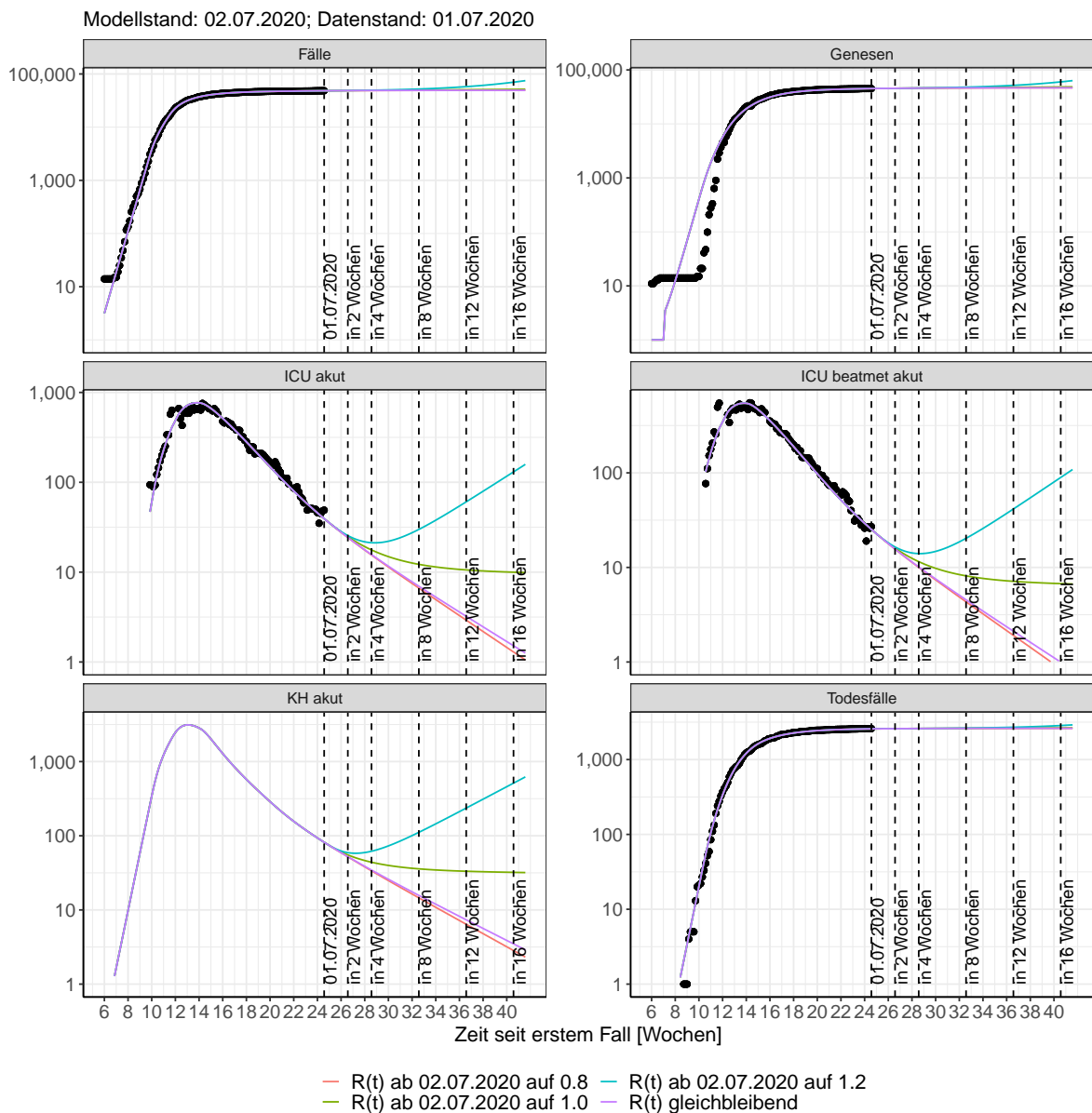
Abbildung 31: Halblogarithmische Darstellung der Modellvorhersage (Fallzahlen, Genesen, ICU Beatmet, ICU Betten, KH Betten, Todesfälle) für Bayern unter Annahme verschiedener Szenarien nach dem 02.07.2020. Punkte: gemeldete Fallzahlen; Linien: Modellvorhersage.
