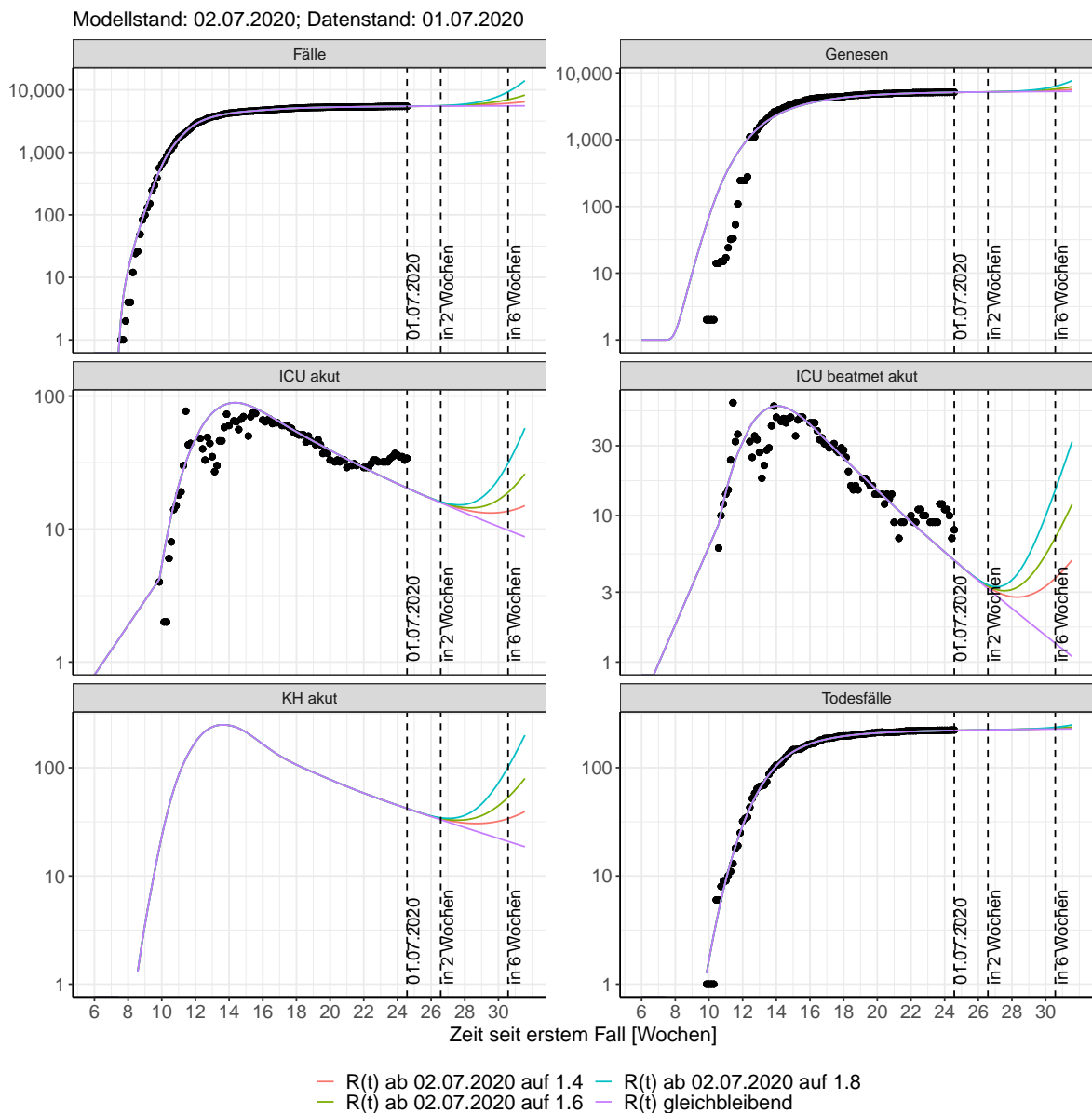
Abbildung 150: Halblogarithmische Darstellung der Modellvorhersage (Fallzahlen, Genesen, ICU Beatmet, ICU Betten, KH Betten, Todesfälle) für Sachsen unter Annahme verschiedener Szenarien nach dem 02.07.2020. Punkte: gemeldete Fallzahlen; Linien: Modellvorhersage.
