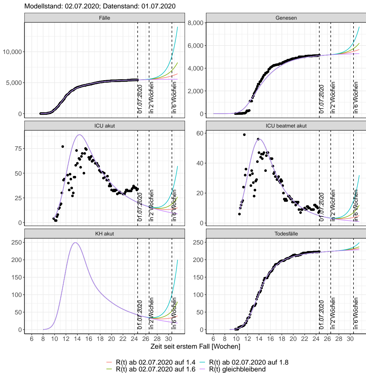
Abbildung 149: Lineare Darstellung der Modellvorhersage (Fallzahlen, Genesen, ICU Beatmet, ICU Betten, KH Betten, Todesfälle) für Sachsen unter Annahme verschiedener Szenarien ab dem 02.07.2020. Punkte: gemeldete Fallzahlen; Linien: Modellvorhersage.
