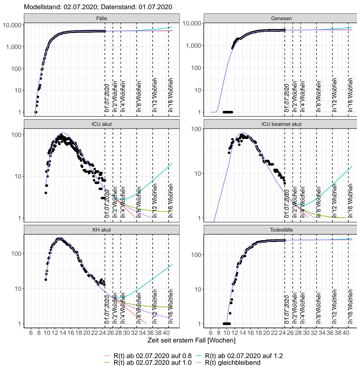
Abbildung 75: Halblogarithmische Darstellung der Modellvorhersage (Fallzahlen, Genesen, ICU Beatmet, ICU Betten, KH Betten, Todesfälle) für Hamburg unter Annahme verschiedener Szenarien nach dem 02.07.2020. Punkte: gemeldete Fallzahlen; Linien: Modellvorhersage.
