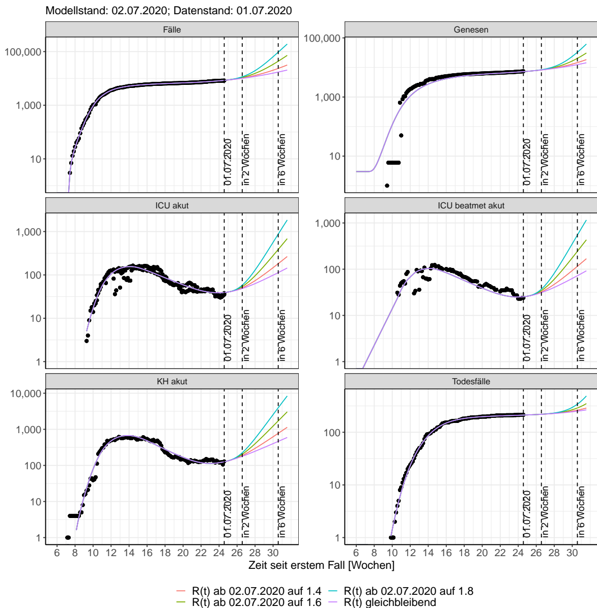
Abbildung 40: Halblogarithmische Darstellung der Modellvorhersage (Fallzahlen, Genesen, ICU Beatmet, ICU Betten, KH Betten, Todesfälle) für Berlin unter Annahme verschiedener Szenarien nach dem 02.07.2020. Punkte: gemeldete Fallzahlen; Linien: Modellvorhersage.
