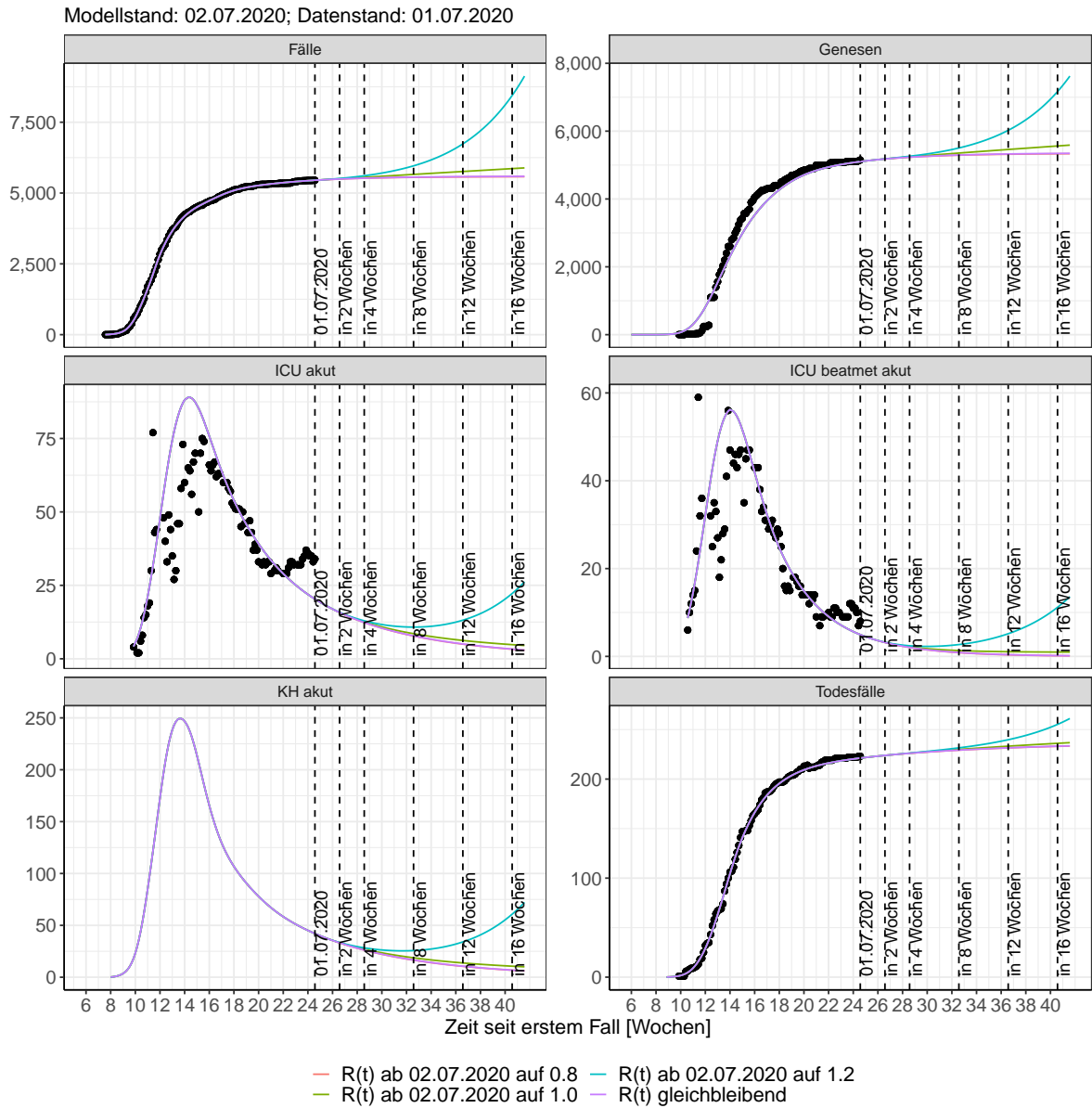
Abbildung 151: Lineare Darstellung der Modellvorhersage (Fallzahlen, Genesen, ICU Beatmet, ICU Betten, KH Betten, Todesfälle) für Sachsen unter Annahme verschiedener Szenarien ab dem 02.07.2020. Punkte: gemeldete Fallzahlen; Linien: Modellvorhersage.
