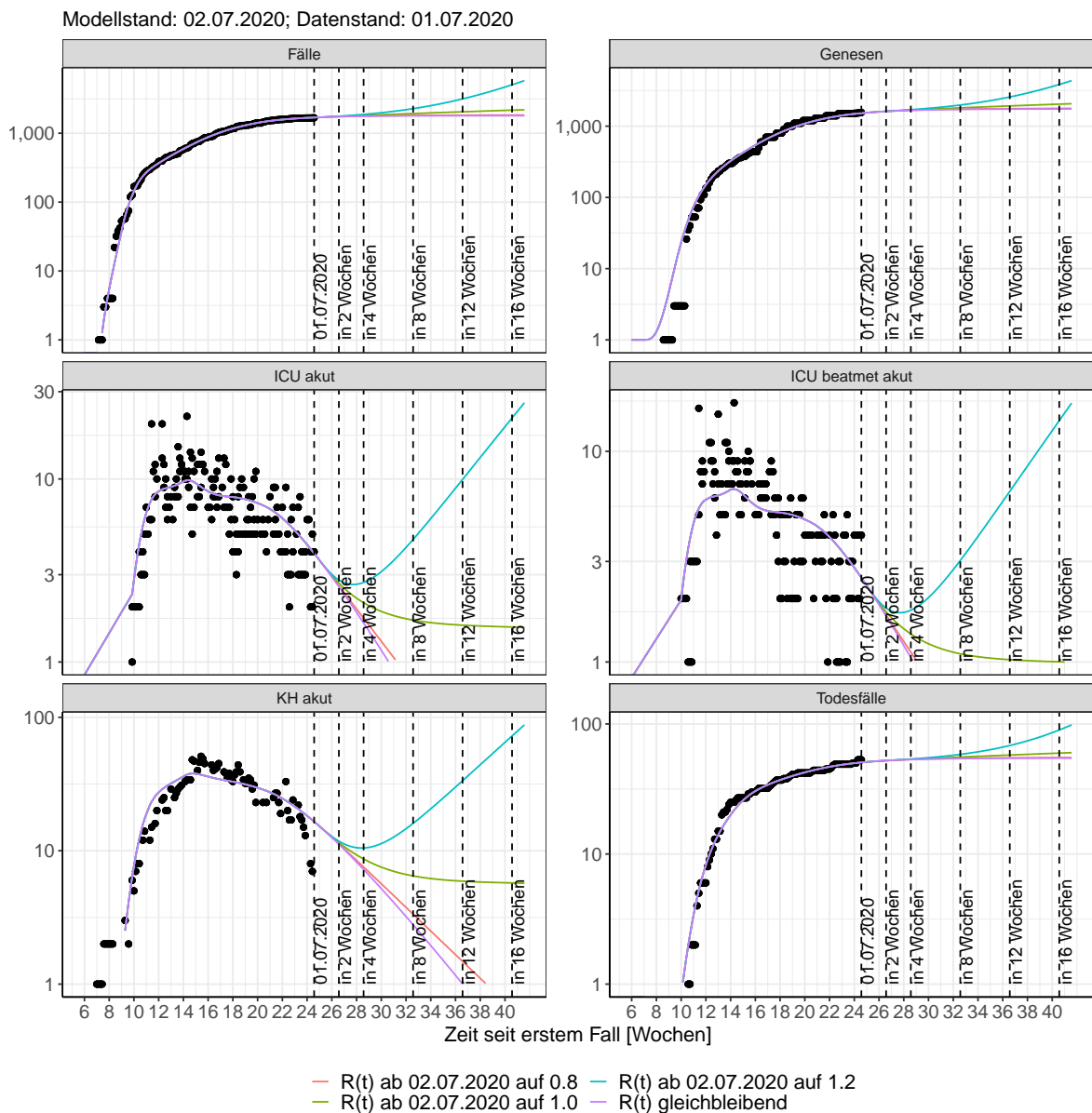
Abbildung 64: Halblogarithmische Darstellung der Modellvorhersage (Fallzahlen, Genesen, ICU Beatmet, ICU Betten, KH Betten, Todesfälle) für Bremen unter Annahme verschiedener Szenarien nach dem 02.07.2020. Punkte: gemeldete Fallzahlen; Linien: Modellvorhersage.
