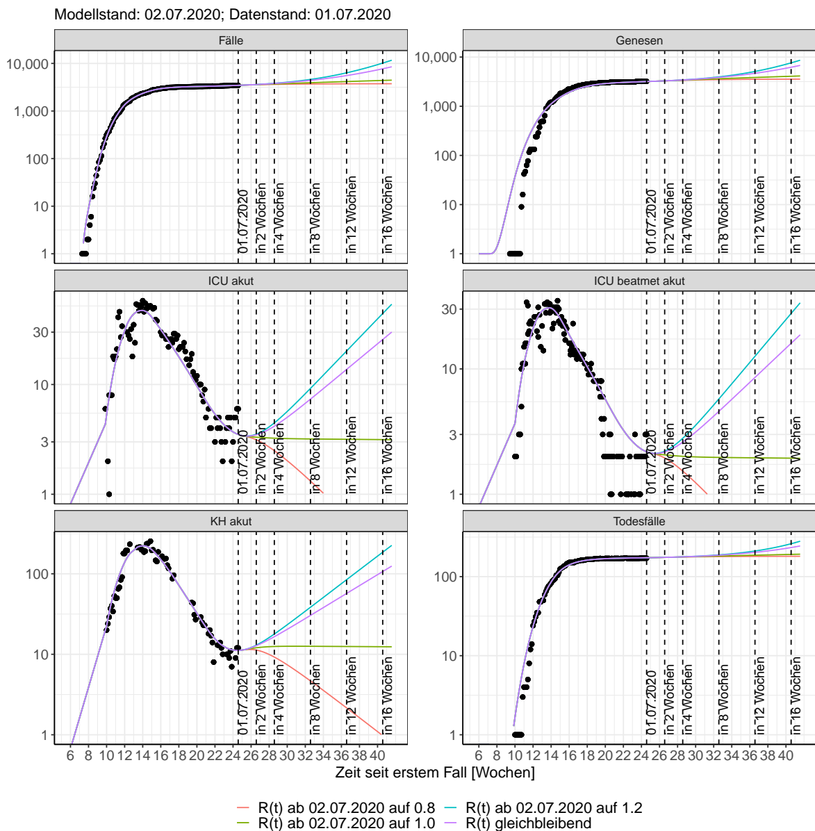
Abbildung 53: Halblogarithmische Darstellung der Modellvorhersage (Fallzahlen, Genesen, ICU Beatmet, ICU Betten, KH Betten, Todesfälle) für Brandenburg unter Annahme verschiedener Szenarien nach dem 02.07.2020. Punkte: gemeldete Fallzahlen; Linien: Modellvorhersage.
