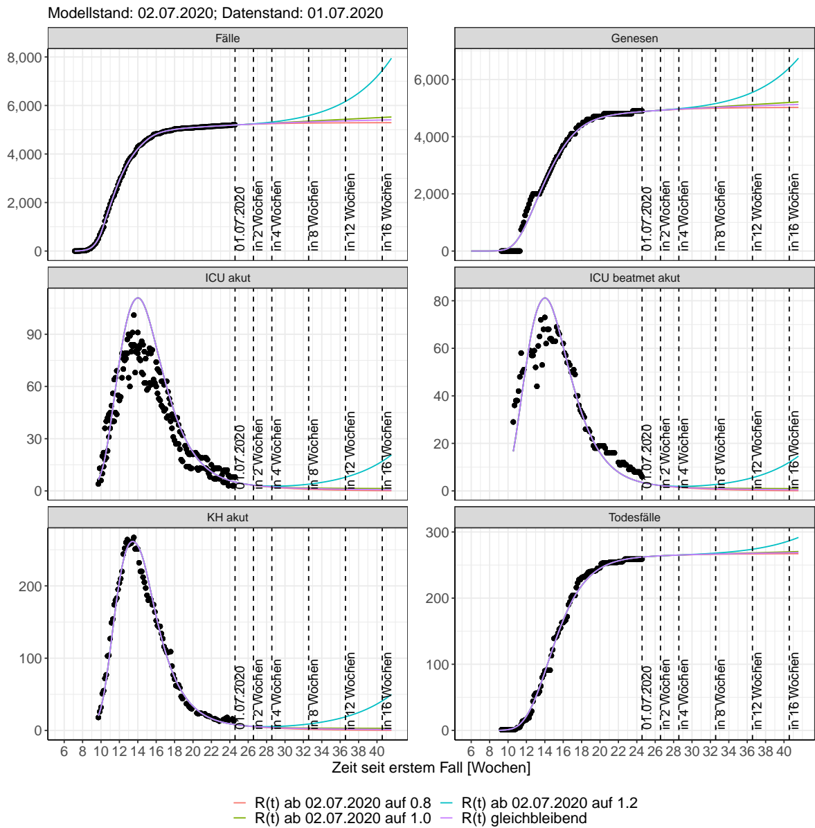
Abbildung 74: Lineare Darstellung der Modellvorhersage (Fallzahlen, Genesen, ICU Beatmet, ICU Betten, KH Betten, Todesfälle) für Hamburg unter Annahme verschiedener Szenarien ab dem 02.07.2020. Punkte: gemeldete Fallzahlen; Linien: Modellvorhersage.
