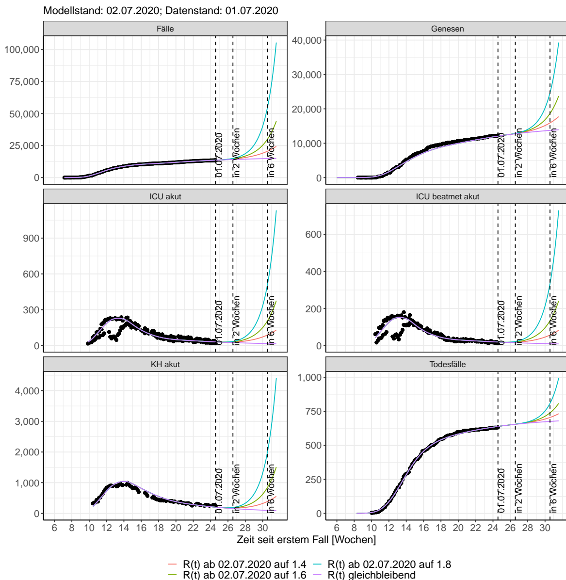
Abbildung 105: Lineare Darstellung der Modellvorhersage (Fallzahlen, Genesen, ICU Beatmet, ICU Betten, KH Betten, Todesfälle) für Niedersachsen unter Annahme verschiedener Szenarien ab dem 02.07.2020. Punkte: gemeldete Fallzahlen; Linien: Modellvorhersage.
