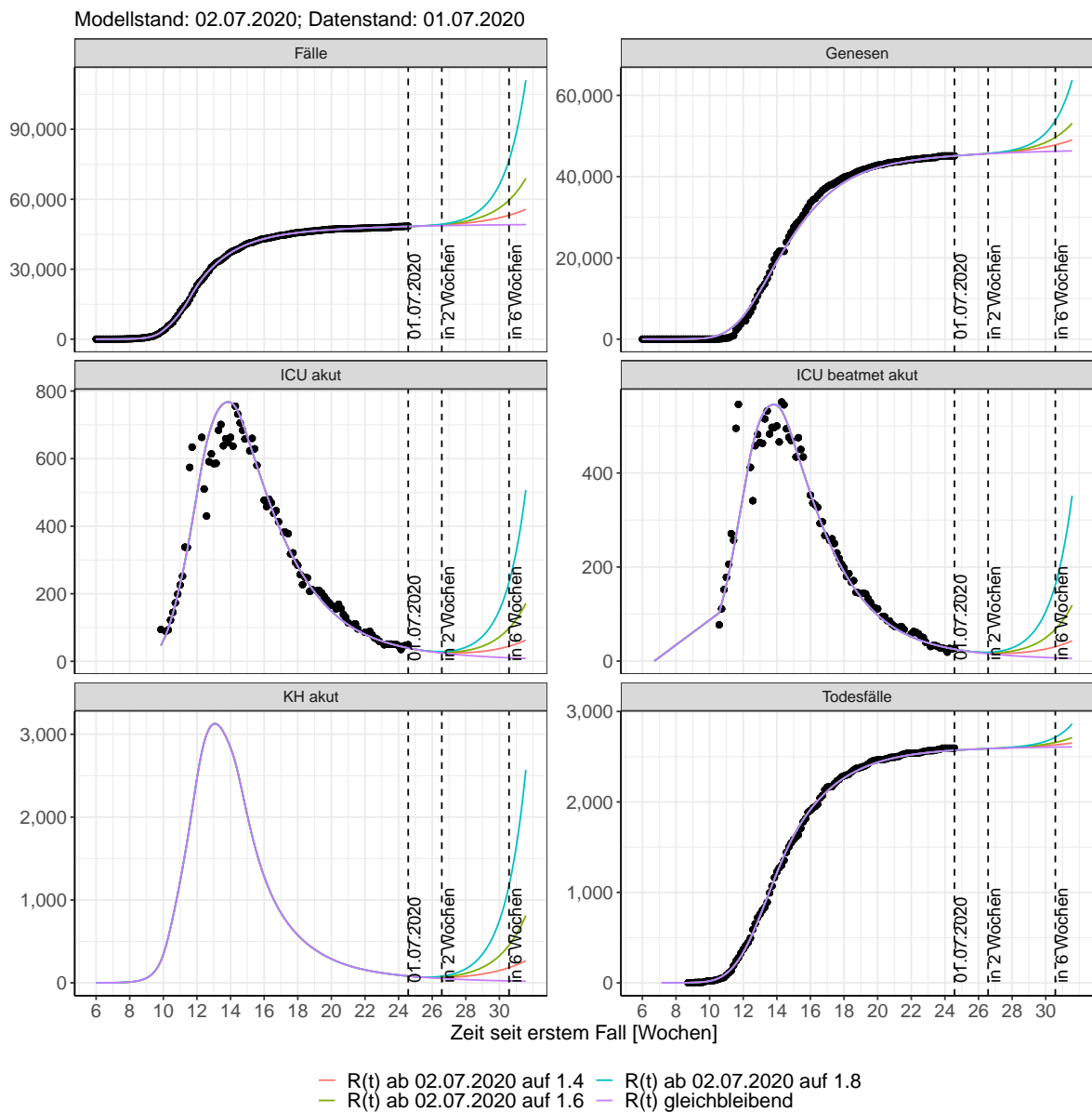
Abbildung 28: Lineare Darstellung der Modellvorhersage (Fallzahlen, Genesen, ICU Beatmet, ICU Betten, KH Betten, Todesfälle) für Bayern unter Annahme verschiedener Szenarien ab dem 02.07.2020. Punkte: gemeldete Fallzahlen; Linien: Modellvorhersage.
