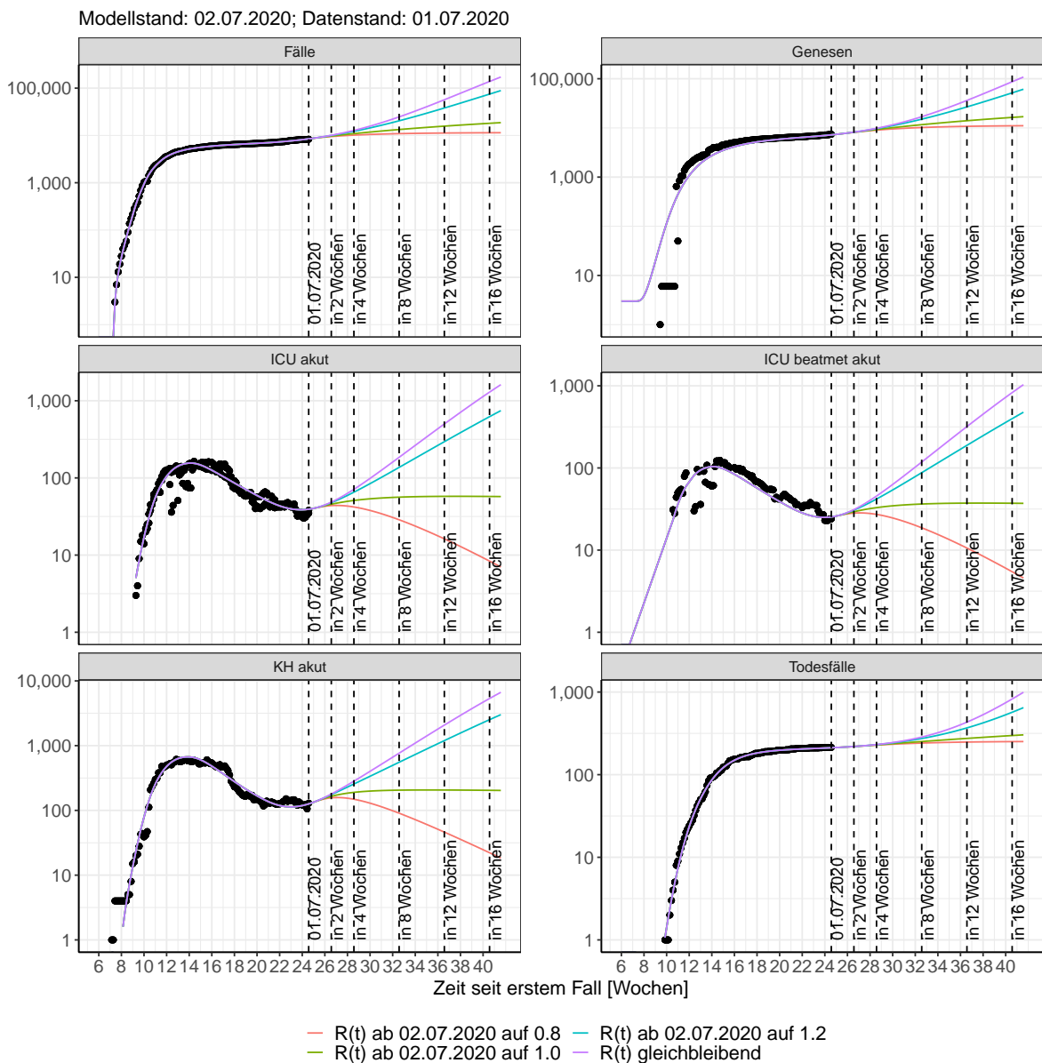
Abbildung 42: Halblogarithmische Darstellung der Modellvorhersage (Fallzahlen, Genesen, ICU Beatmet, ICU Betten, KH Betten, Todesfälle) für Berlin unter Annahme verschiedener Szenarien nach dem 02.07.2020. Punkte: gemeldete Fallzahlen; Linien: Modellvorhersage.
