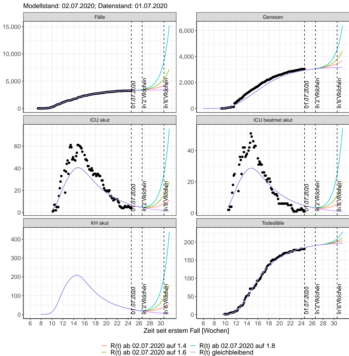
Abbildung 182: Lineare Darstellung der Modellvorhersage (Fallzahlen, Genesen, ICU Beatmet, ICU Betten, KH Betten, Todesfälle) für Thüringen unter Annahme verschiedener Szenarien ab dem 02.07.2020. Punkte: gemeldete Fallzahlen; Linien: Modellvorhersage.
