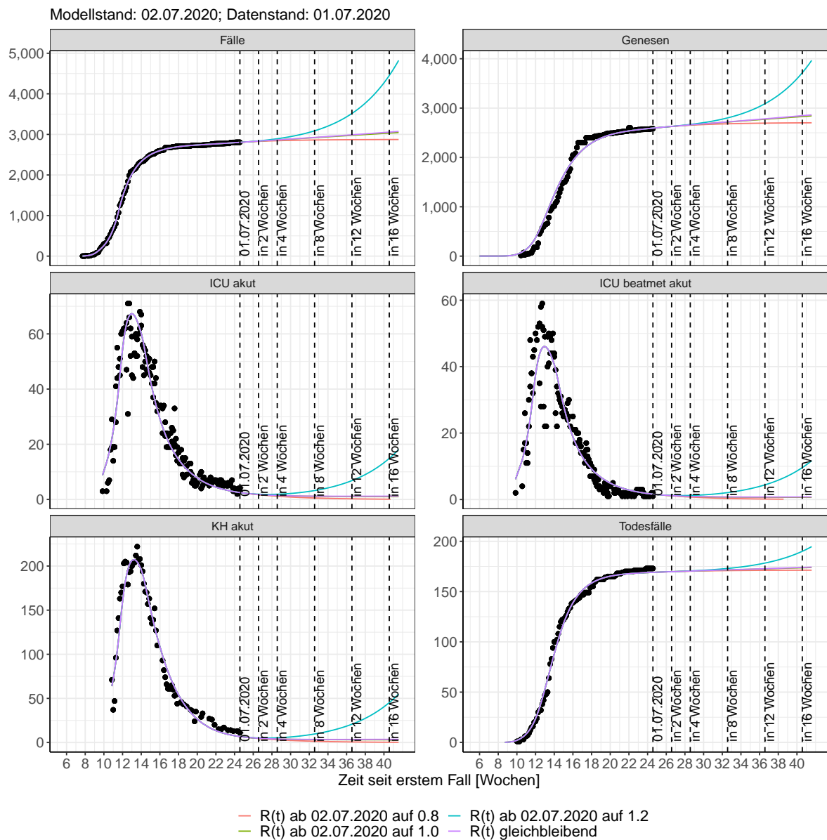
Abbildung 140: Lineare Darstellung der Modellvorhersage (Fallzahlen, Genesen, ICU Beatmet, ICU Betten, KH Betten, Todesfälle) für Saarland unter Annahme verschiedener Szenarien ab dem 02.07.2020. Punkte: gemeldete Fallzahlen; Linien: Modellvorhersage.
